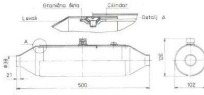
Слика 1а – нутрашња права и кондензаторска спојница
