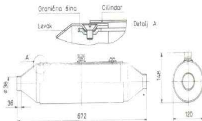
Слика 1б – Унутрашња пупинована спојница
