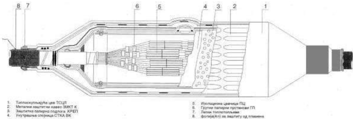
Слика 2 - Спојница за пружне телекомуникационе каблове
