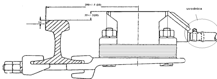
Nosač balize
