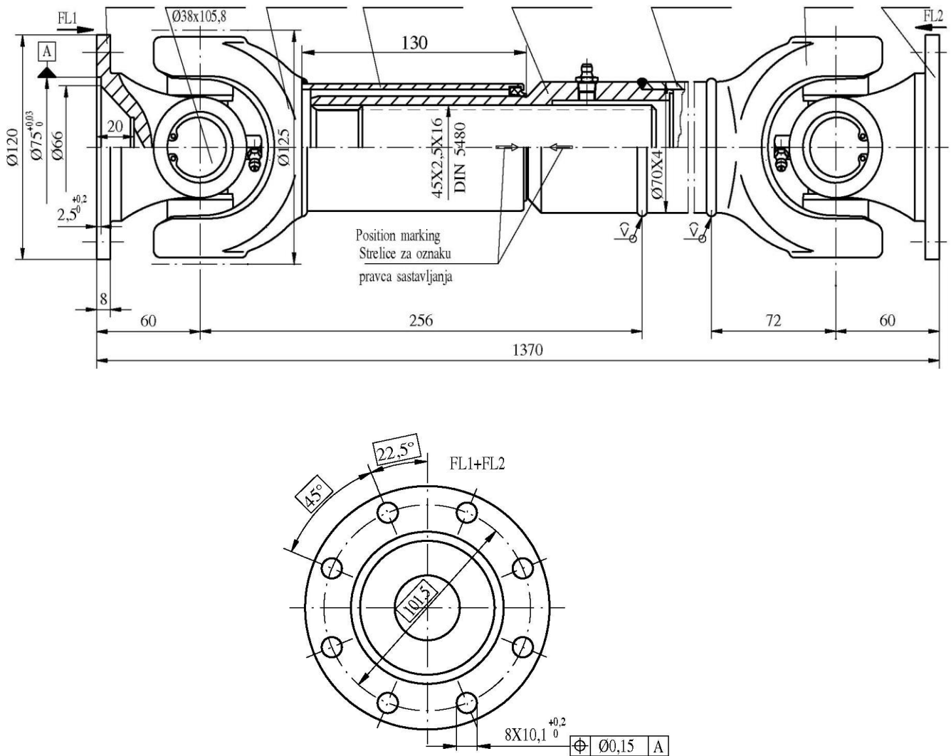
Слика 3: Карданско вратило В120.01.1370
