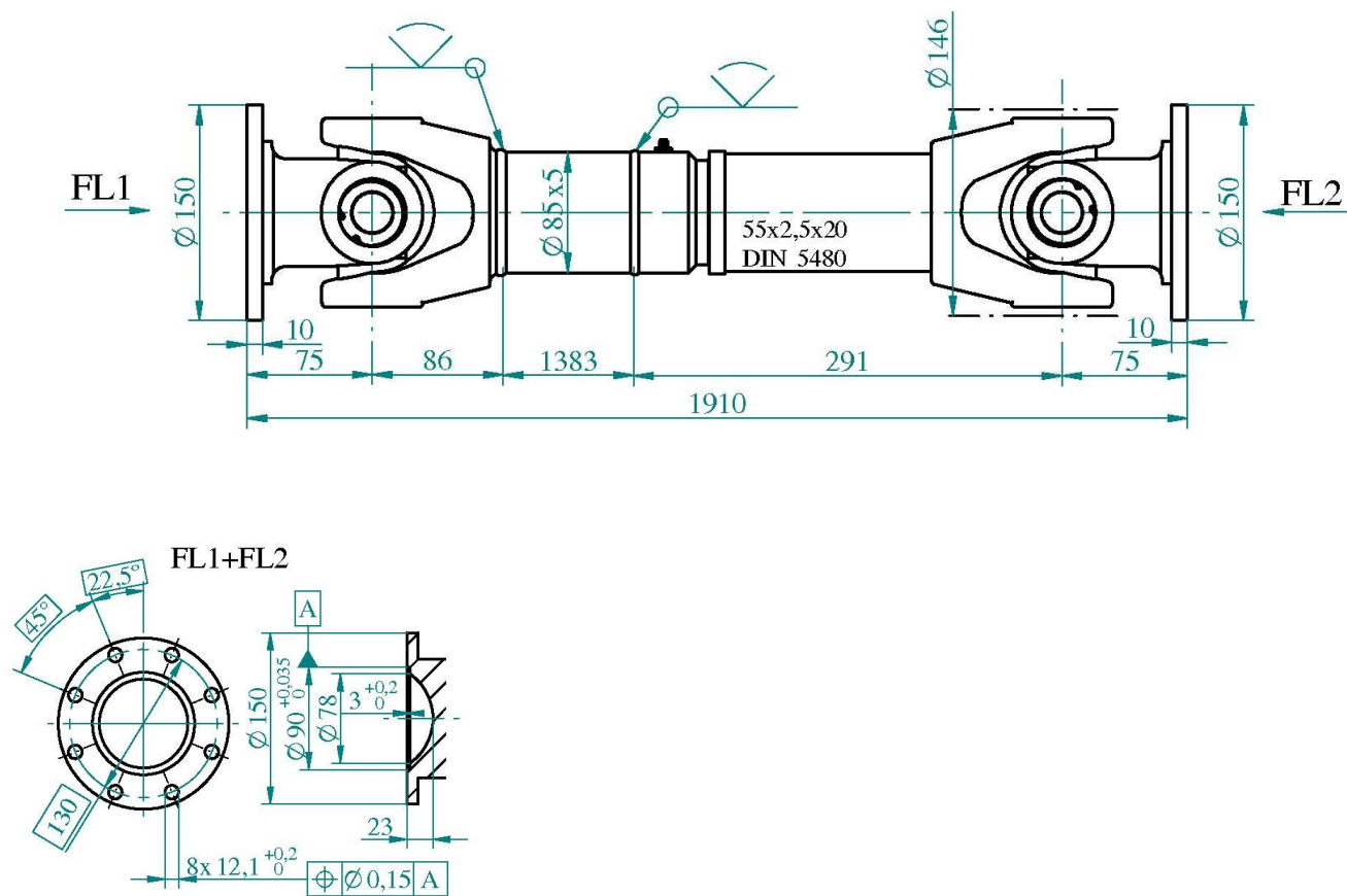
Слика 2: Карданско вратило B150.01.1910
