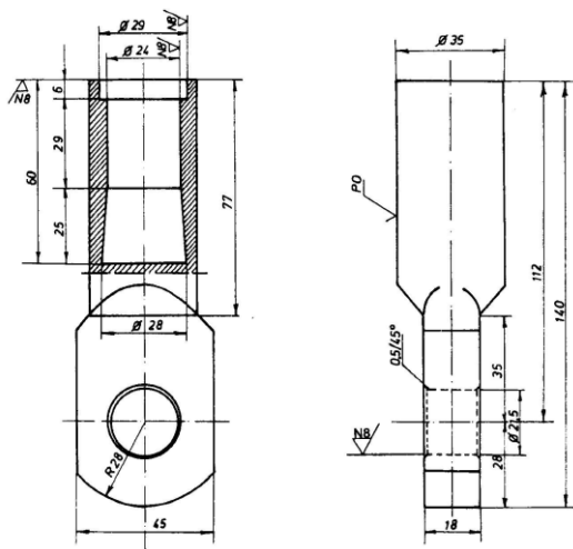
Слика 2. Капа изолатор каталошки број 350502
