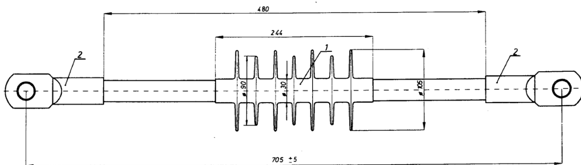
Слика 1. Затезни изолатор каталошки број 350500
