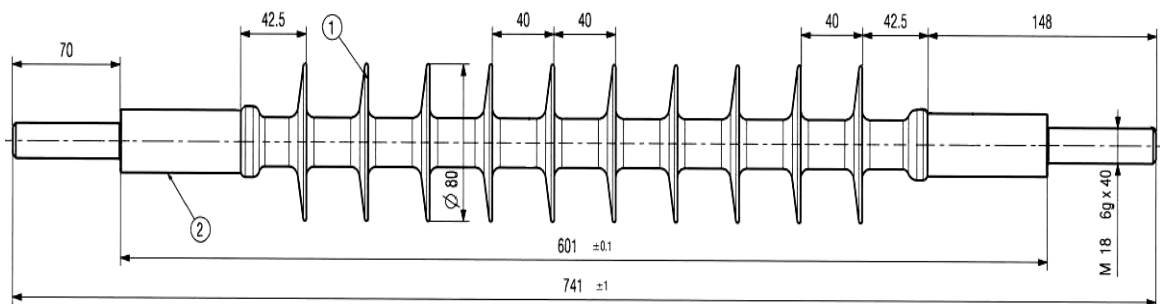
Слика 4. 400100g горњи изолатор
