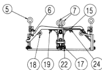
Слика 2. Склоп секционог изолатор SAE 400100
