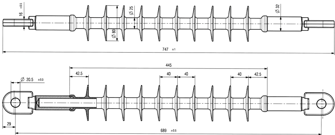
Слика 3. 400100d доњи изолатор
