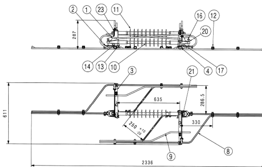
Слика 1. Склоп секционог изолатор SAE 400100
