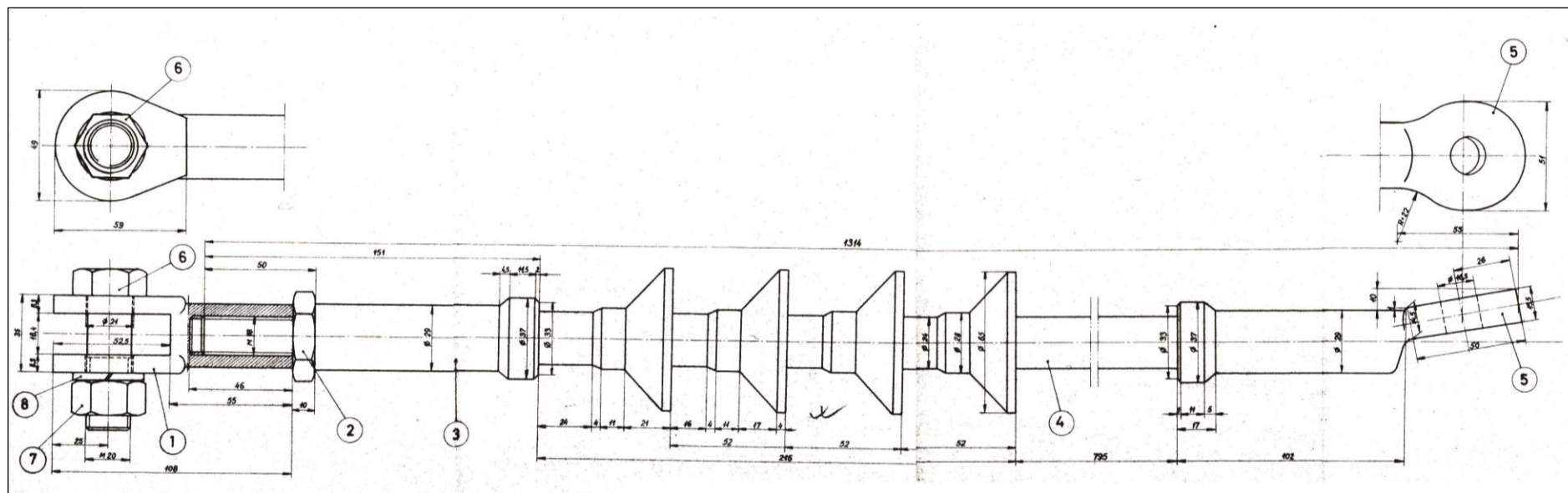
Цртеж број 2 - изолаторску затега права у чврстој тачки каталошки број 305100
