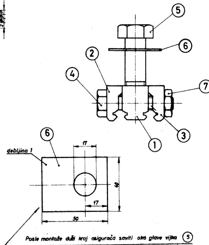
Цртеж број 3 – стезалку двоструког контактнoг проводника у чврстој тачки каталошки број 305000
