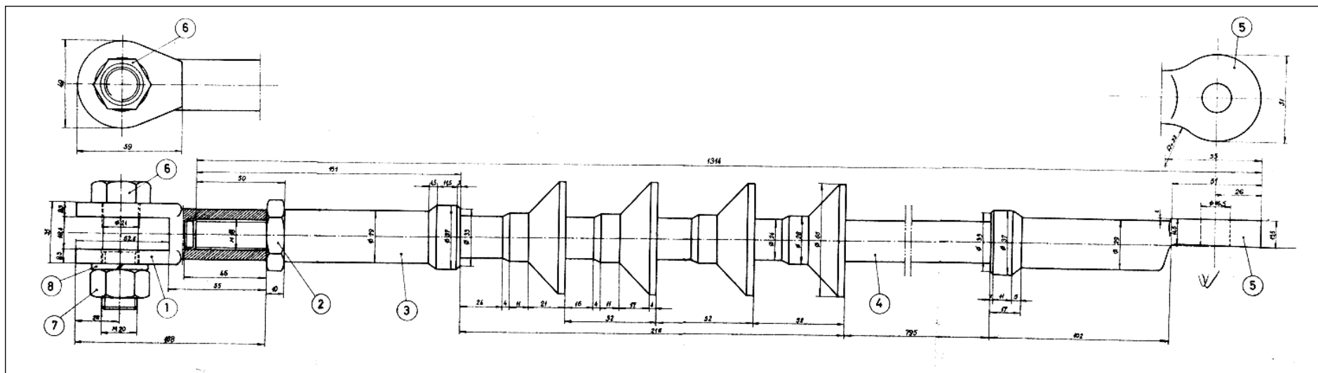
Цртеж број 1 - изолаторску затега права у чврстој тачки каталошки број 305200
