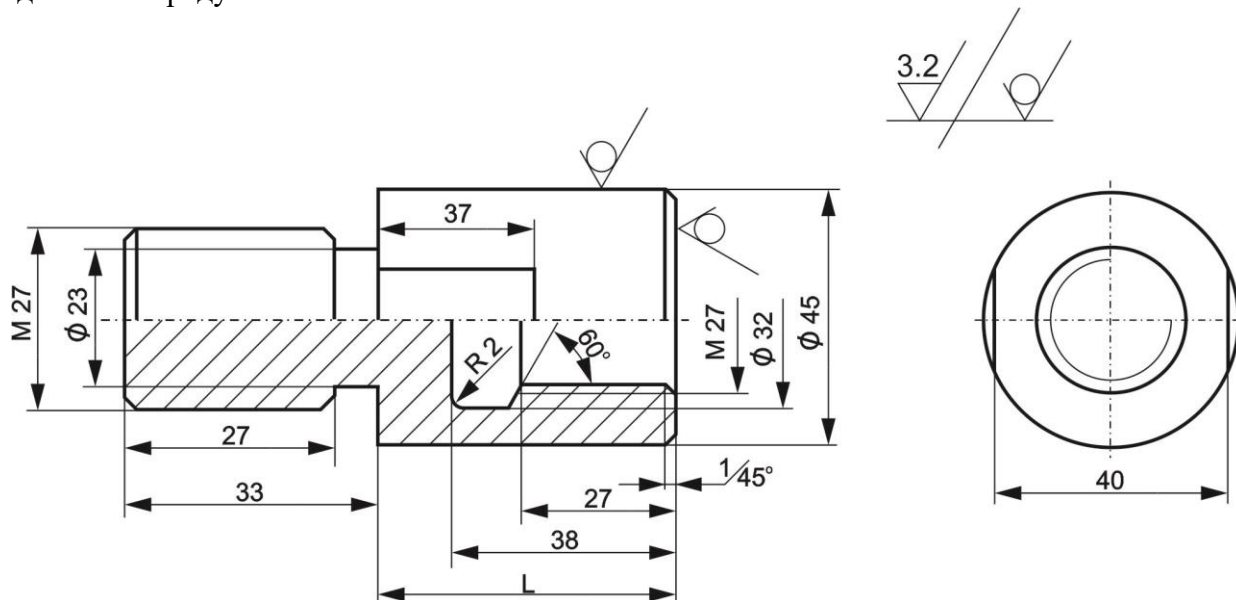
Цртеж број 4. Наставак за причвршћење опреме за вешање у тунелу TR1 – 73
