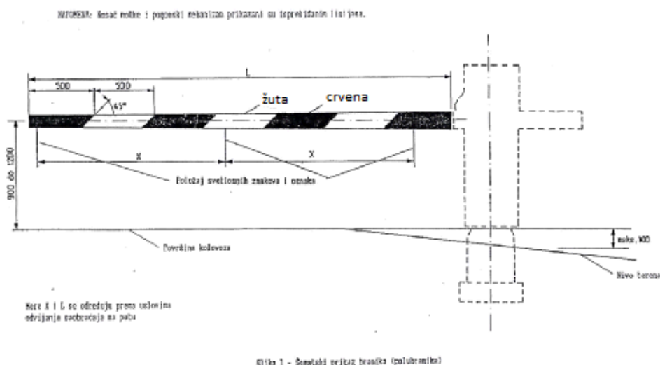
Слика 1 - Шематски приказ баника (полубаника)
