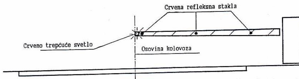
Слика 3. Распоред светлосних знакова на мотки браника ( полубраника) типа L=3,5м и L= 4.5м
