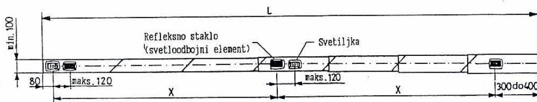
Слика 2. Распоред светлосних знакова на мотки браника ( полубраника) типа L=7,5\text{м}
