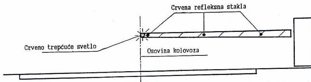
Слика 3. Распоред светлосних знакова на мотки браника ( полубраника) типа L=3,5\text{м} и L=4,5\text{м}
