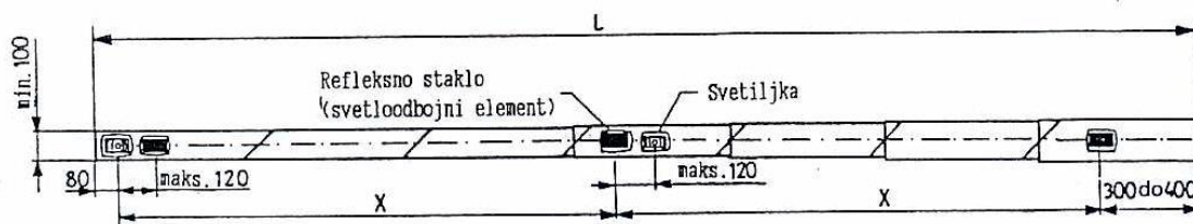
Слика 2. Распоред светлосних знакова на мотки браника ( полубраника) типа L=7,5м
