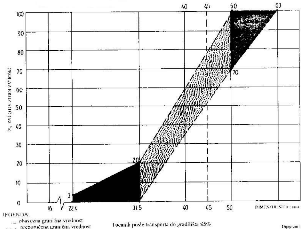
Дијаграм гранулометријског састава туцаника 31,5 / 63 mm
