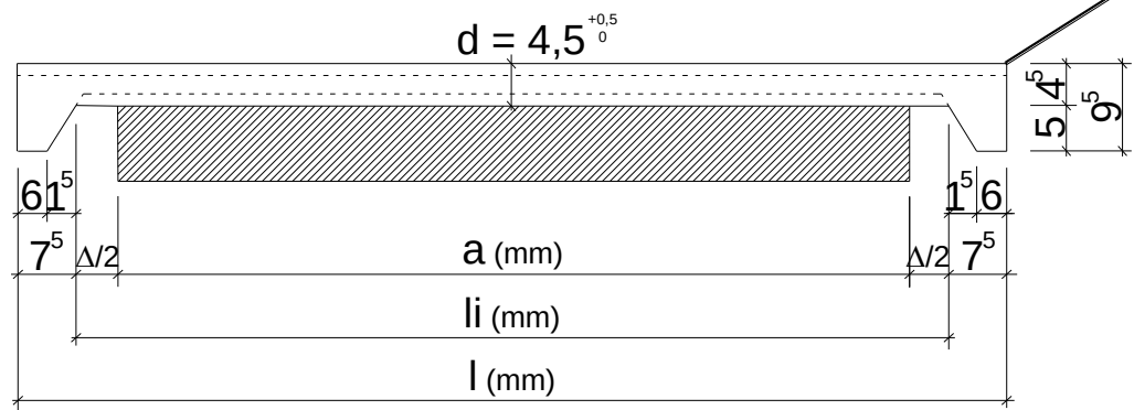
ТАБЕЛА: Димензије гумене подлошке за шину 49Е1
