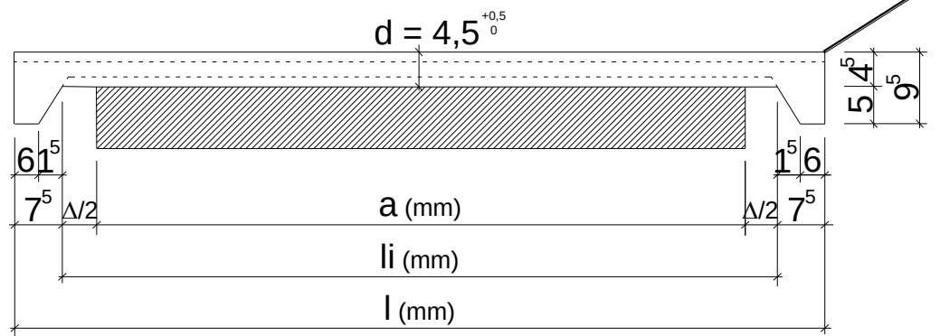
ТАБЕЛА: Димензије гумене подлошке за шину 49Е1
