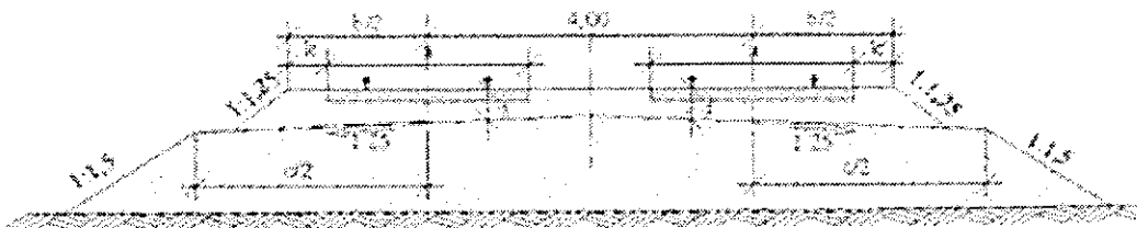
Слика 5. Попречни пресек застора призме код двоколосечне и паралелне пруге у правцу
