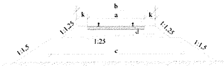
Слика 3. Попречни пресек засторне призме на једноколосечној прузи у правцу код једностраног нагиба планума после машинског решетања застора.
