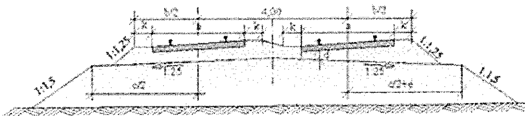
Слика 6. Попречни пресек засторне призме код двоколосечних пруга, у кривини
