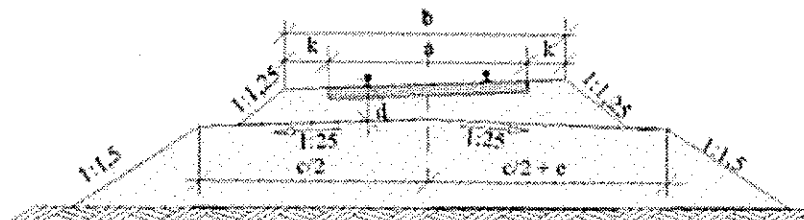
Слика 2. Попречни пресек засторне призме на једноколосечној прузи у кривини код двостраног нагиба пленума.
