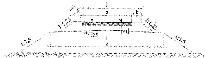
Слика 1. Попречни пресек засторне призме на једноколосечној прузи у правцу код двостраног нагиба пленума.
