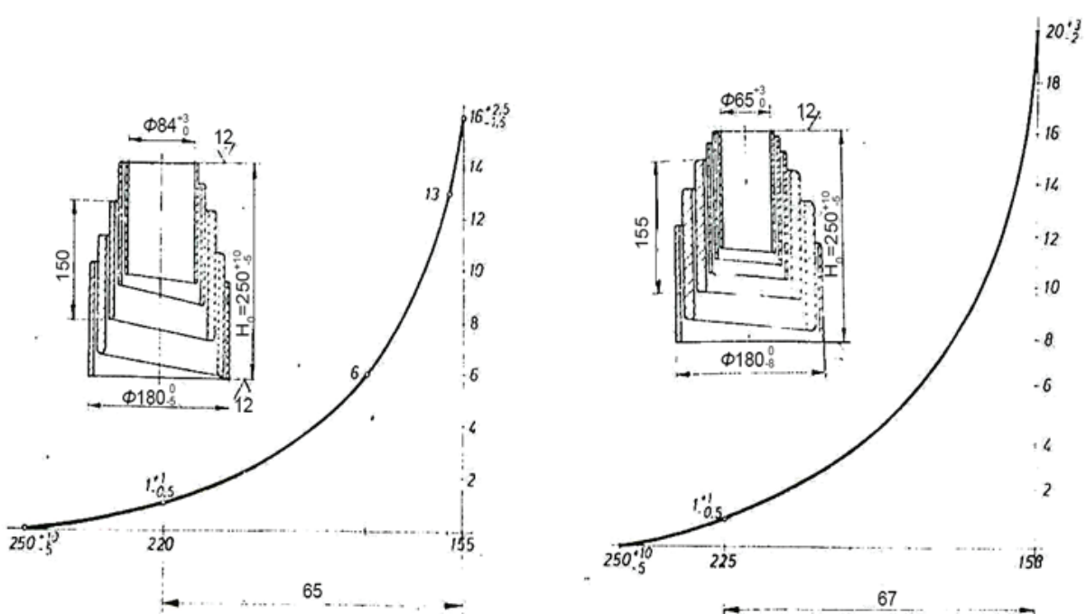
Сл.1. Опруга за тегљенике продужног типа код кола
