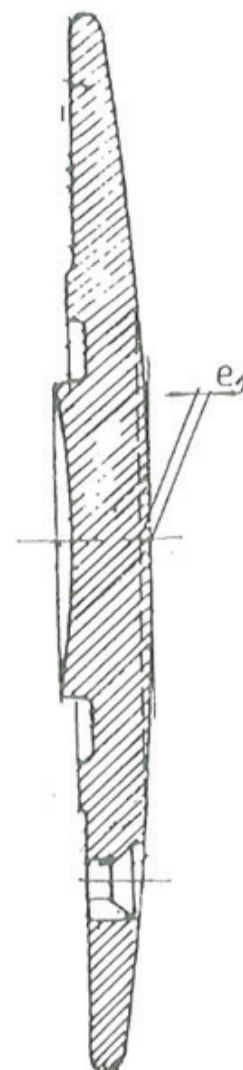
Сл 3. Одбојничка плоча одбојника 590 kN, 105mm, минер 30 kJ
