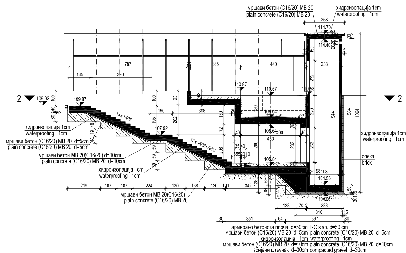
ПОПРЕЧНИ ПРЕСЕК 5-5 КРОЗ ПОТХОДНИК CROSS SECTION 5-5 THROUGH THE SUBWAY
