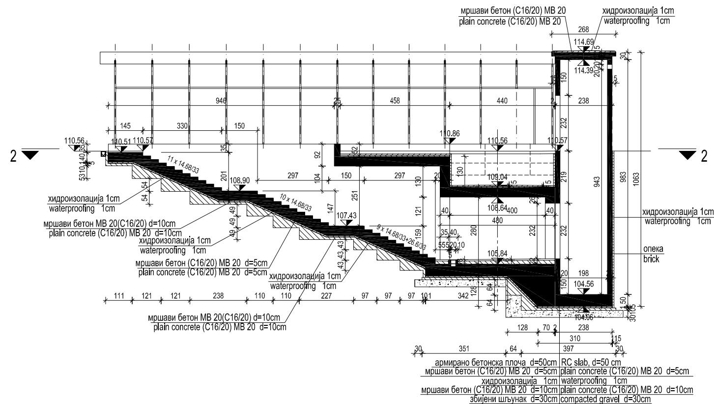
ПОПРЕЧНИ ПРЕСЕК 4-4 КРОЗ ПОТХОДНИК CROSS SECTION 4-4 THROUGH THE SUBWAY
