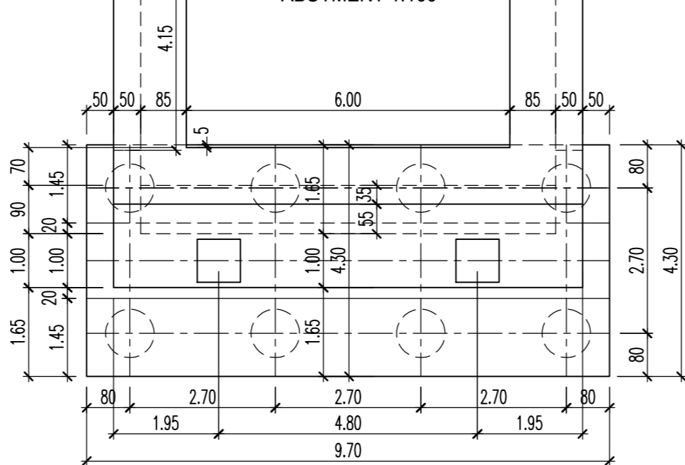
ОСНОВНО ТЕЛО С6 ABUTMENT 1:100
