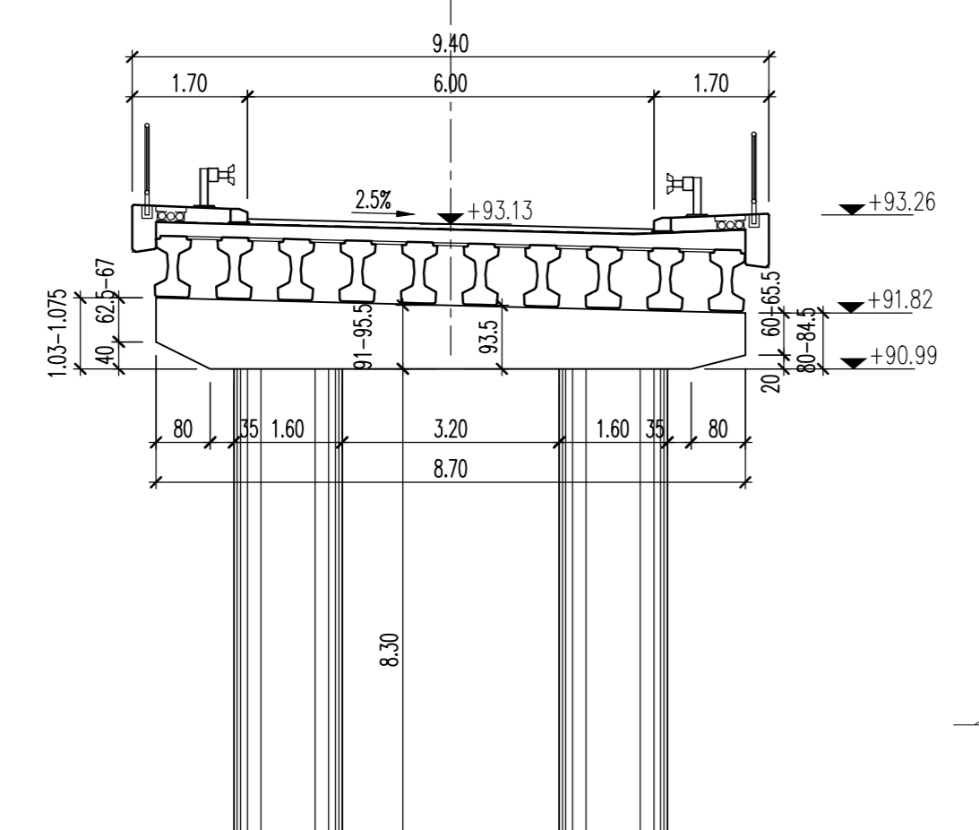
ПОПРЕЧНИ ПРЕСЕК СТУБА С3 CROSS SECTION С3 km 0+213.51 1:100
