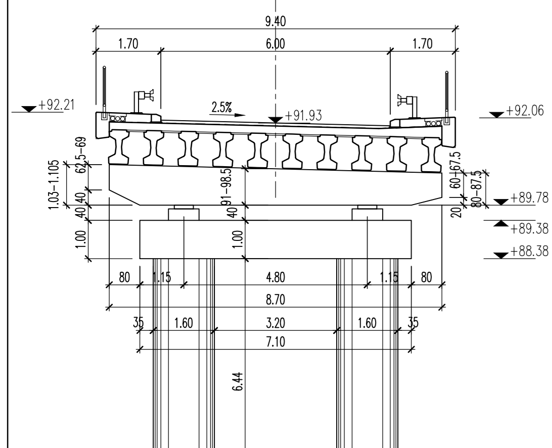
ПОПРЕЧНИ ПРЕСЕК СТУБА С2 CROSS SECTION km 0+190.31 1:100
