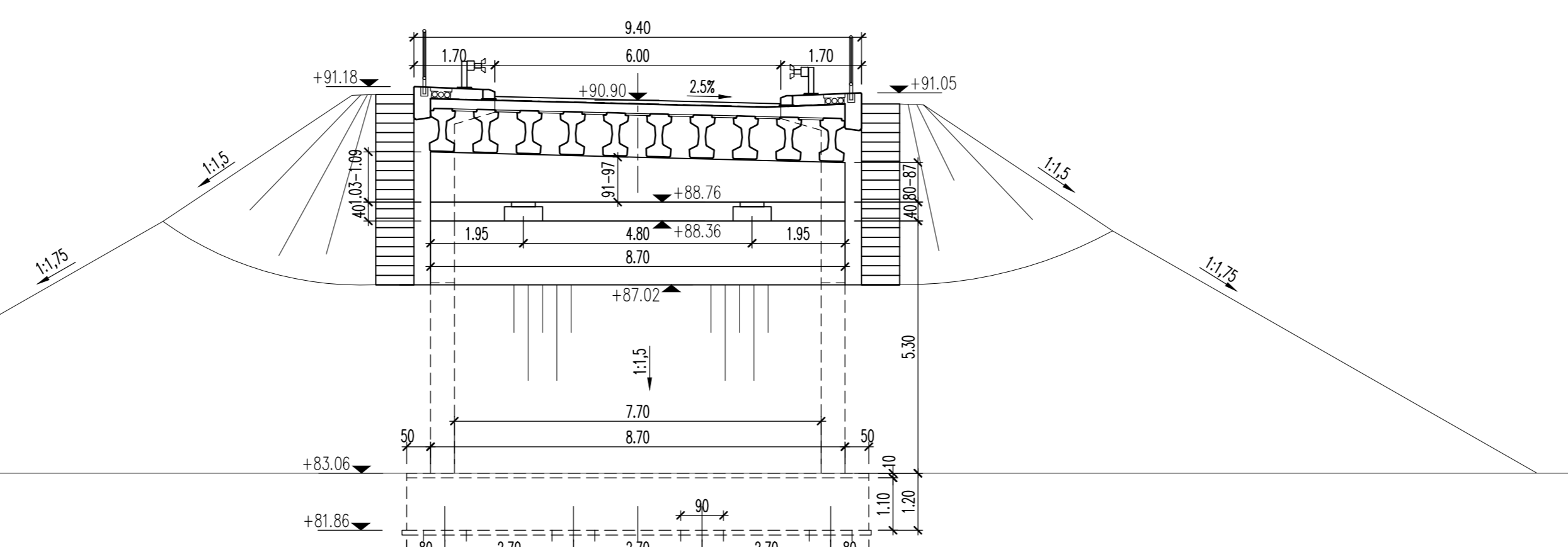
ПОПРЕЧНИ ПРЕСЕК СТУБА С6 CROSS SECTION С6 km 0+277.01 1:100
