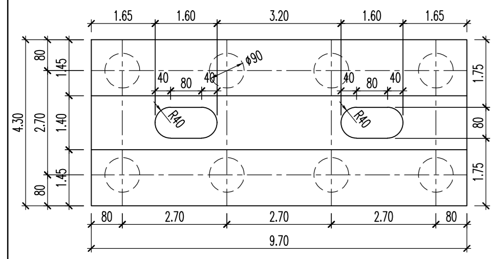
ОСНОВНА ТЕЛО С2 BASE 1:100
