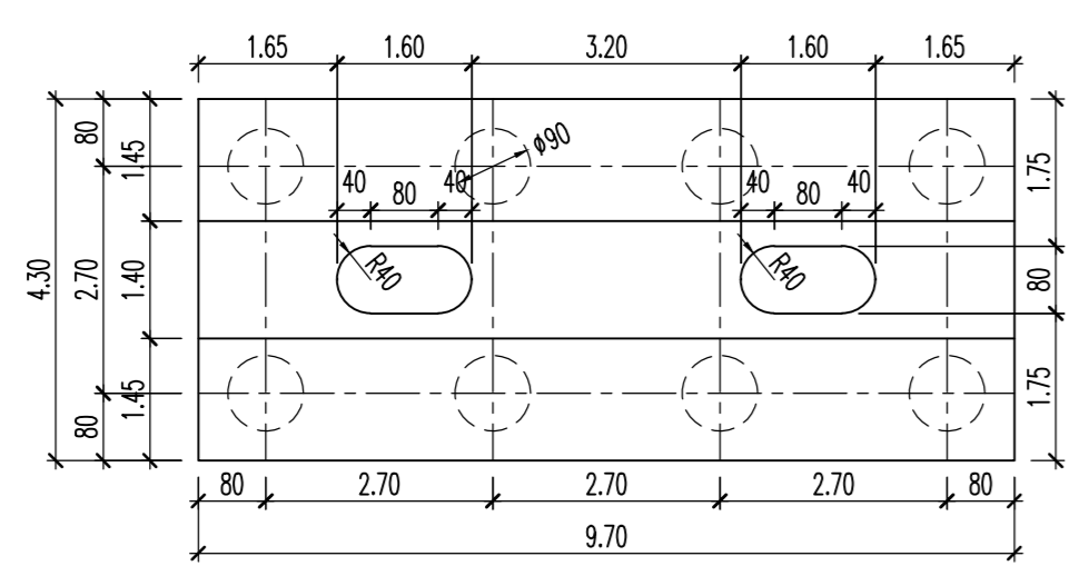
ОСНОВНА ТЕЛО С3 BASE 1:100
