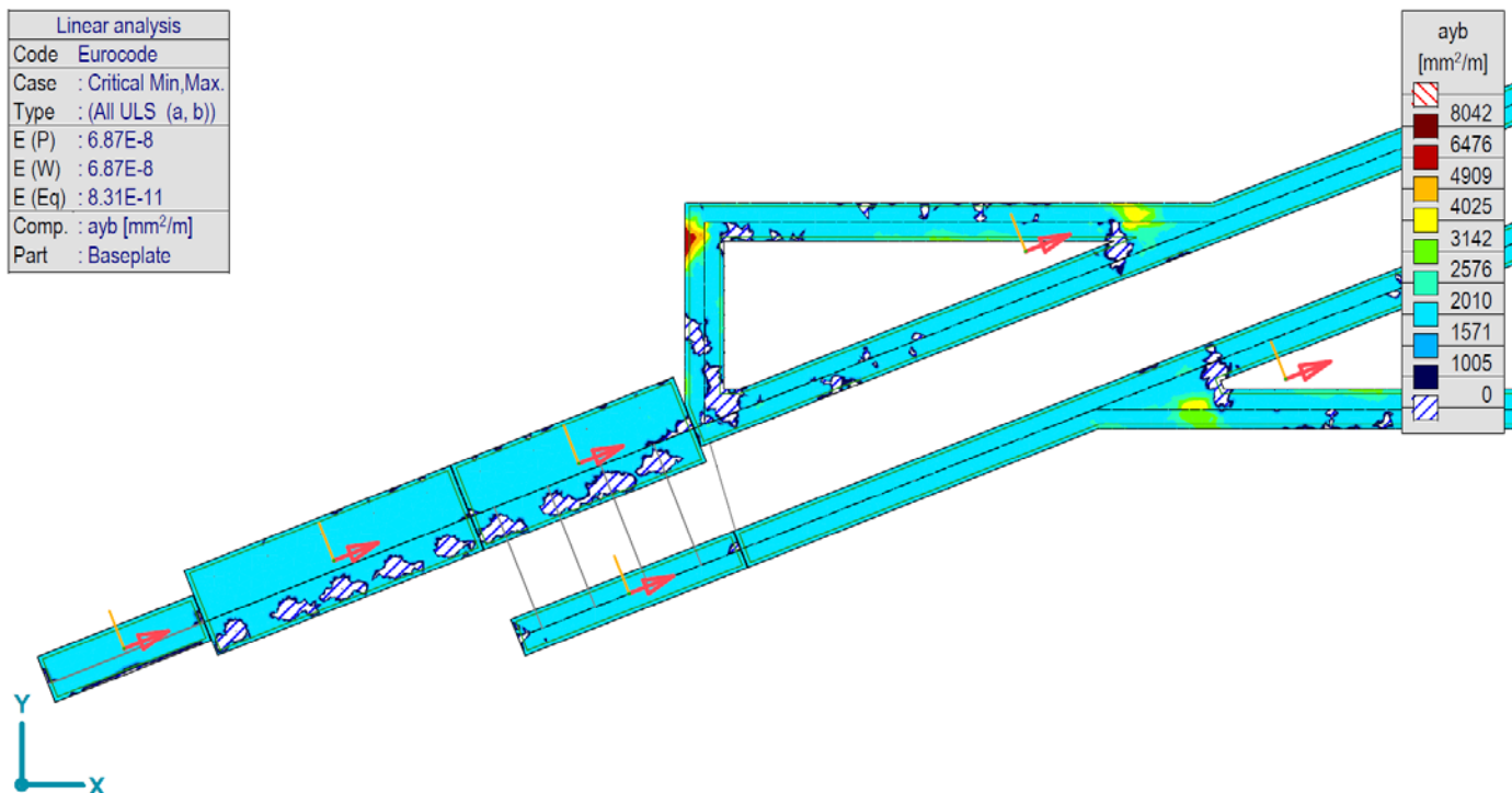
[RI], > Плоча, Linear, (Auto) Критично, ayb, Isosurfaces 2D, Горњи поглед
