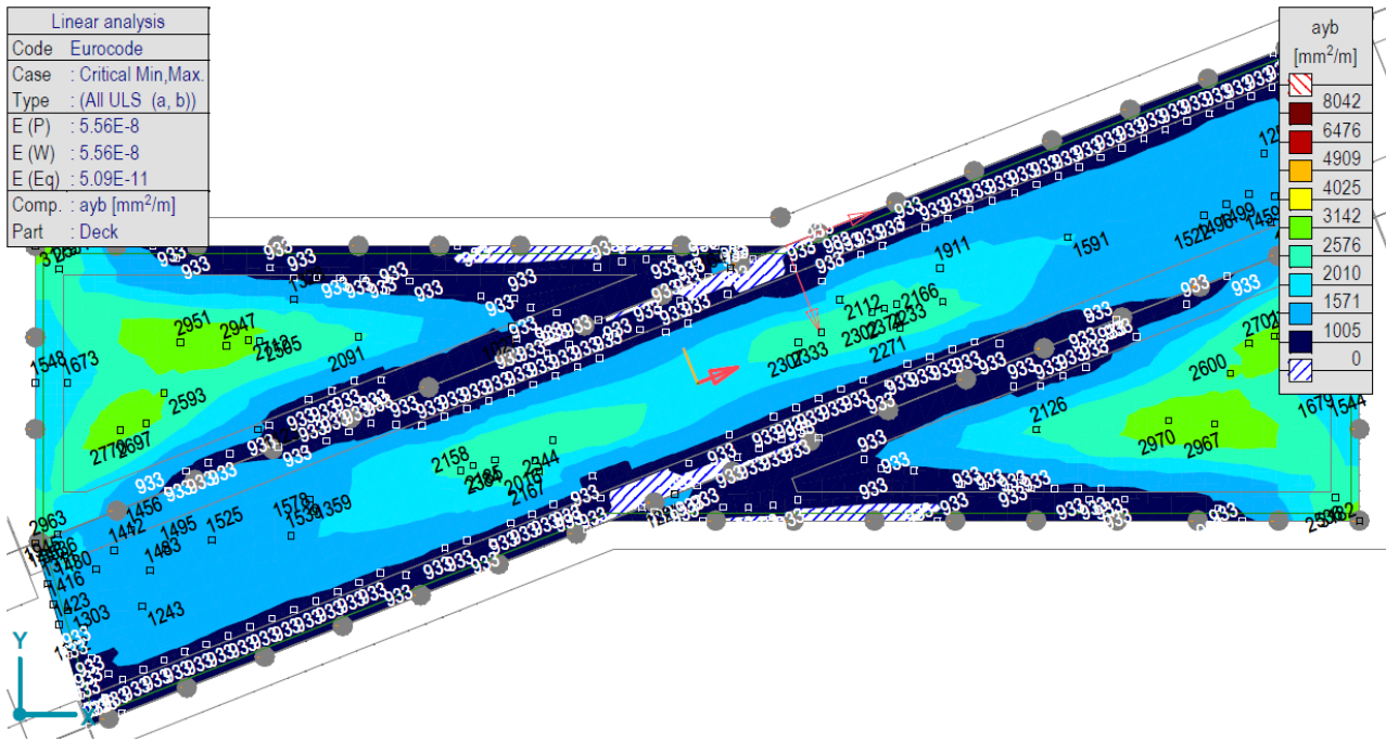
[RI], > Палуба, Линеарно, (Auto) Критично, ayb, Isosurfaces 2D, Горњи поглед
