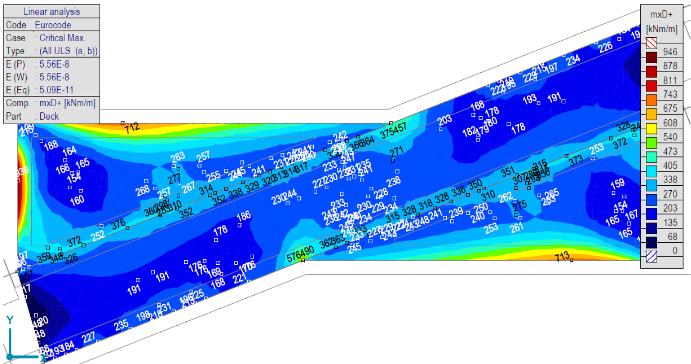
[I], > Палуба, Линеарно, (Auto) Крит. Мах., mxD+, Isosurfaces 2D, Горњи поглед
