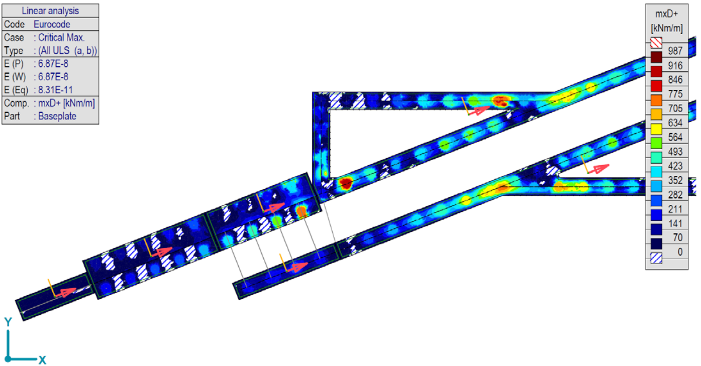
[[I]], > Плоча, Линеарно, (Auto) Критично макс., mxD+, Isosurfaces 2D, Горњи поглед
