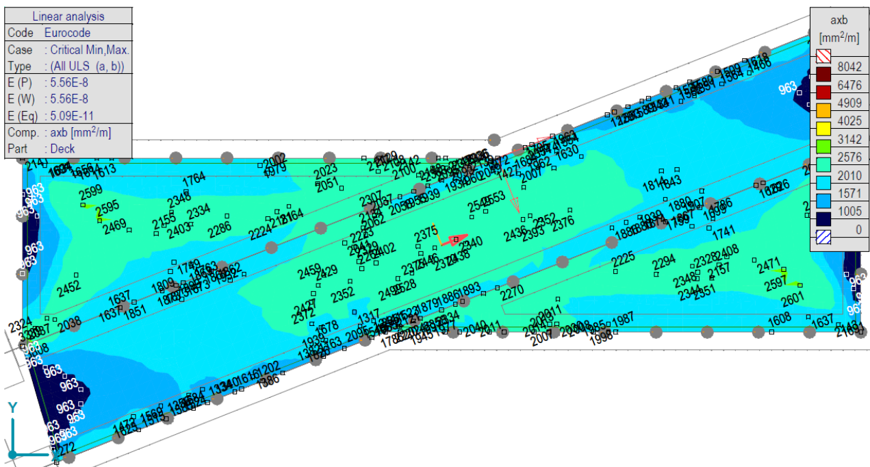
[R|], > Палуба, Лиенарно, (Auto) Крут., axb, Isosurfaces 2D, Горњи поглед
