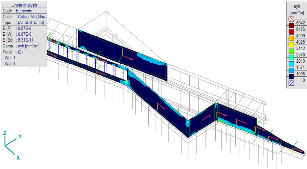
Количина арм. - [RI], > 2 дела, Линеарно,(Auto) Крив., ayb, Isosurfaces 2D
