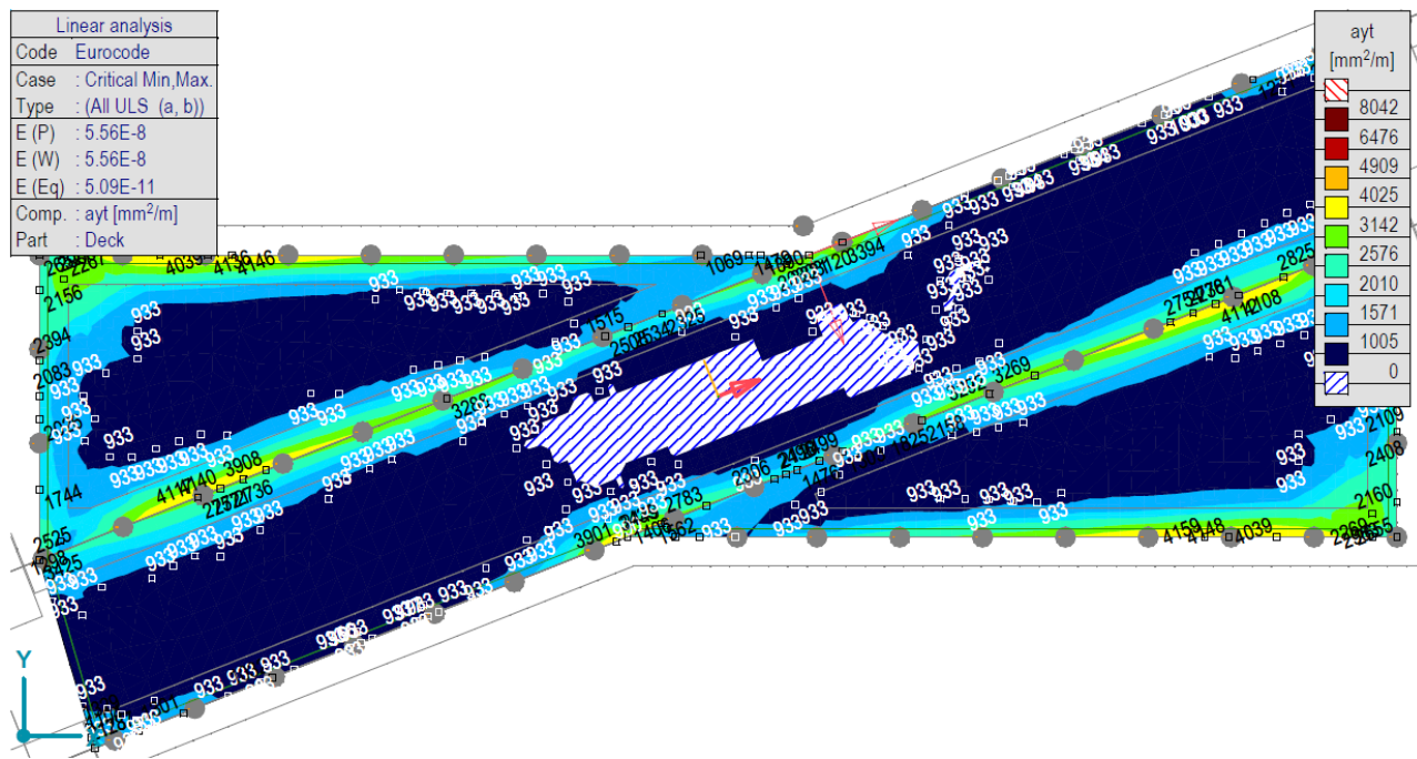
[RI], > Палуба, Линеарно, (Auto) Крит., ayt, Isosurfaces 2D, Горњи поглед
