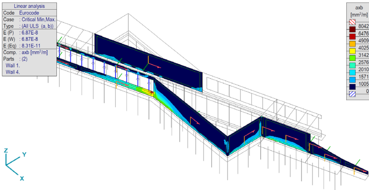
Количина арм. - [RI], > 2 дела, Количина арм. - Линеарно, (Auto) Крм., axb, Isosurfaces 2D
