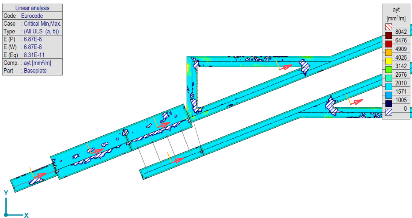
[RI], > Плоча, Линарно, (Auto) Критично, ayt, Isosurfaces 2D, Горњи поглед
