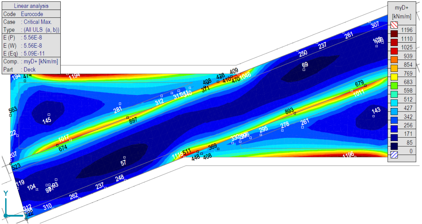
[I], > Палуба, Линеарно,(Auto) Крит. Мах., myD+, Isosurfaces 2D, Горњи поглед
