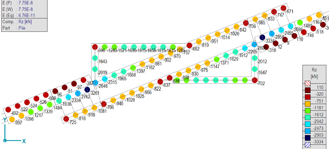
[I], > Шип, Линеарно,(Auto) Крит. Мах., Rz (зглобни осл.), Isosurfaces 2D, Горњи поглед
