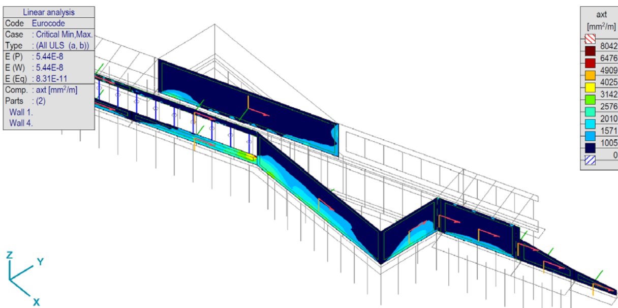
Количина арм. - [RI], > 2 дела, Линеарно, (Auto) Крм., axt, Isosurfaces 2D
