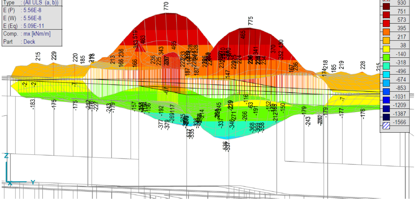
III, > Палуба, Линеарно,(Auto) Крм., mx, Isosurfaces 3D
