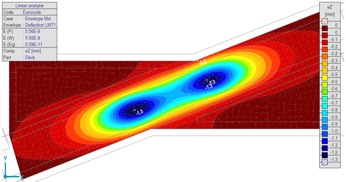
[[], > Палуба, Линеанро,(УгибLM71) Анвелопна Мин., e rel, Isosurfaces 2D, Горњи поглед
