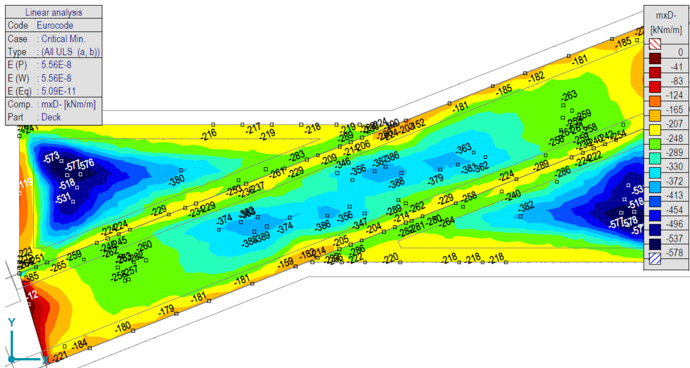
[I], > Палуба, Линеарно, (Auto) Крит. Мин., mxD-, Isosurfaces 2D, Горњи поглед
