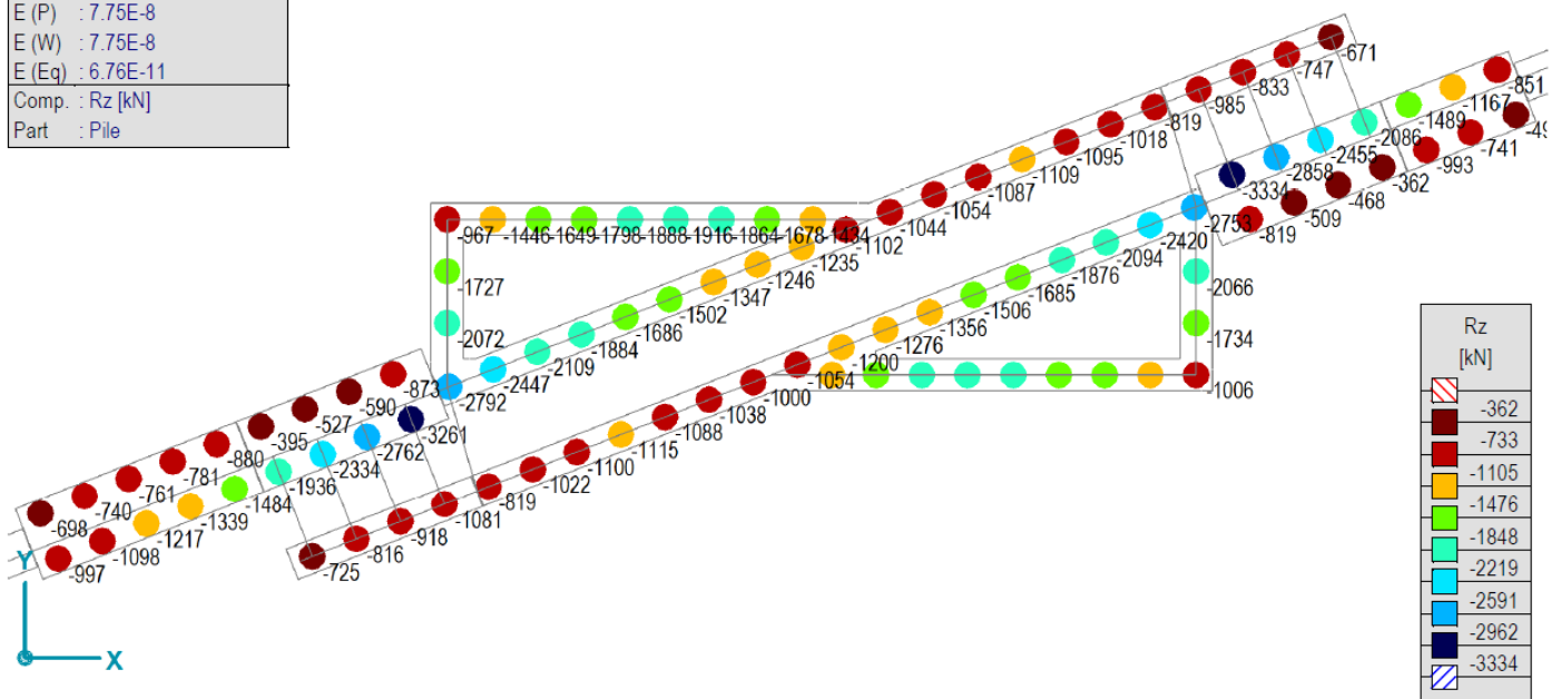
[I], > Шип, Линеанро,(ГСУ Квази-стално) Крит. мин., Rz (зглобни осл.), Isosurfaces 2D, Горњи поглед
