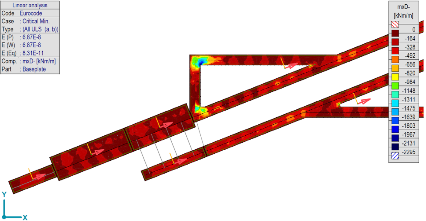
[[I]], > Плоча, Линеарно, (Auto) Критично Мин., mxD-, Isosurfaces 2D, Горњи поглед
