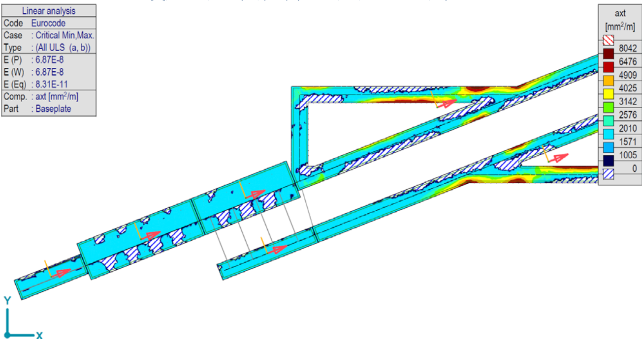
[R], > Плоча, Линеарно, (Auto) Критично, axt, Isosurfaces 2D, Горњи поглед
