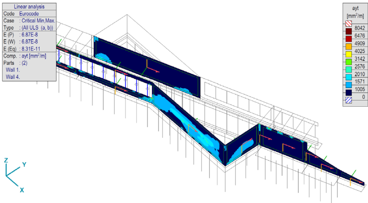
Количина арм. - [RI], > 2 дела, Линеарно,(Auto) Крив., ayt, Isosurfaces 2D
