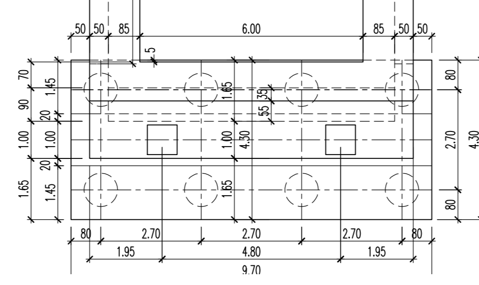
OSNOVNA ТЕЛО С8 BASE 1:100
