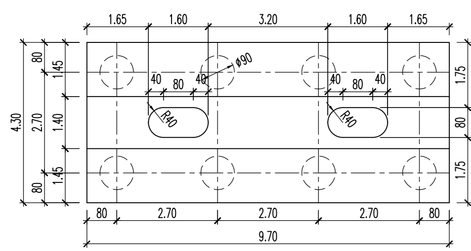
OSNOVNA ТЕЛО С2 BASE 1:100
