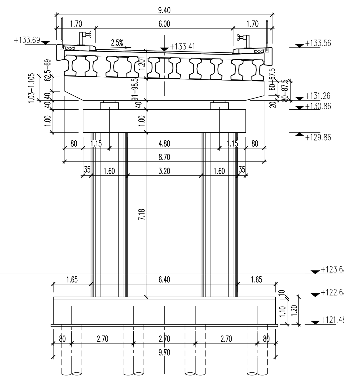
OSNOVNA ТЕЛО С2 BASE 1:100
