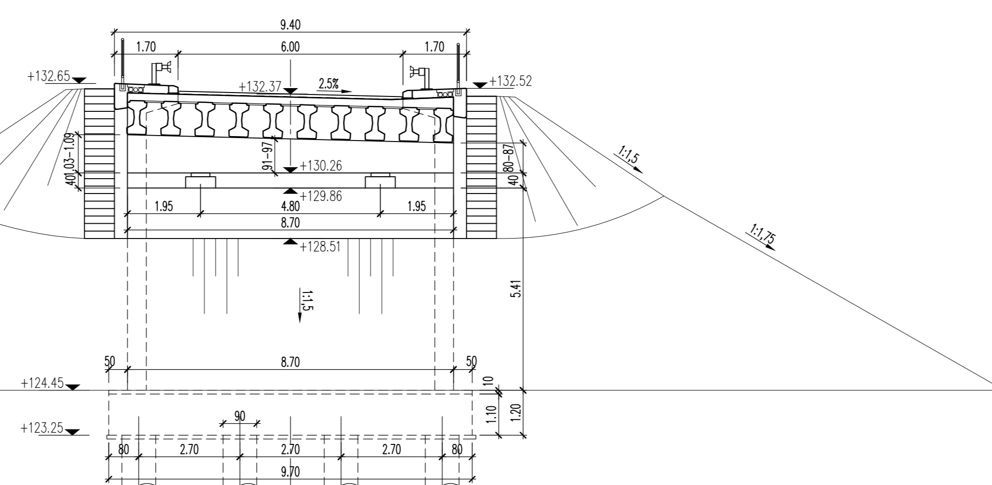
ПОПРЕЧНИ ПРЕСЕК СТУБА С8 CROSS SECTION С8 KM 1+102.38 1:100
