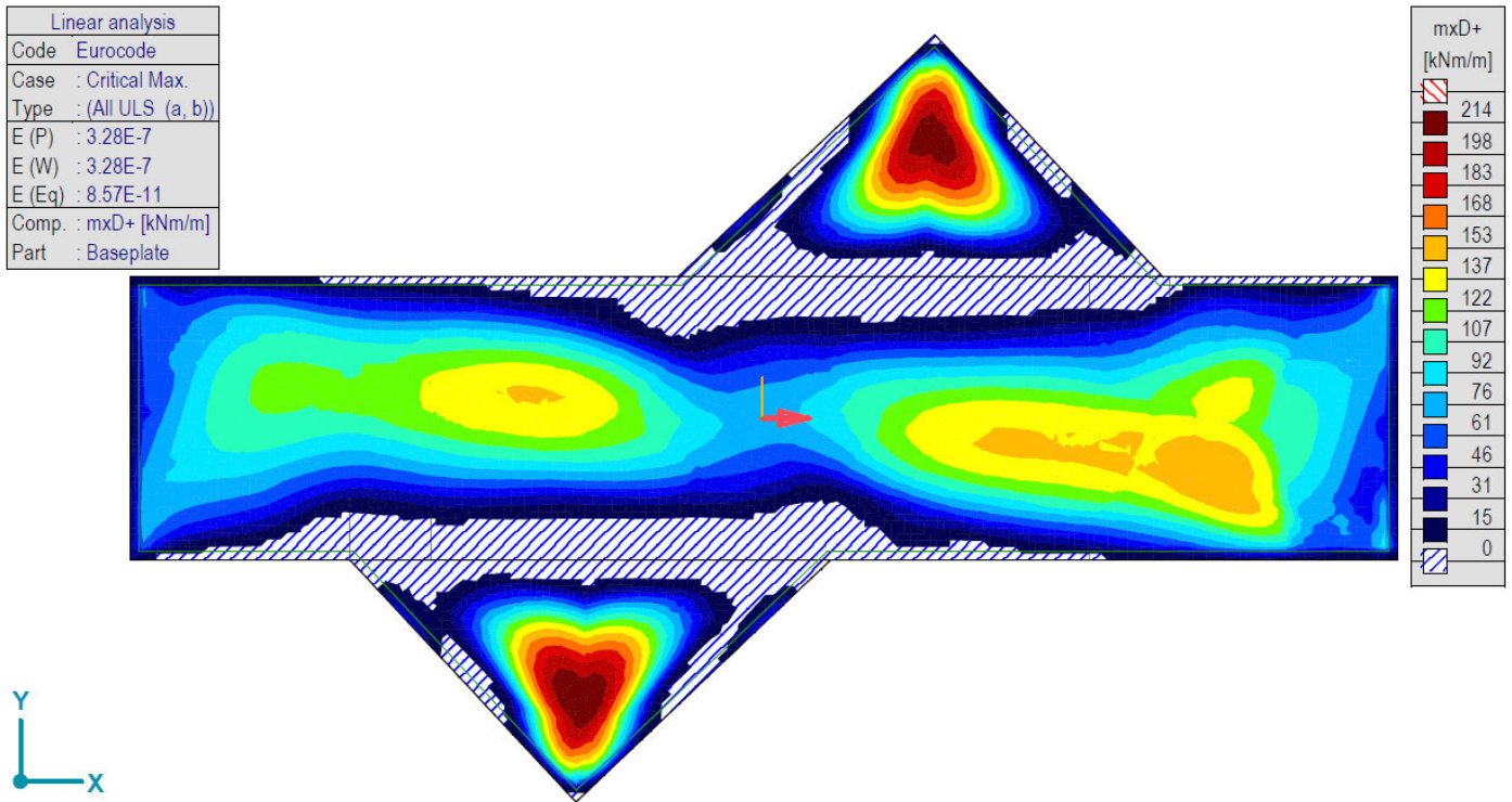
[[I], > Плоча, Линеарно,(Auto) Крит. Мах., mxD+, Isosurfaces 2D, Горњи поглед
