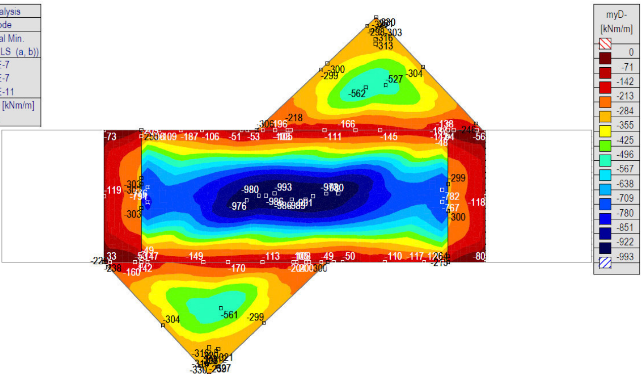
[[I], > Палуба, Линеарно, (Auto) Крит. мин., myD-, Isosurfaces 2D, Горњи поглед
