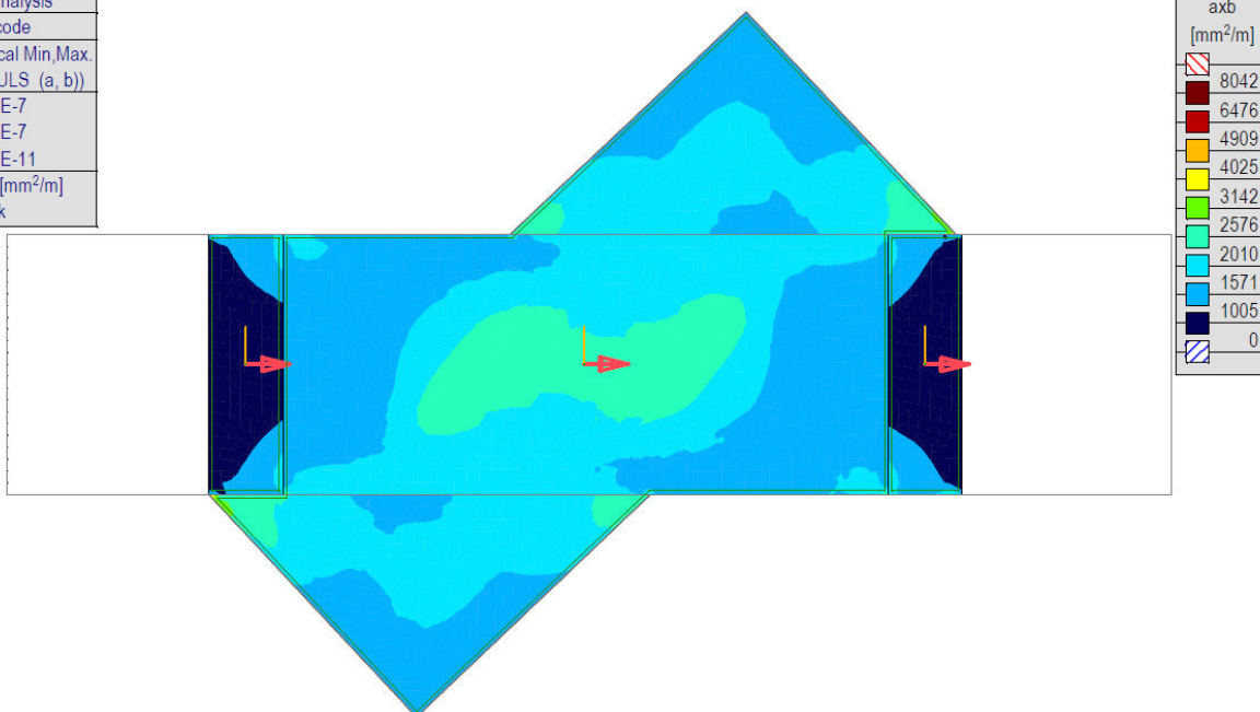
[RI], > Палуба, Линеарно,(Auto) Крит., axb, Isosurfaces 2D, Горњи поглед
