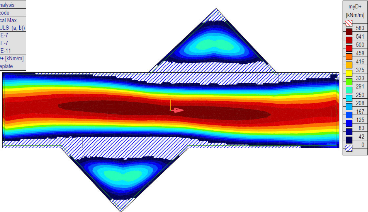
[[I], > Плоча, Линеарно,(Auto) Крит. макс..., myD+, Isosurfaces 2D, Горњи поглед
