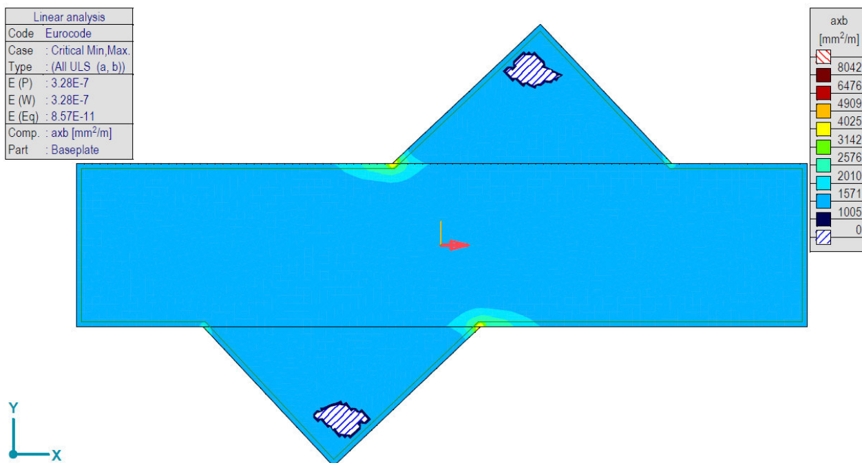
[R1], > Плоча, Линеарно, (Auto) Critical, axb, Isosurfaces 2D, Гоњрни поглед
