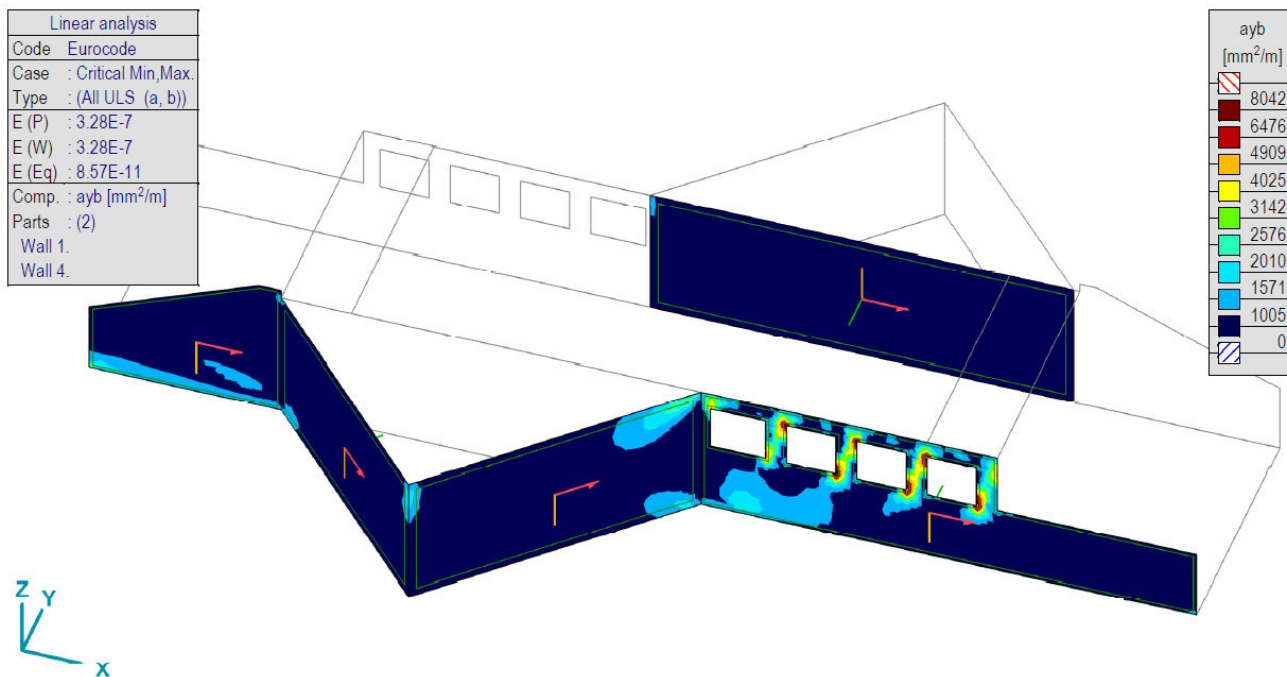
Кол. арм. - [R], > 2 parts, Линеарно,(Auto) Крив., ayb, Isosurfaces 2D
