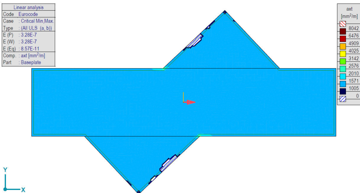
[R1], > Плоча, Линеарно, (Auto) Крит., axt, Isosurfaces 2D, Горњи поглед
