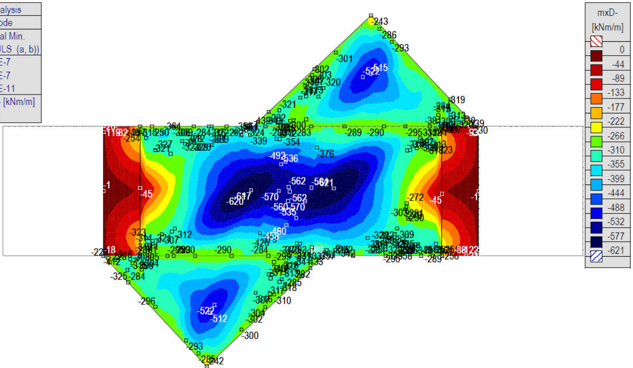
[I], > Палуба, Linear,(Auto) Крит. мин., mxD-, Isosurfaces 2D, Горњи поглед
