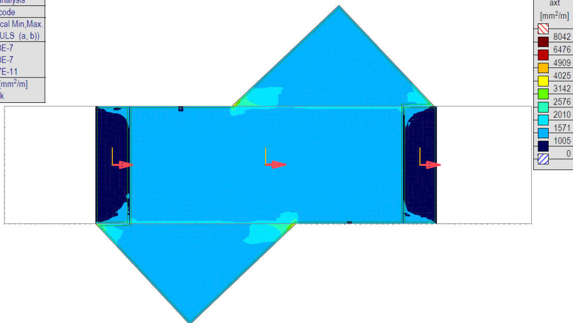
[RI], > Палуба, Линеарно,(Auto) Крит., axt, Isosurfaces 2D, Горњи поглед
