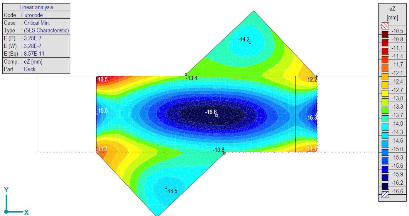
[I], > Палуба, Линеарно, (SLS Characteristic) Крит. мин., eZ, Isosurfaces 2D, Горњи поглед
