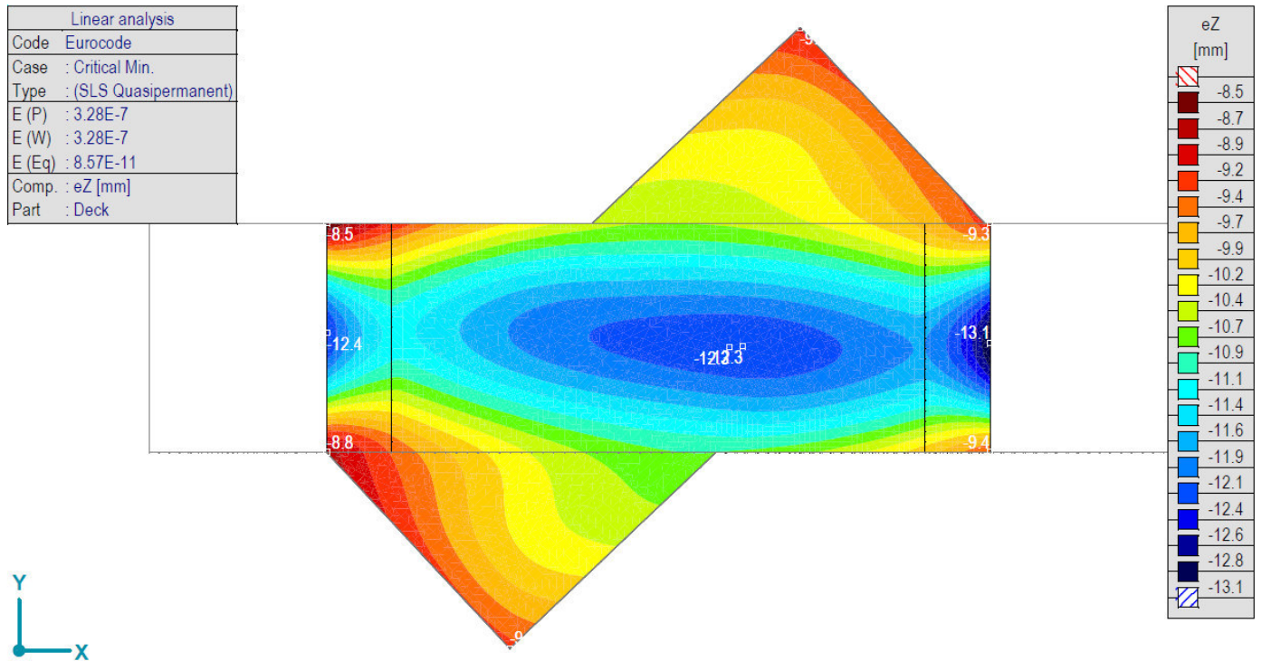
[I], > Палуба, Линеарно, (SLS Quasipermanent) Крит. мин., eZ, Isosurfaces 2D, Горњи поглед
