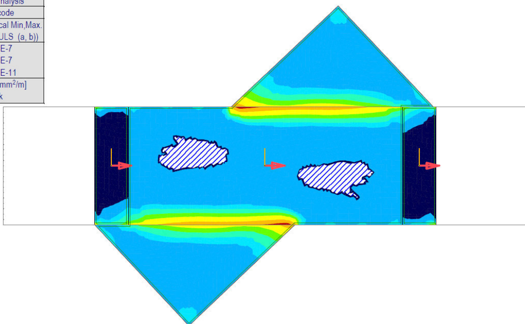
[RI], > Палуба, Линеарно,(Auto) Крит., ayt, Isosurfaces 2D, Горњи поглед
