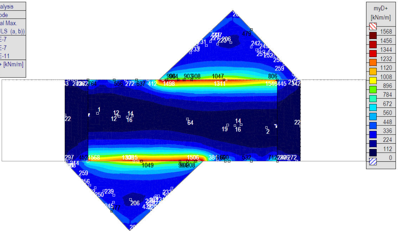
[[I], > Палуба, Линеарно, (Auto) Крит. макс., myD+, Isosurfaces 2D, Горњи поглед
