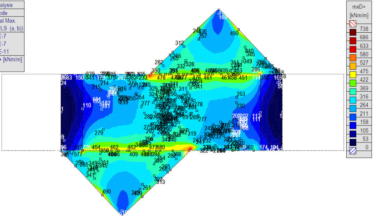
[I], > Палуба, Linear,(Auto) Крит. макс., mxD+, Isosurfaces 2D, Горњи поглед
