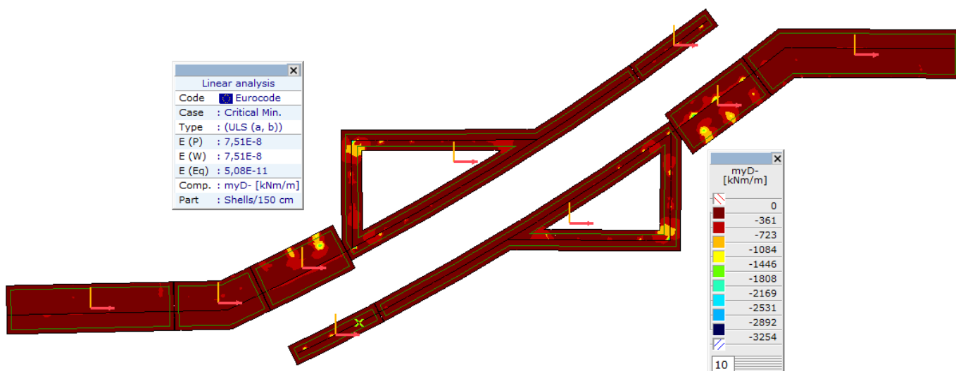
Плоча, Линеарно,(Auto) Критично мах., myD-, Isosurfaces 2D, Горњи поглед
