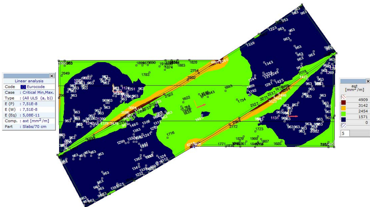
Палуба, Лиенарно,(Auto) Крит., axt, Isosurfaces 2D, Горњи поглед
