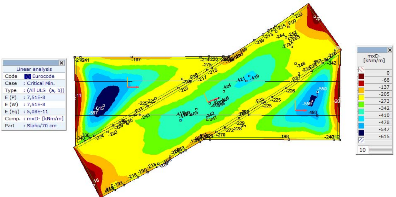
Палуба, Линеарно,(Auto) Крит. Мин., mxD-, Isosurfaces 2D, Горњи поглед
