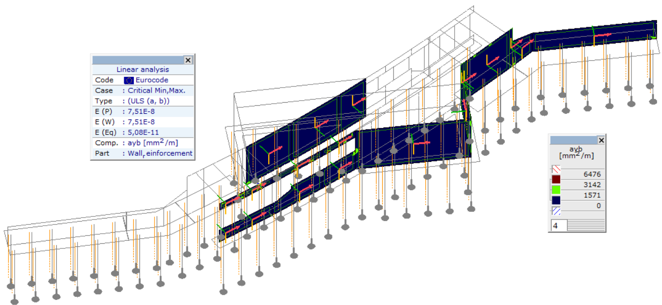
Количина арм.- Линеарно,(Auto) Кpum., ayb, Isosurfaces 2D
