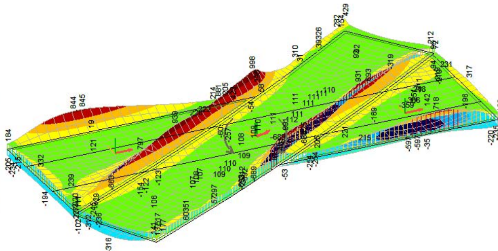
Палуба, Лінейно,(Auto) Крив., my, Isosurfaces 3D
