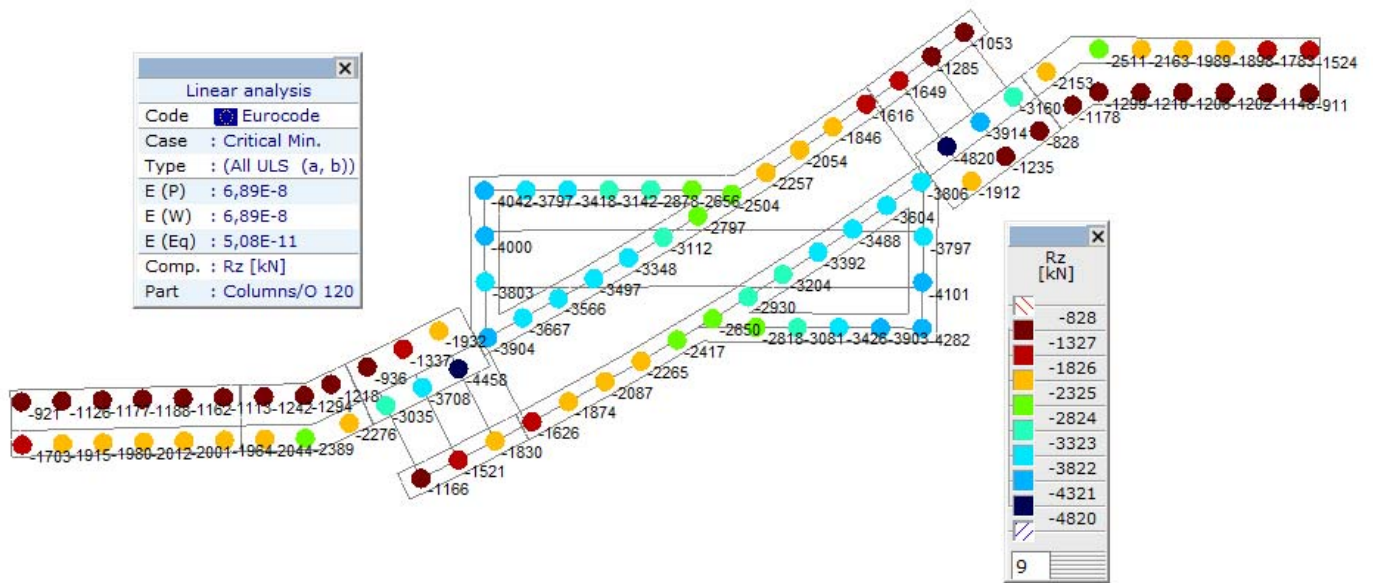
Шип, Линеарно, (Auto) Критично Мин., Rz (зглобни осл.), Isosurfaces 2D, Горњи поглед
