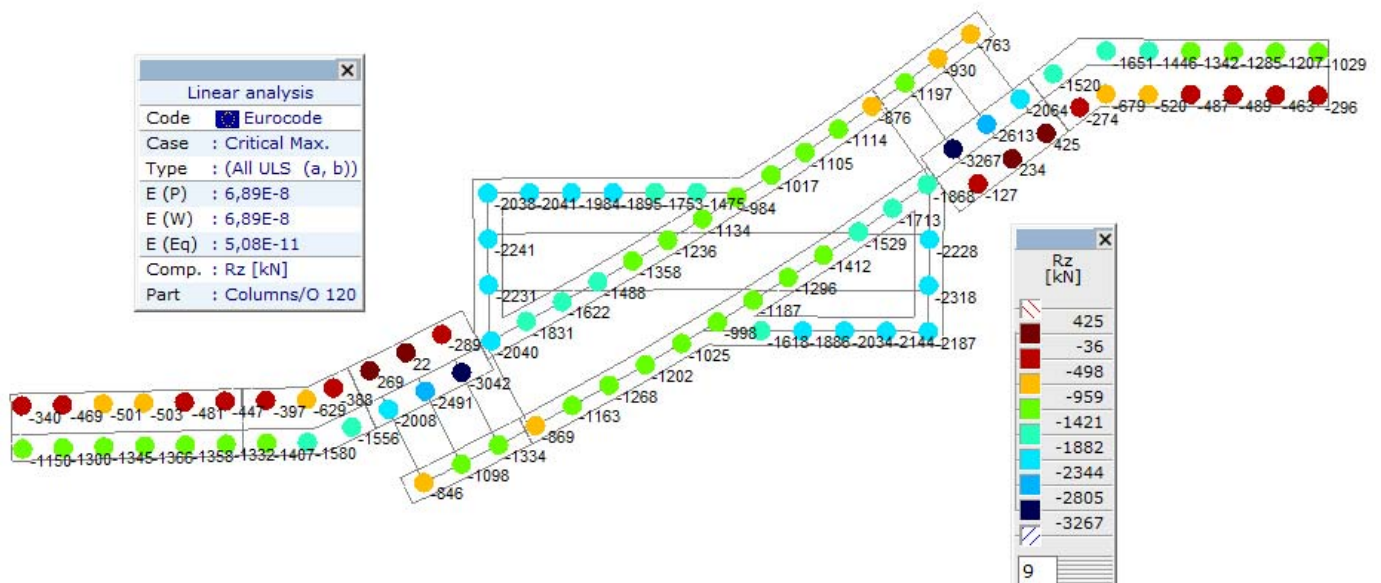
Шип, Линеарно, (Auto) Крит. Мах., Rz (зглобни осл.), Isosurfaces 2D, Горњи поглед
