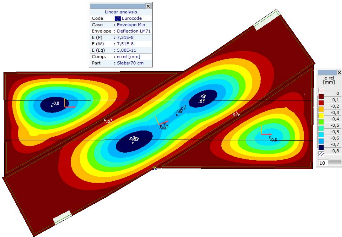
Палуба, Линеанро,(УгибLM71) Анвелопа Мин., e rel, Isosurfaces 2D, Горњи поглед
