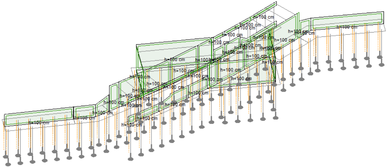
Дебљина елемента - зидови
