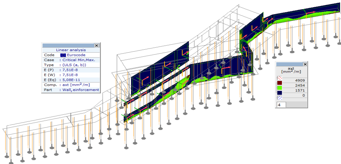
Количина арм.- Линеарно, (Auto) Крут., axt, Isosurfaces 2D
