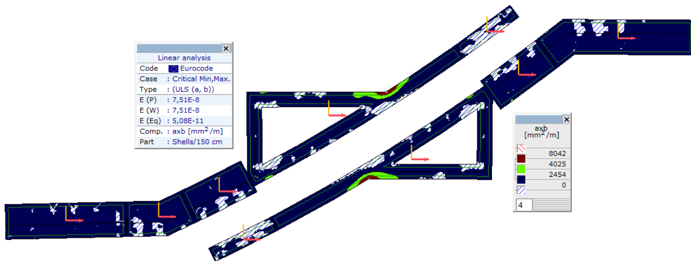
Плоча, Линеарно, (Auto) Критично, axb, Isosurfaces 2D, Горњи поглед
