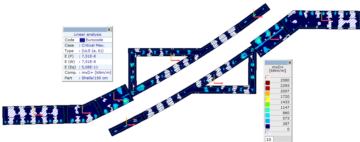
Плоча, Линеарно, (Auto) Критично макс., mxD+, Isosurfaces 2D, Горњи поглед
