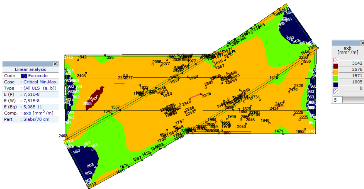
Палуба, Лиенарно,(Auto) Крит., axb, Isosurfaces 2D, Горњи поглед
