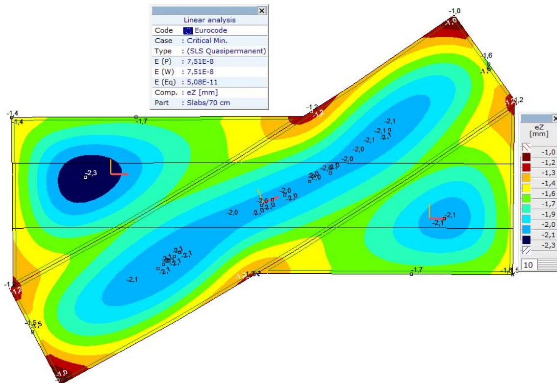
Палуба, Линеарно,(SLS Quasipermanent) Крит. мин., eZ, Isosurfaces 2D, Горњи поглед
