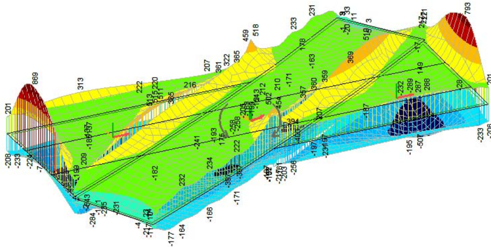
Палуба, Лінейно,(Auto) Крив., mx, Isosurfaces 3D
