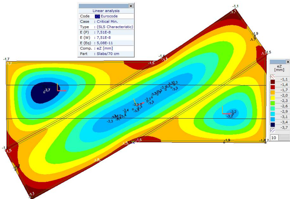
Палуба, Линеарно,(ГСУ каракт.) Крит. Мин., eZ, Isosurfaces 2D, Горњи поглед
