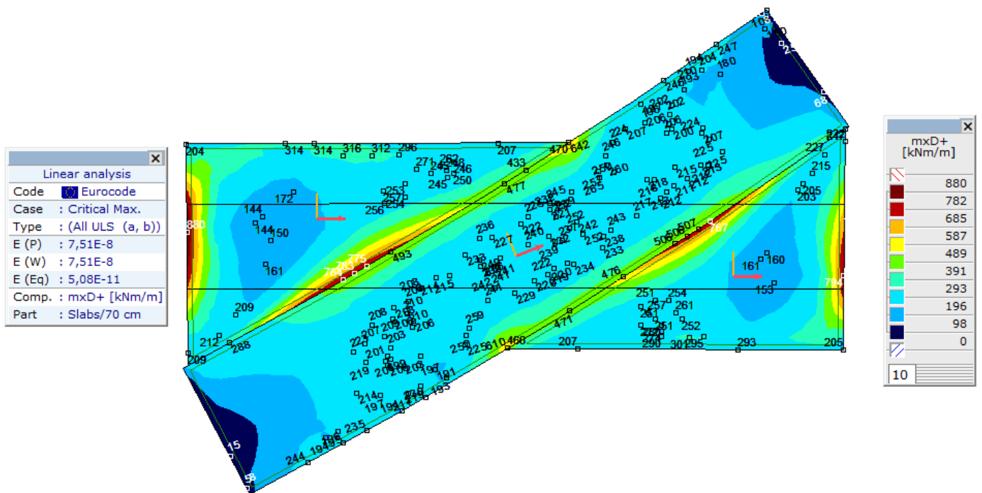
Палуба, Линеарно,(Auto) Крит. Мах., mxD+, Isosurfaces 2D, Горњи поглед
