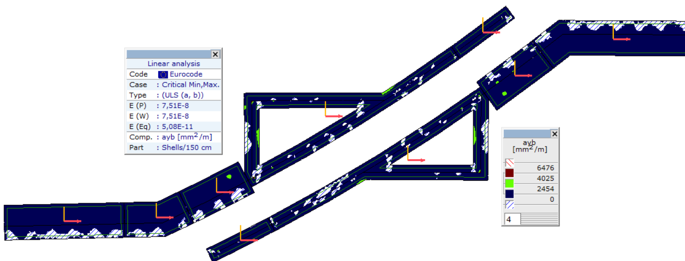
Плоча, Linear, (Auto) Критично, ayb, Isosurfaces 2D, Горњи поглед
