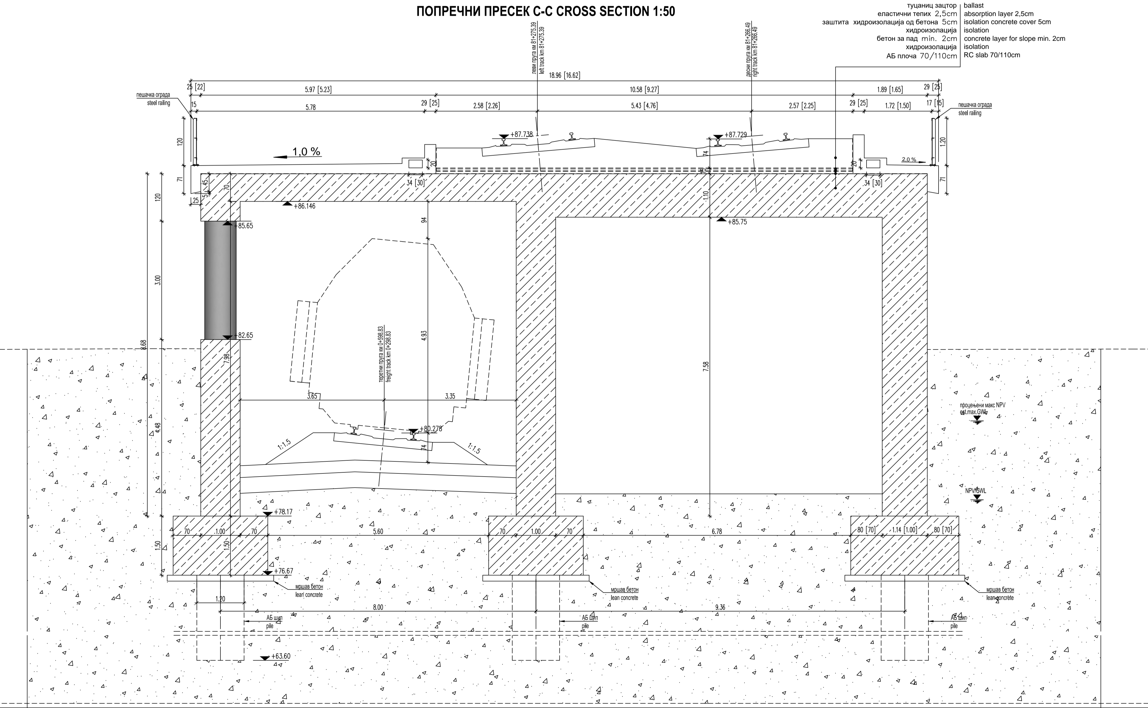
ПОПРЕЧНИ ПРЕСЕК С-С CROSS SECTION 1:50
