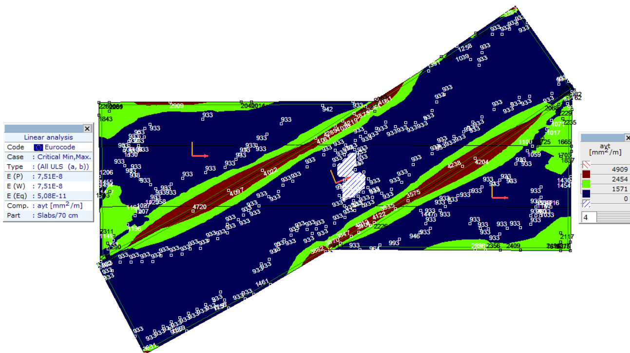
Палуба, Линеарно,(Auto) Крит., ayt, Isosurfaces 2D, Горњи поглед
