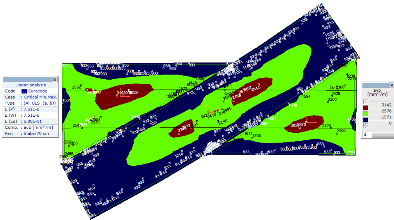
Палуба, Линеарно,(Auto) Критично, ayb, Isosurfaces 2D, Горњи поглед
