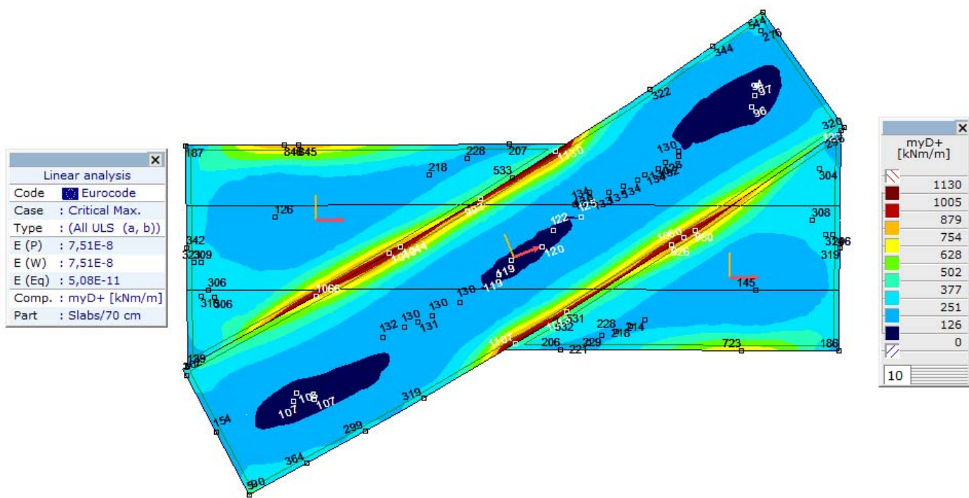
Палуба, Линеарно,(Auto) Крит. Max., myD+, Isosurfaces 2D, Горњи поглед
