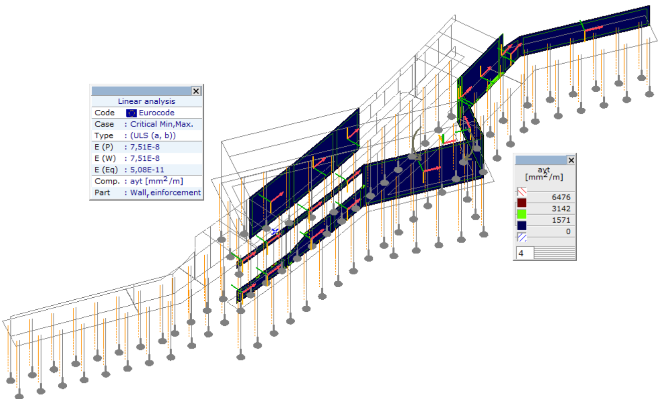
Количина арм. - Линеарно,(Auto) Кpum., ayt, Isosurfaces 2D
