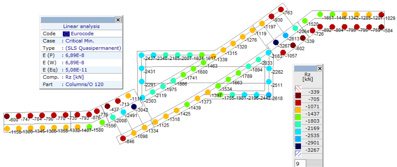
Шип, Линеарно,(ГСУ Квази-стално) Крит. мин., Rz (зглобни осл.), Isosurfaces 2D, Горњи поглед
