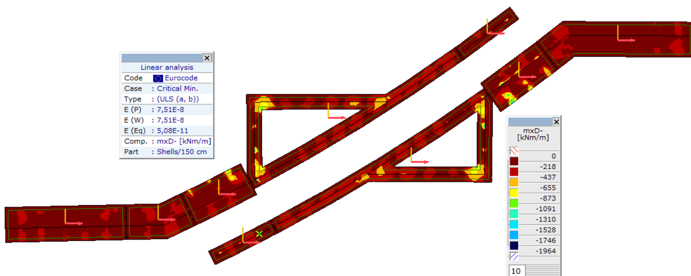
Плоча, Линеарно, (Auto) Критично Мин., mxD-, Isosurfaces 2D, Горњи поглед
