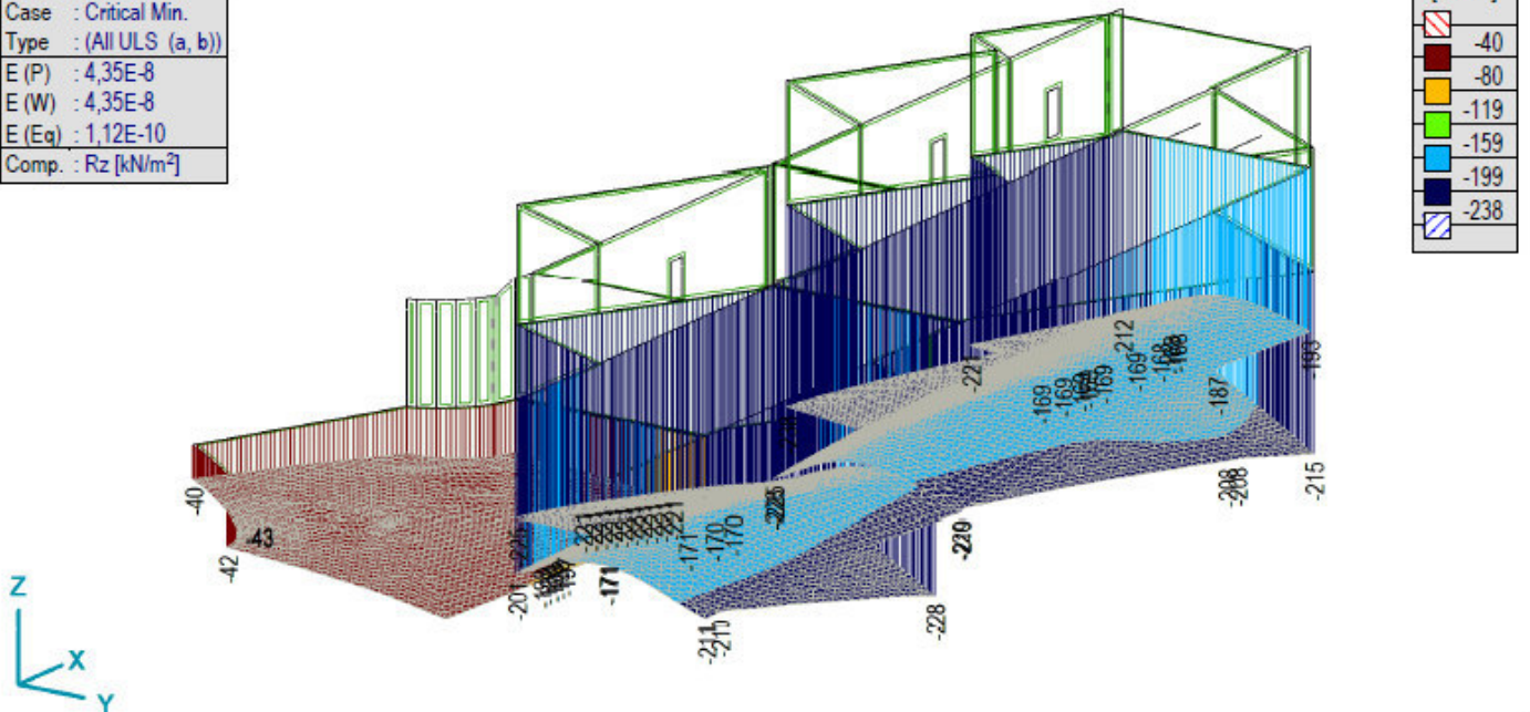
[I], Линеарно,(Auto) Крит. мин..., Rz (surf. supp.), Isosurfaces 3D
