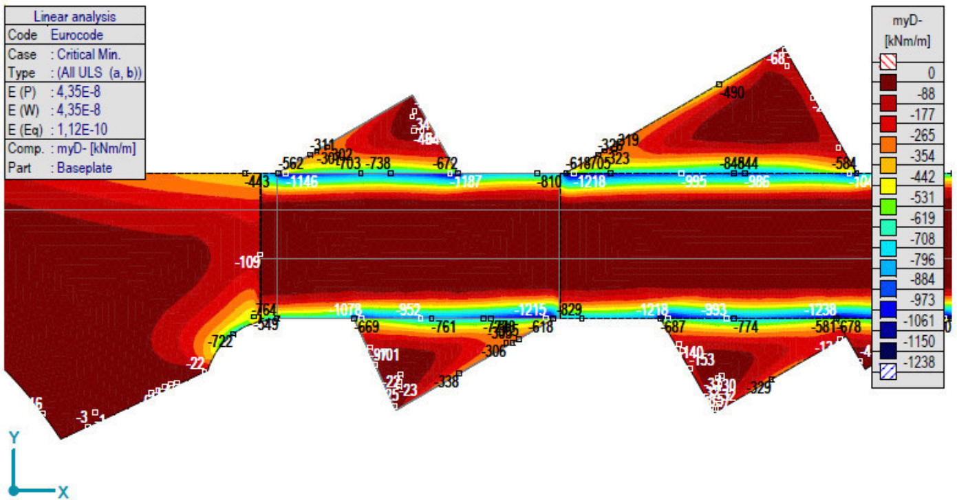
[[], > Плоча, Линеарно,(Auto) Крит. мин..., myD-, Isosurfaces 2D, Горњи поглед
