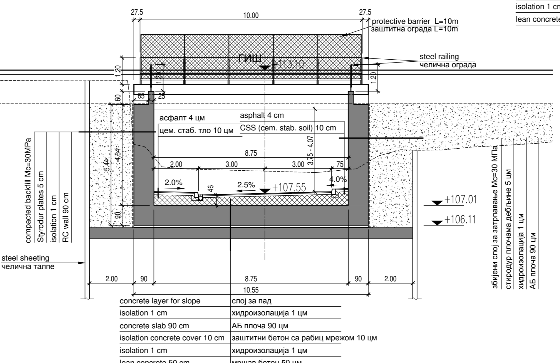
ПОПРЕЧНИ ПРЕСЕК 1:100 CROSS SECTION 2-2
