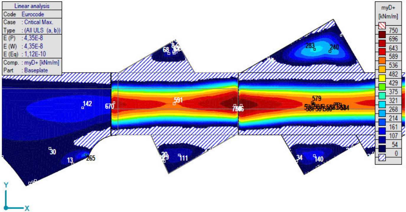
[[], > Плоча, Линеарно,(Auto) Крит. макс..., myD+, Isosurfaces 2D, Горњи поглед
