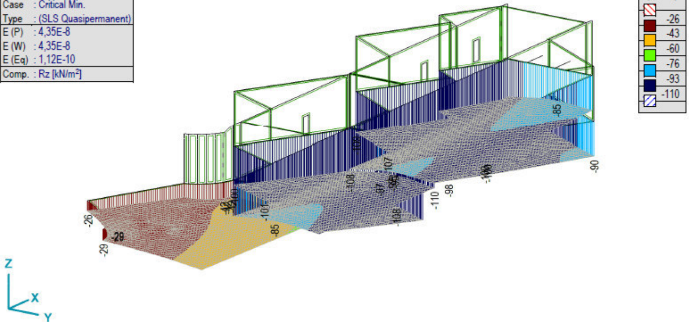
[I], Линеарно,(SLS Квази-стално) Крит. мин..., Rz (surf. supp.), Isosurfaces 3D
