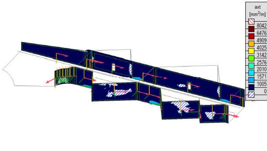
Кол. арм. - [R], > 2 parts, Линеарно,(Auto) Крив., axt, Isosurfaces 2D
