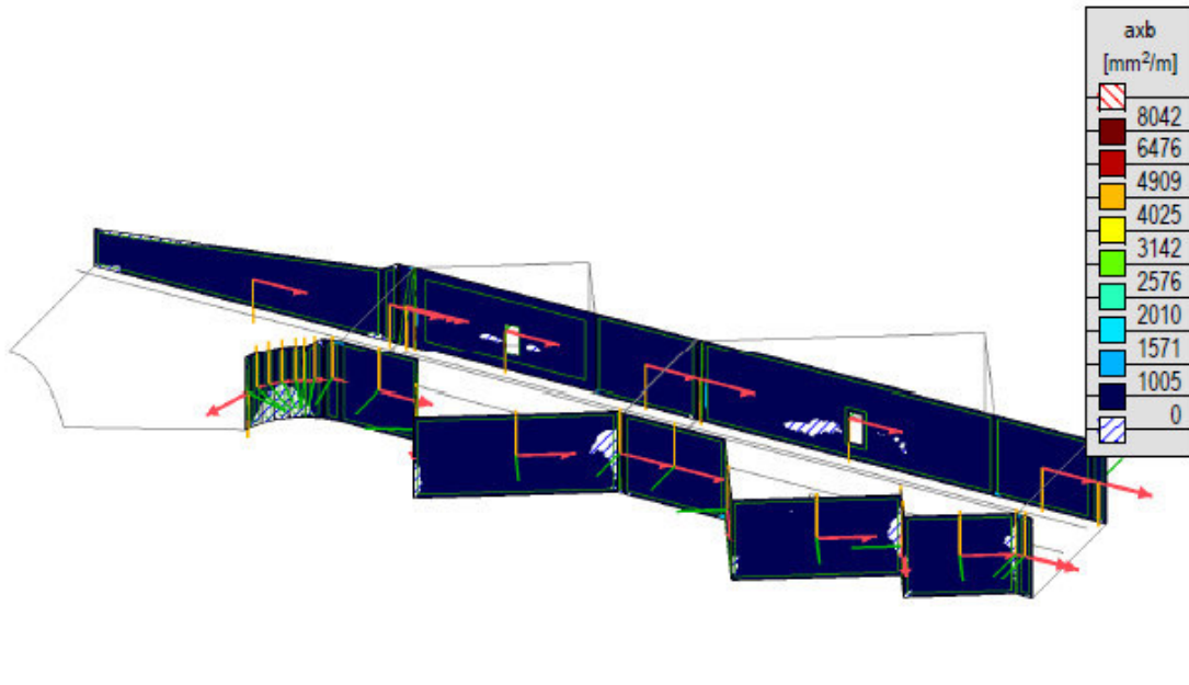
Кол. арм. - [R], > 2 дела, Линеарно,(Auto) Крив., axb, Isosurfaces 2D
