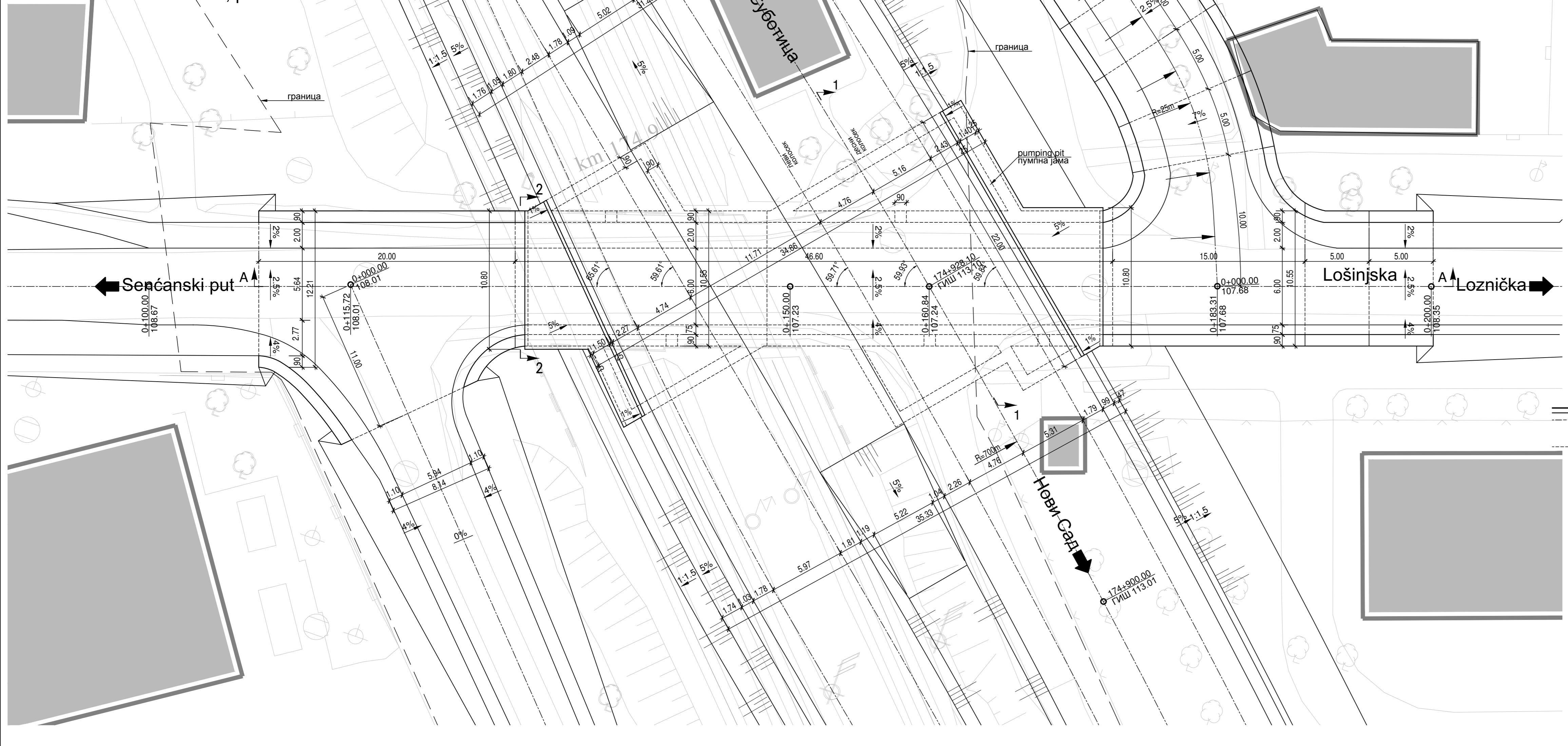
ОСНОВА ПОДВОЖЊАКА / UNDERPASS LAYOUT 1:200
