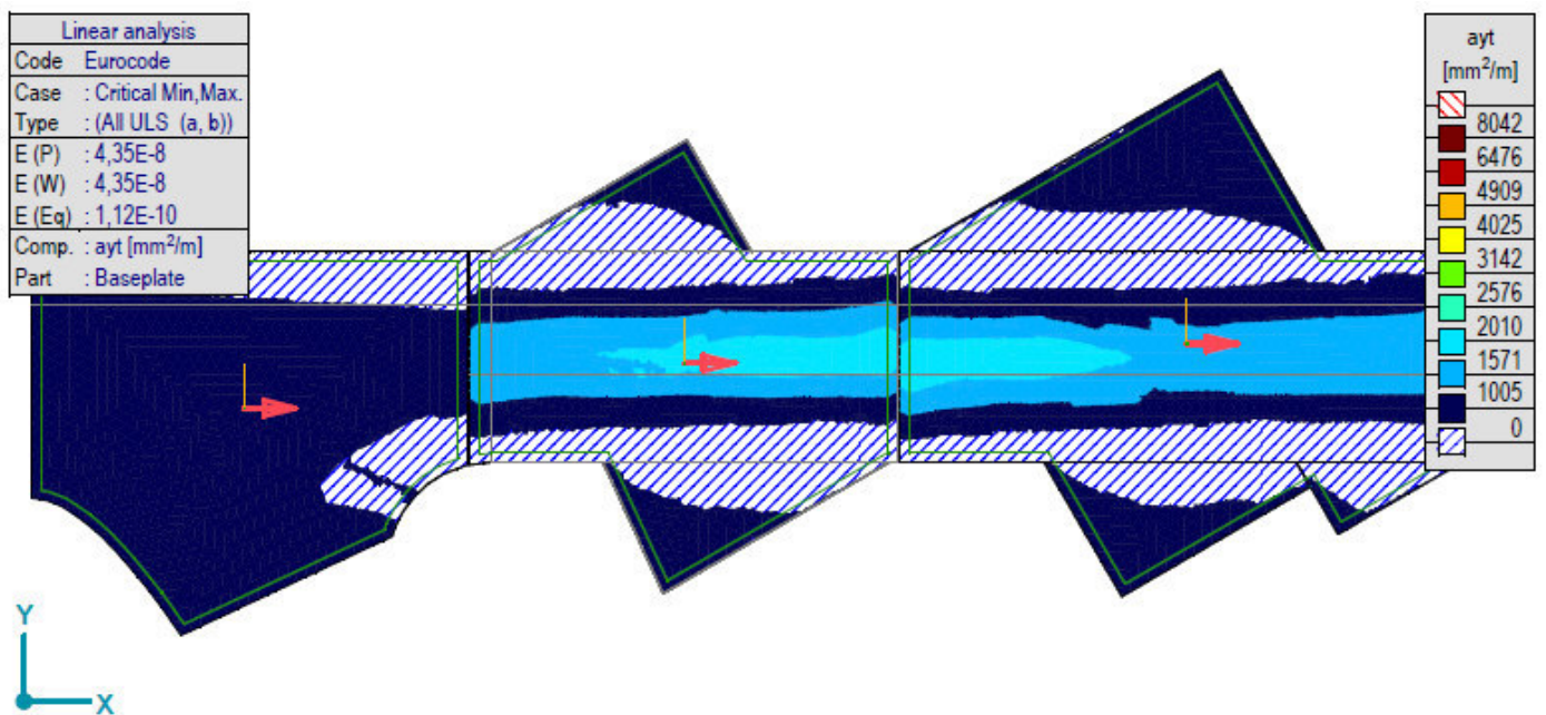
[RI], > Плоча, Линеарно,(Auto) Крив., аyt, Isosurfaces 2D, Горњи поглед
