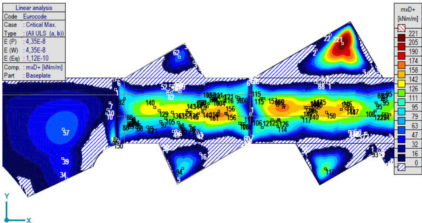
[[I], > Плоча, Линеар,(Auto) Крит. Max., mxD+, Isosurfaces 2D, Горњи поглед
