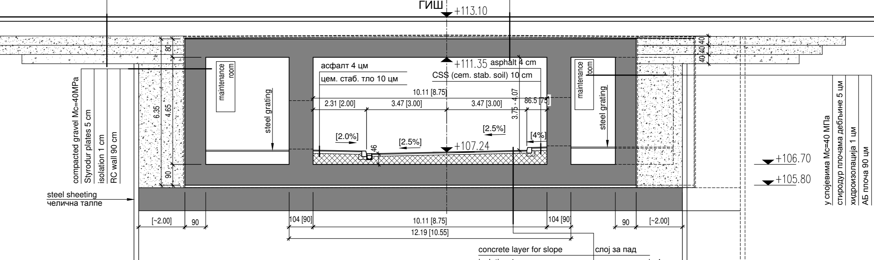
ПОПРЕЧНИ ПРЕСЕК 1:100 CROSS SECTION 2-2
