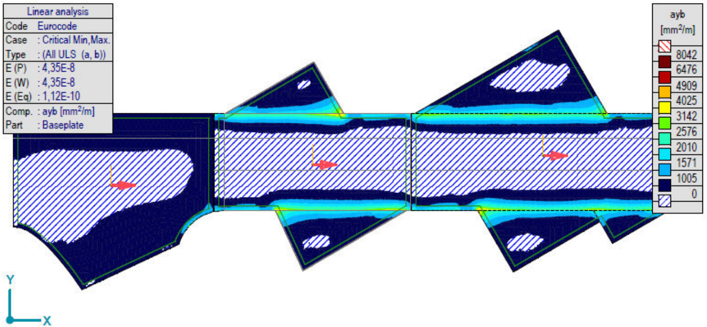
[RI], > Плоча, Линеарно,(Auto) Крив., ахт, Isosurfaces 2D, Горњи поглед
