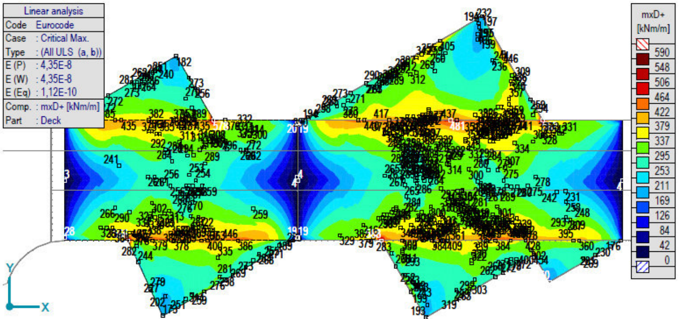
[[I], > Палуба, Linear,(Auto) Крит. макс., mxD+, Isosurfaces 2D, Горњи поглед
