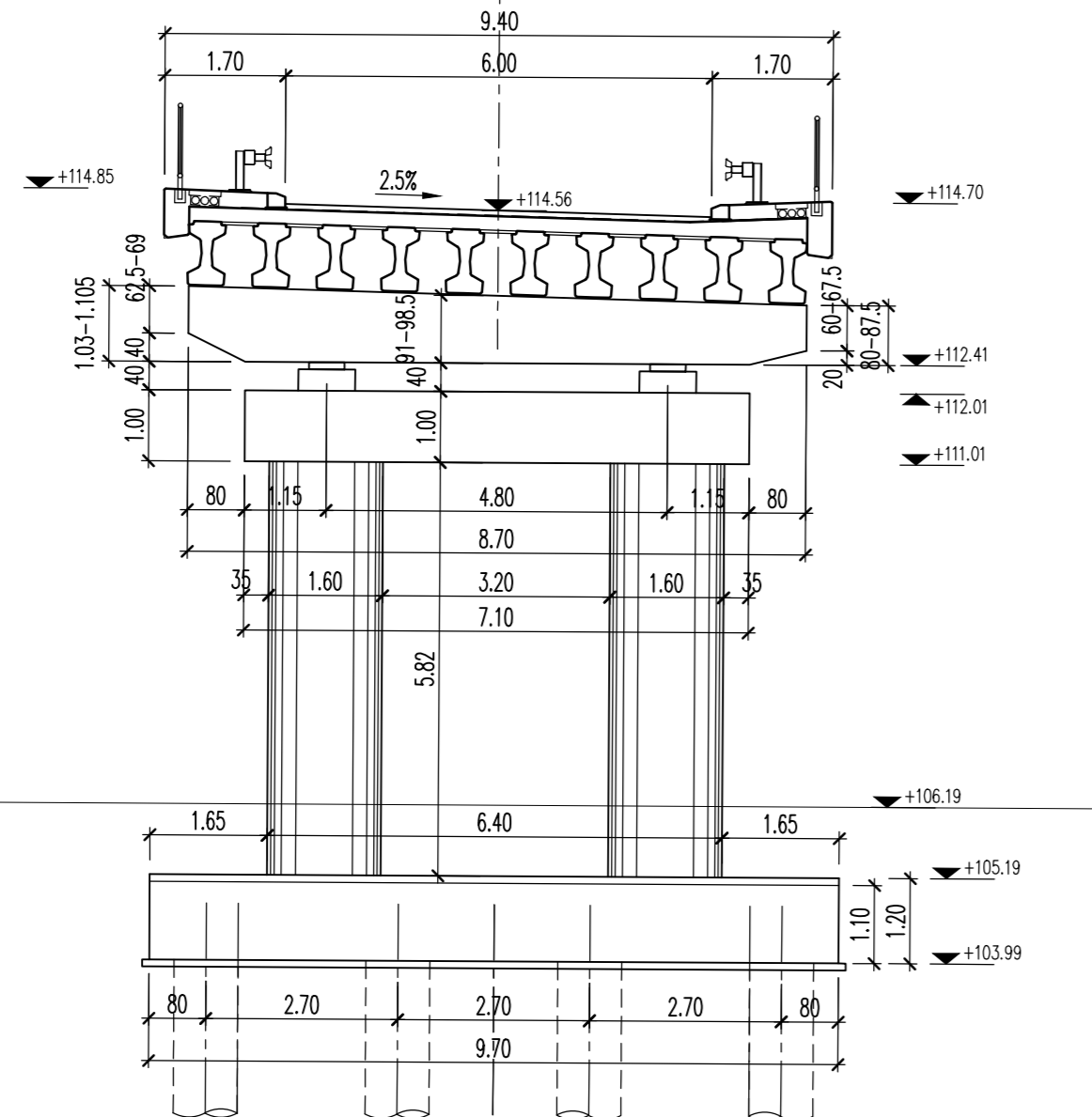
ПОПРЕЧНИ ПРЕСЕК СТУБА С8 CROSS SECTION C8 km 0+426.77 1:100
