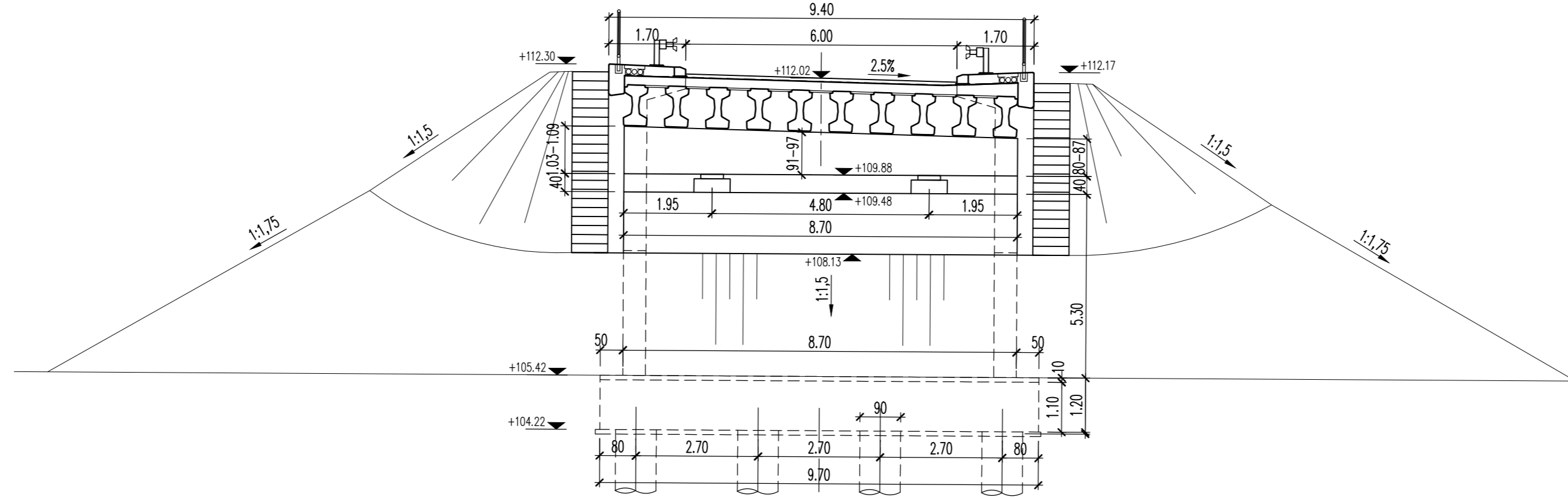
ПОПРЕЧНИ ПРЕСЕК СТУБА С10 CROSS SECTION C10 km 0+469.07 1:100
