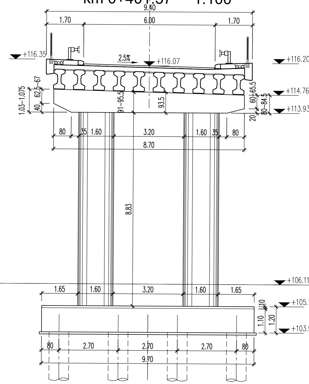
ПОПРЕЧНИ ПРЕСЕК СТУБА С7 CROSS SECTION C7 km 0+401.57 1:100
