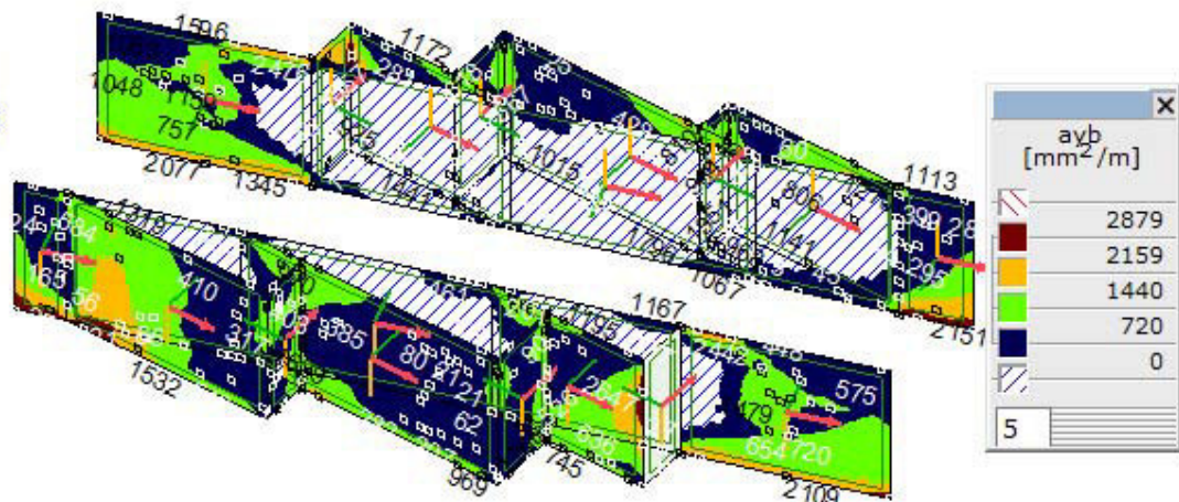
Кол. арм. - [R], > 2 parts, Линеарно,(Auto) Крум., аyb, Isosurfaces 2D
