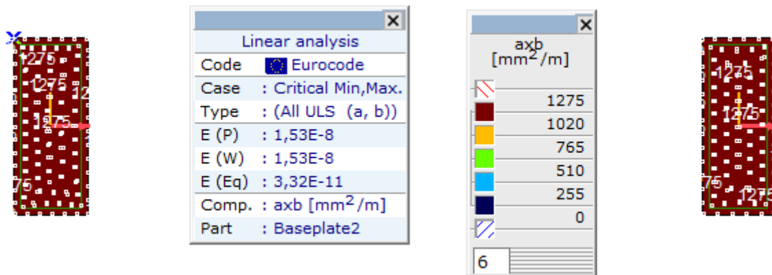
[RI], > Плоча, Линеарно,(Auto) Critical, axb, Isosurfaces 2D, Гоњрни поглед
