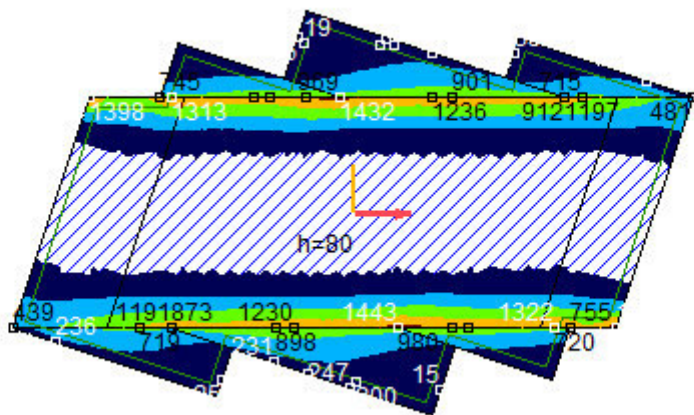
[I], > Палуба, Линеарно,(Auto) Крит. макс., myD+, Isosurfaces 2D, Горњи поглед
