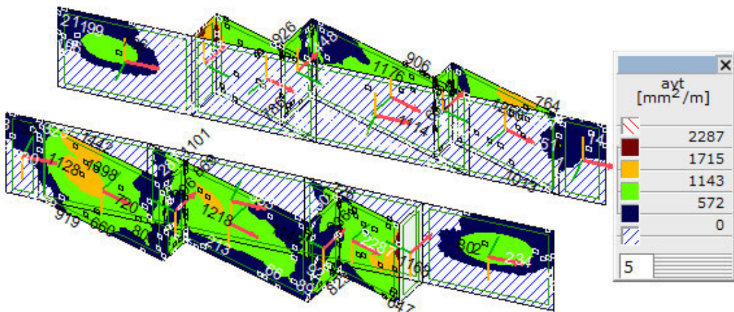
Кол. арм. - [R], > 2 parts, Линеарно,(Auto) Крум., аyt, Isosurfaces 2D
