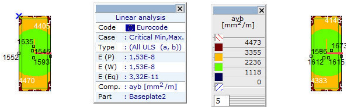
[RI], > Плоча, Линеарно,(Auto) Крит., ayb, Isosurfaces 2D, Горњи поглед
