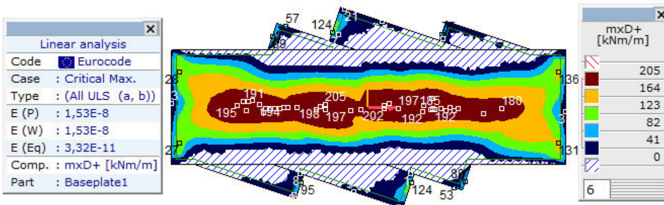
[[], > Плоча, Линеарно,(Auto) Крит. Max., mxD+, Isosurfaces 2D, Горњи поглед
