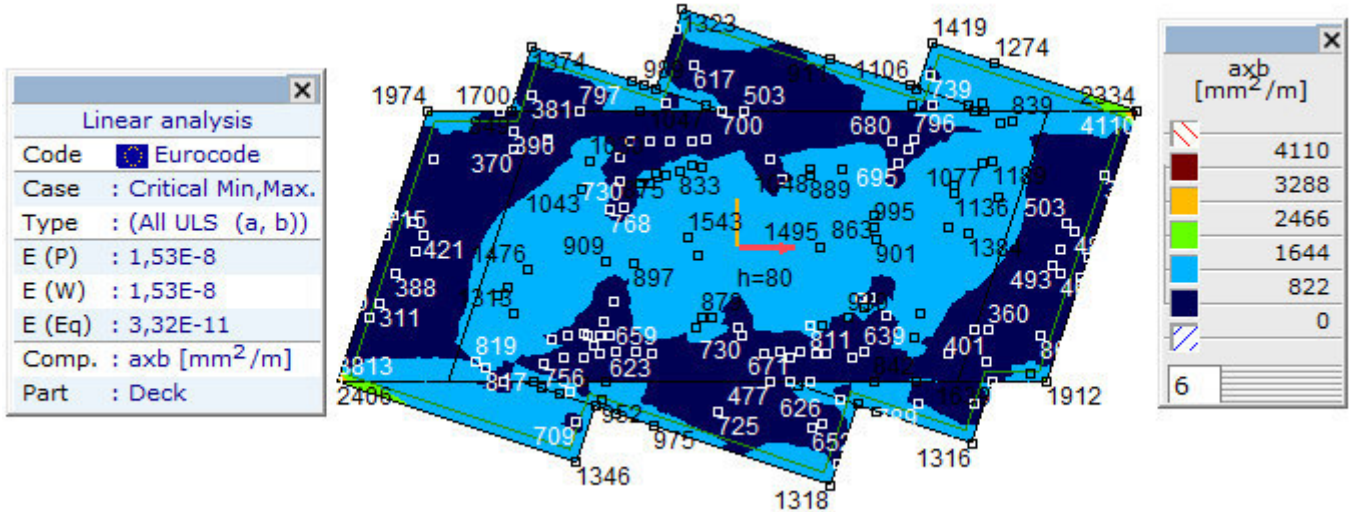
[RI], > Палуба, Линеарно,(Auto) Крм., axb, Isosurfaces 2D, Горњи поглед
