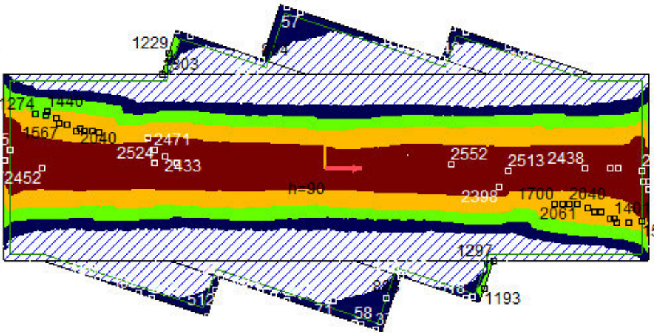
[RI], > Плоча, Линеарно,(Auto) Крм., ayt, Isosurfaces 2D, Горњи поглед
