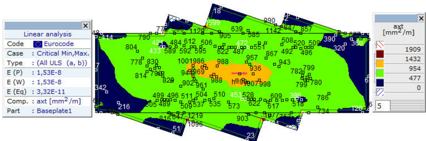
[RI], > Плоча, Линеарно,(Auto) Крит., axt, Isosurfaces 2D, Горњи поглед
