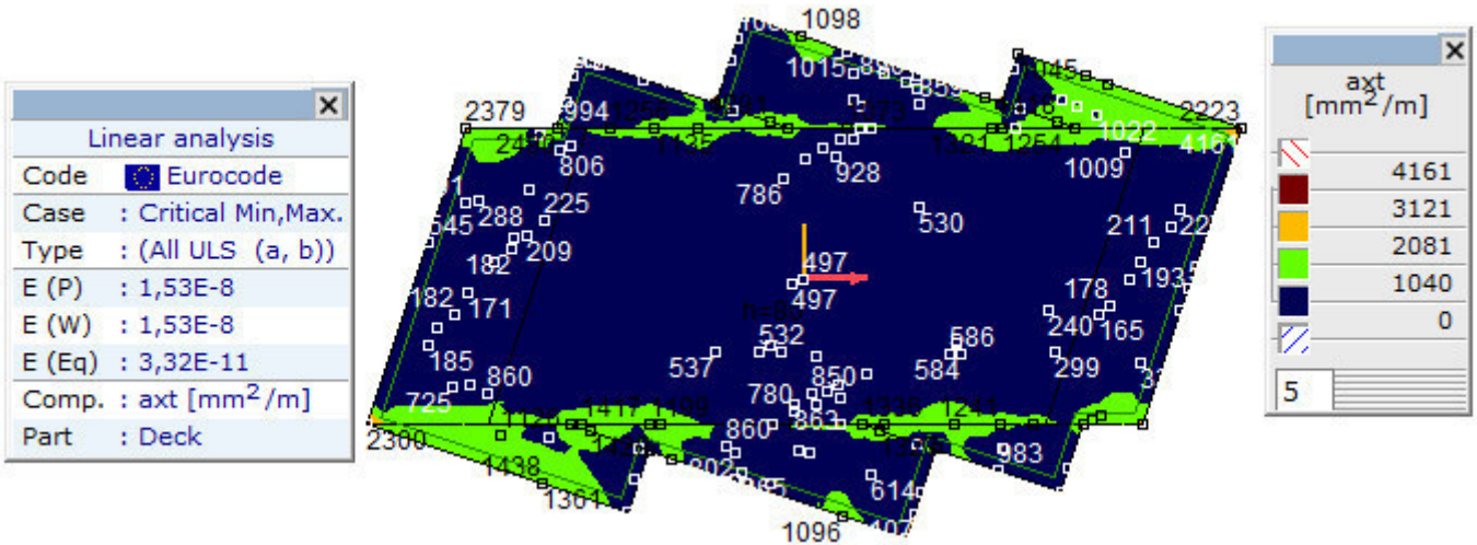
[RI], > Палуба, Линеарно,(Auto) Крм., axt, Isosurfaces 2D, Горњи поглед
