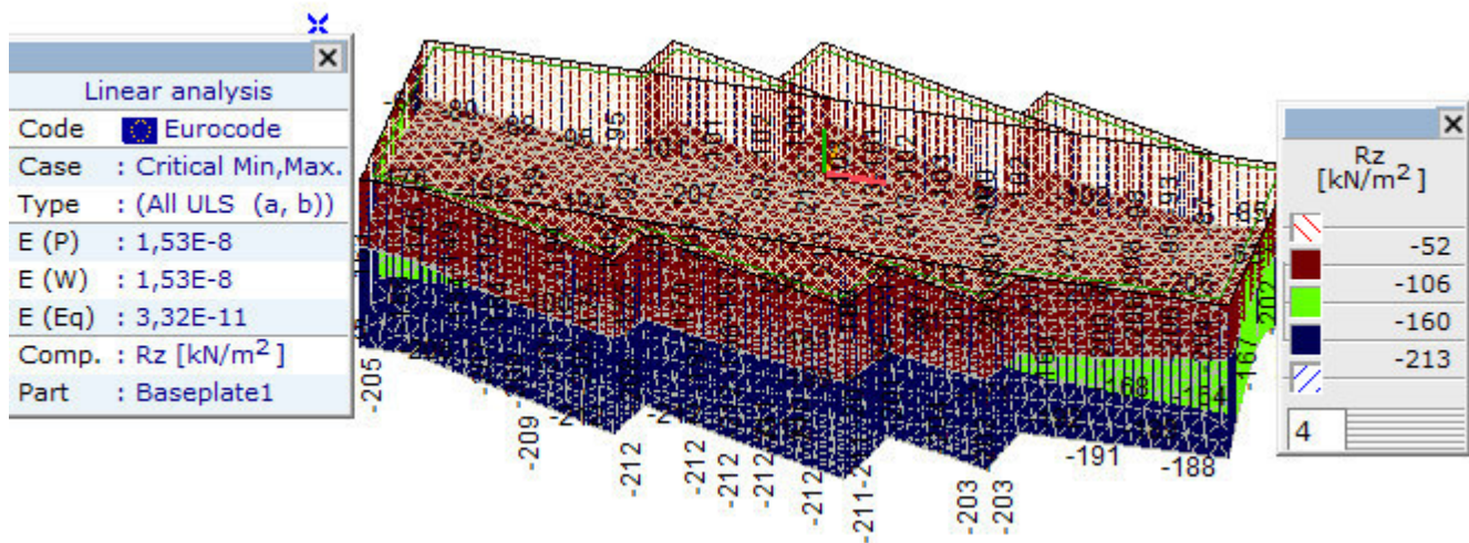
[I], Линеарно,(SLS Квази-стално) Крит. мин..., Rz (surf. supp.), Isosurfaces 3D
