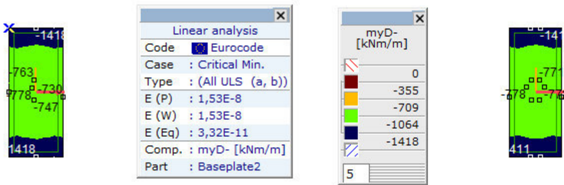
[I], > Плоча, Линеарно,(Auto) Крит. мин., myD-, Isosurfaces 2D, Горњи поглед
