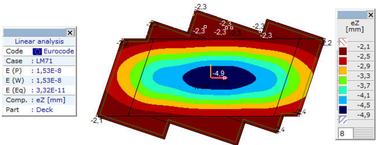
[[], > Палуба, Линеарно,(SLS Characteristic) Крит. мин., eZ, Isosurfaces 2D, Горњи поглед
