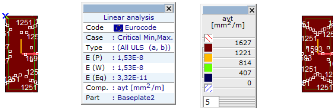
[RI], > Плоча, Линеарно,(Auto) Крит., ayt, Isosurfaces 2D, Горњи поглед
