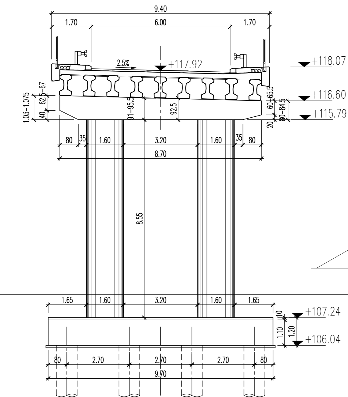
OSNOVNA ТЕЛО С3 BASE 1:100
