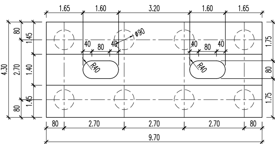
OSNOVNA ТЕЛО С3 BASE 1:100
