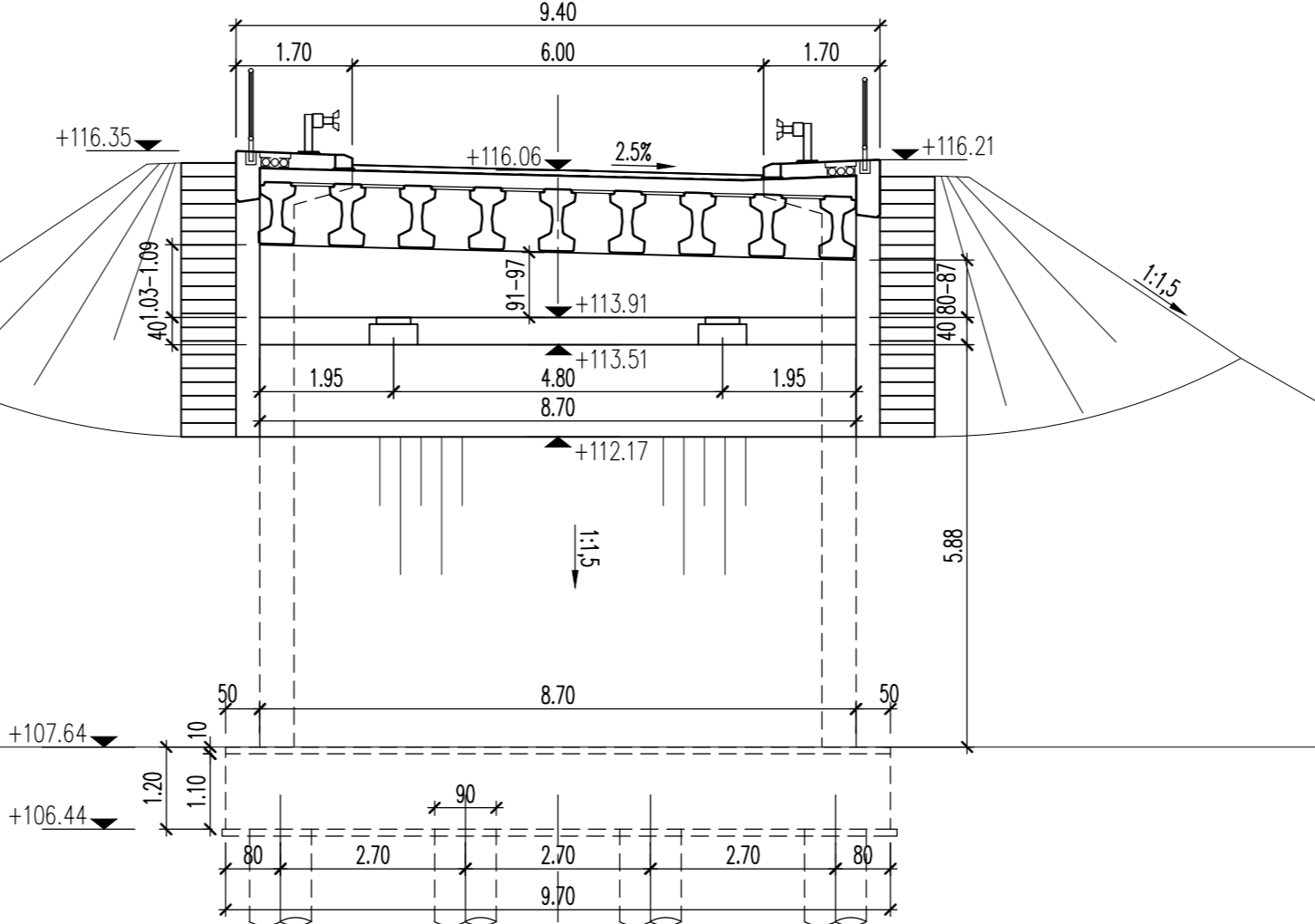
ПОПРЕЧНИ ПРЕСЕК СТУБА С8 CROSS SECTION С8 km 0+479.76 1:100
