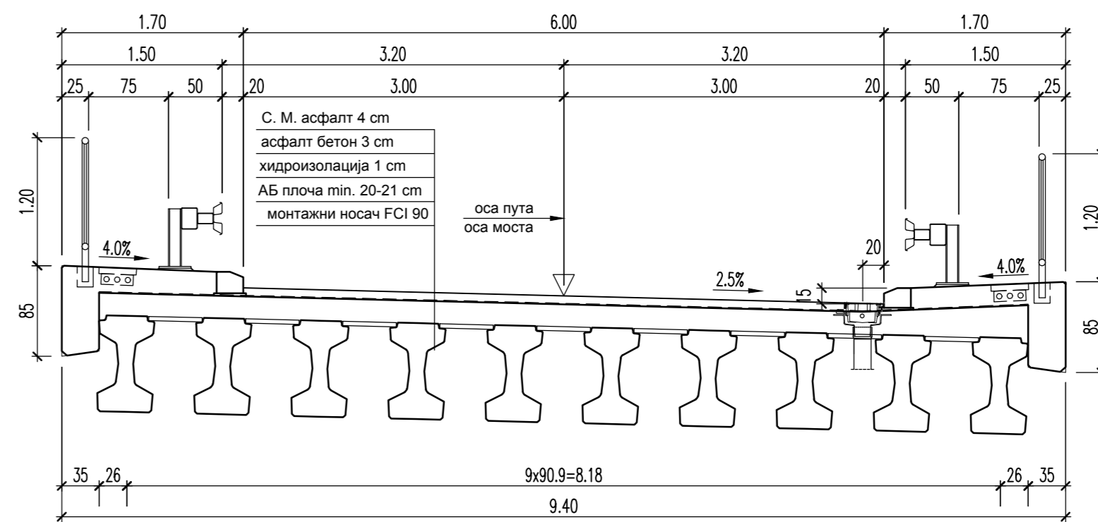
КАРАКТЕРИСТИЧНИ ПОПРЕЧНИ ПРЕСЕЦИ НАДВОЖЊАКА GENERAL CROSS SECTION 1:50
