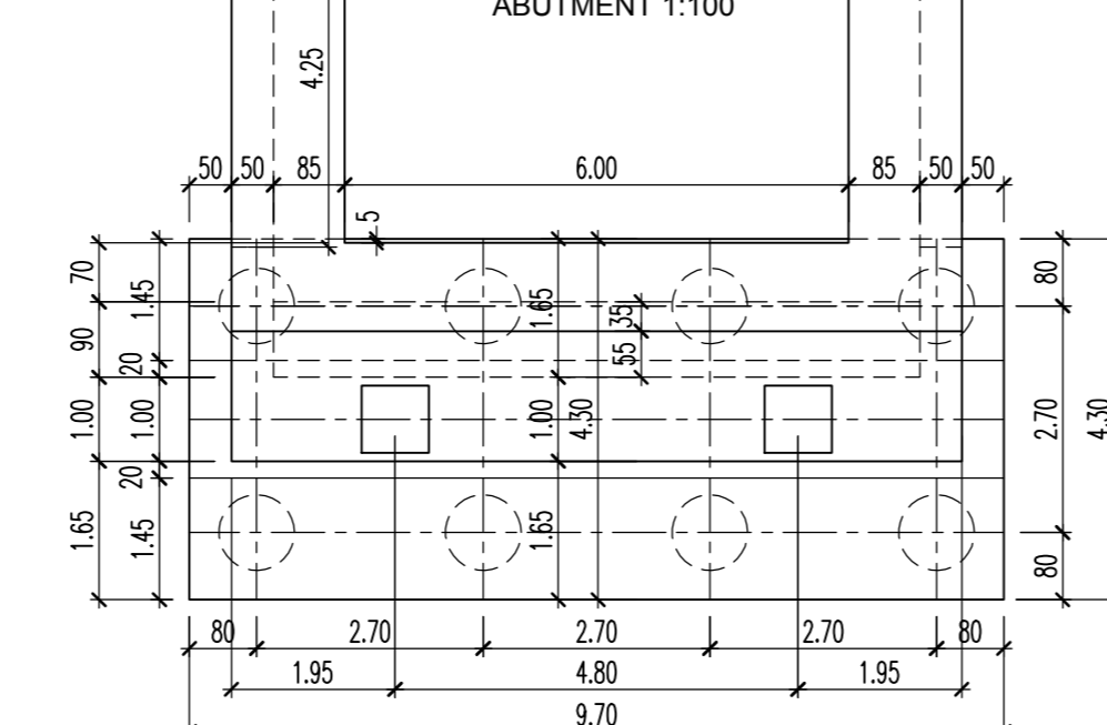
ОСНОВНО ТЕЛО С6 ABUTMENT 1:100
