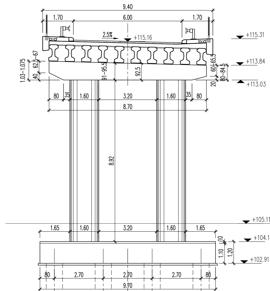
ПОПРЕЧНИ ПРЕСЕК СТУБА С3 CROSS SECTION C3 KM 0+200.59 1:100
