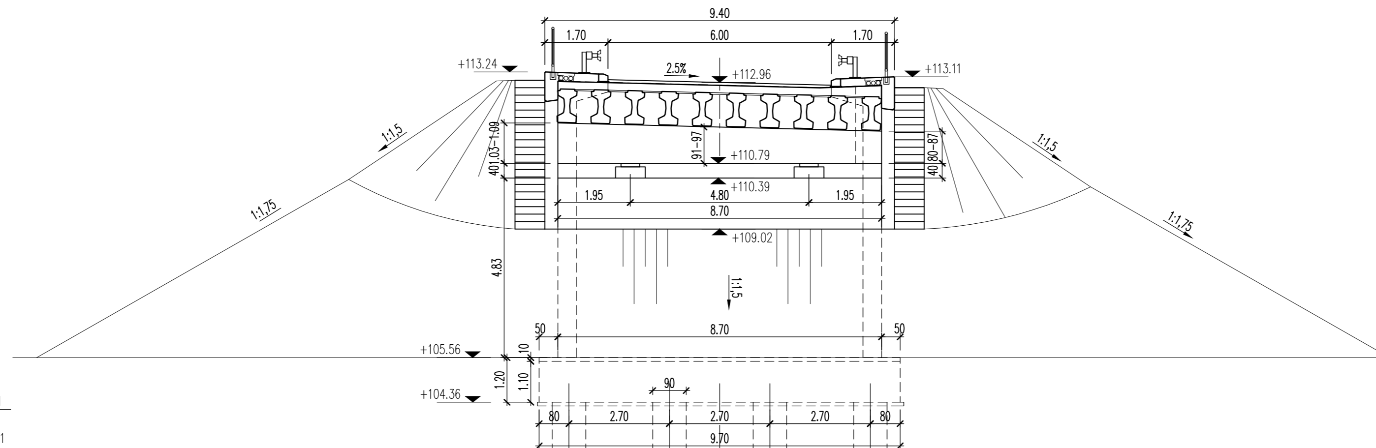
ПОПРЕЧНИ ПРЕСЕК СТУБА С6 CROSS SECTION C6 KM 0+264.09 1:100
