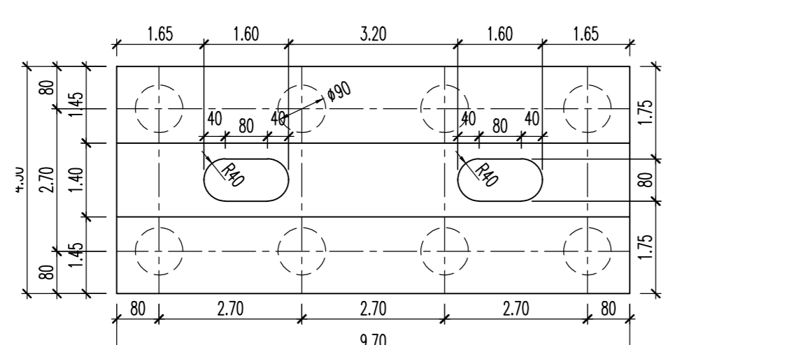
OSNOVNA TELU C3 BASE 1:100
