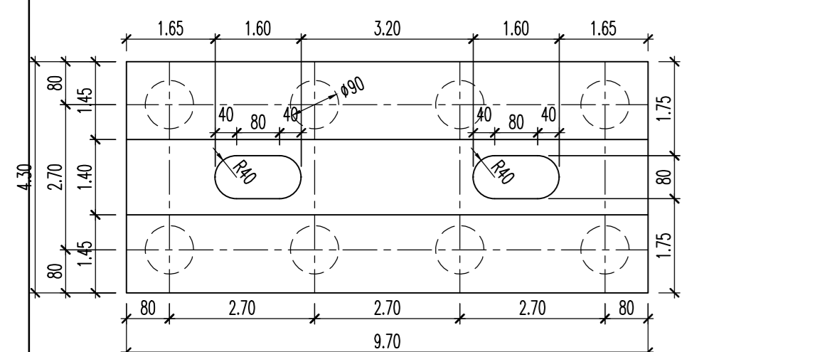
OSNOVNA TELU C2 BASE 1:100
