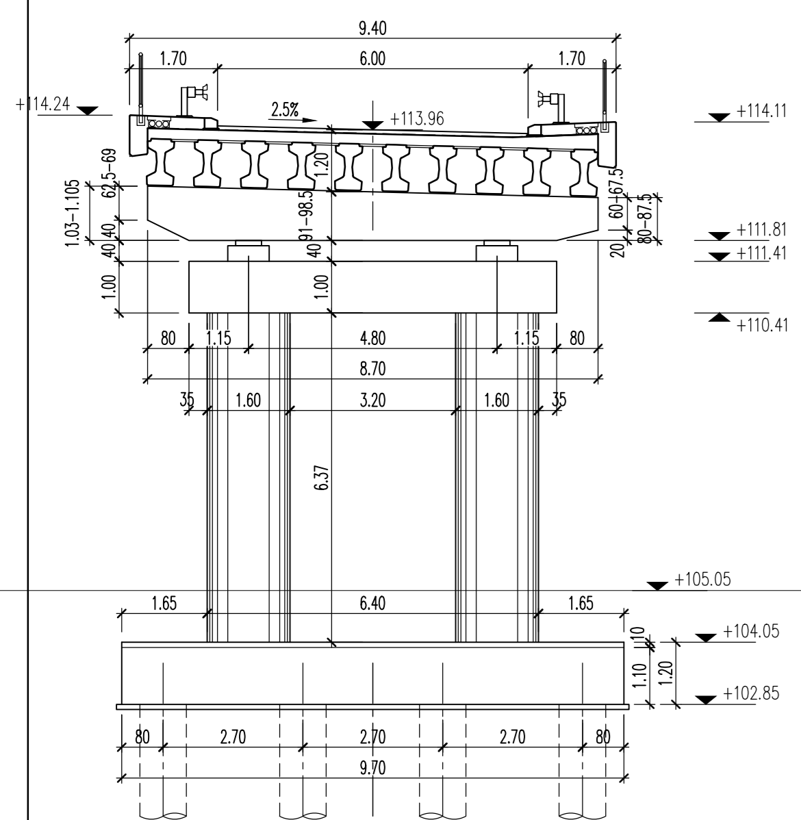
OSNOVNA TELU C2 BASE 1:100
