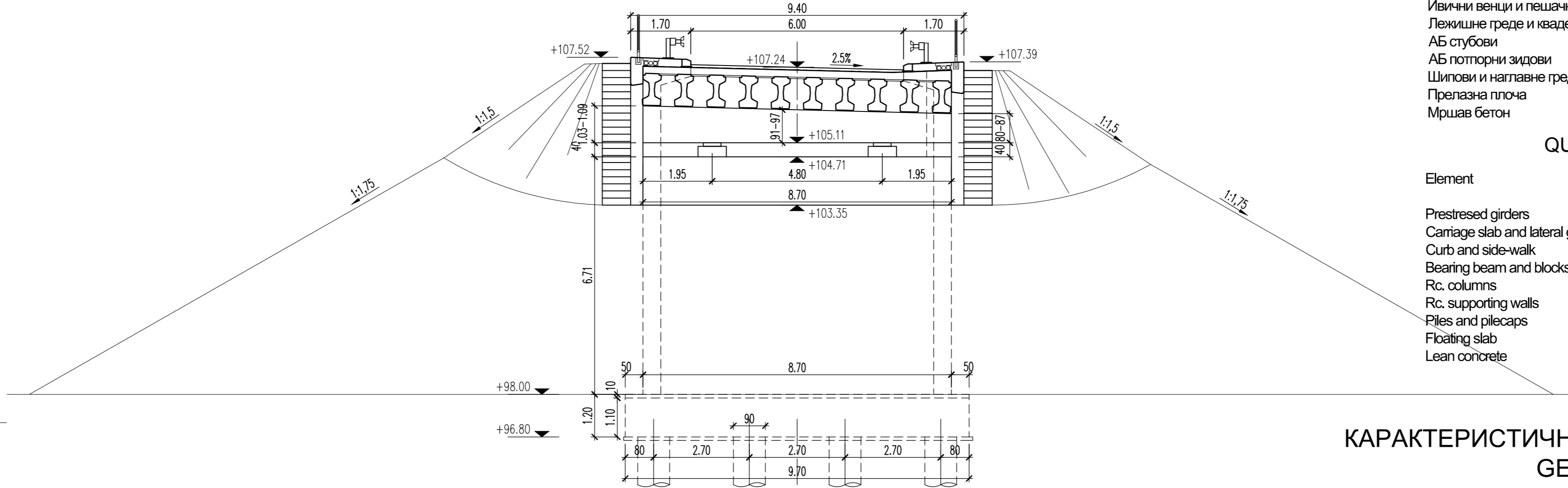
OSNOVNA ТЕЛО С6 ABUTMENT 1:100
