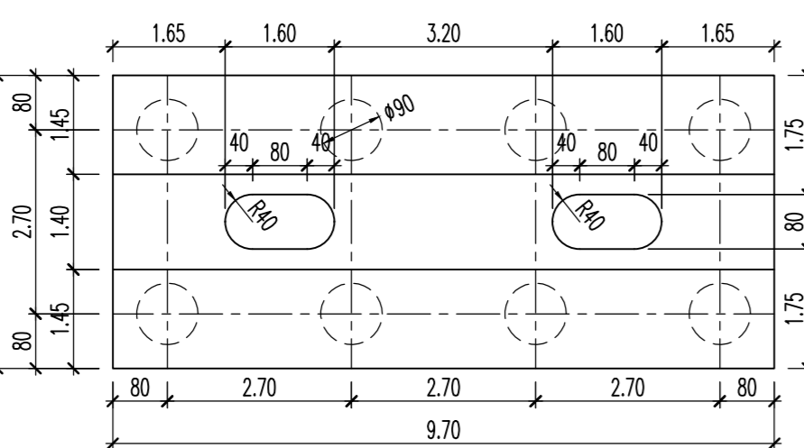
OSNOVNA ТЕЛО С3 BASE 1:100
