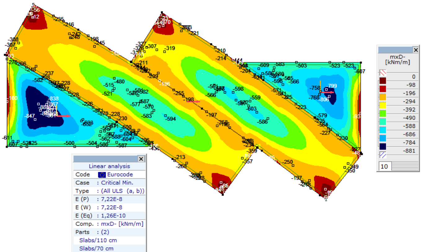
Линеарно,(Auto) Крит. Мин., mxD-, Isosurfaces 2D, Горњи поглед
