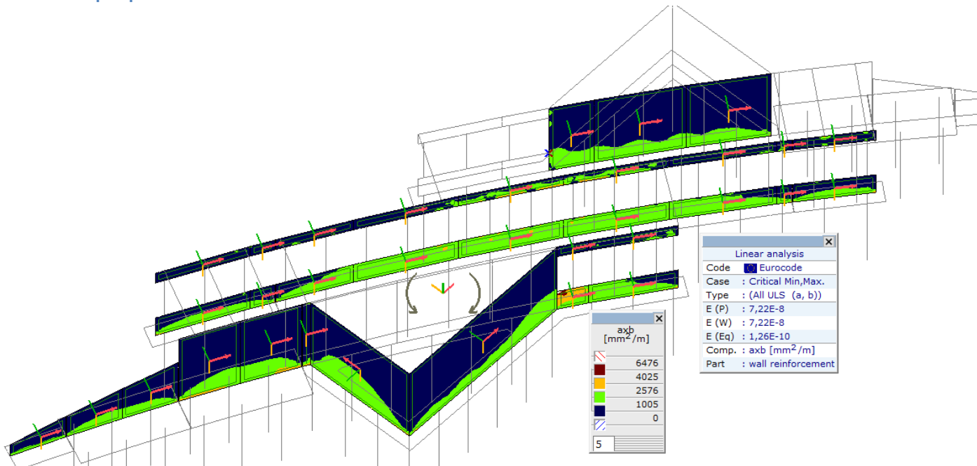
Линеарно, (Auto) Крм., axb, Isosurfaces 2D
