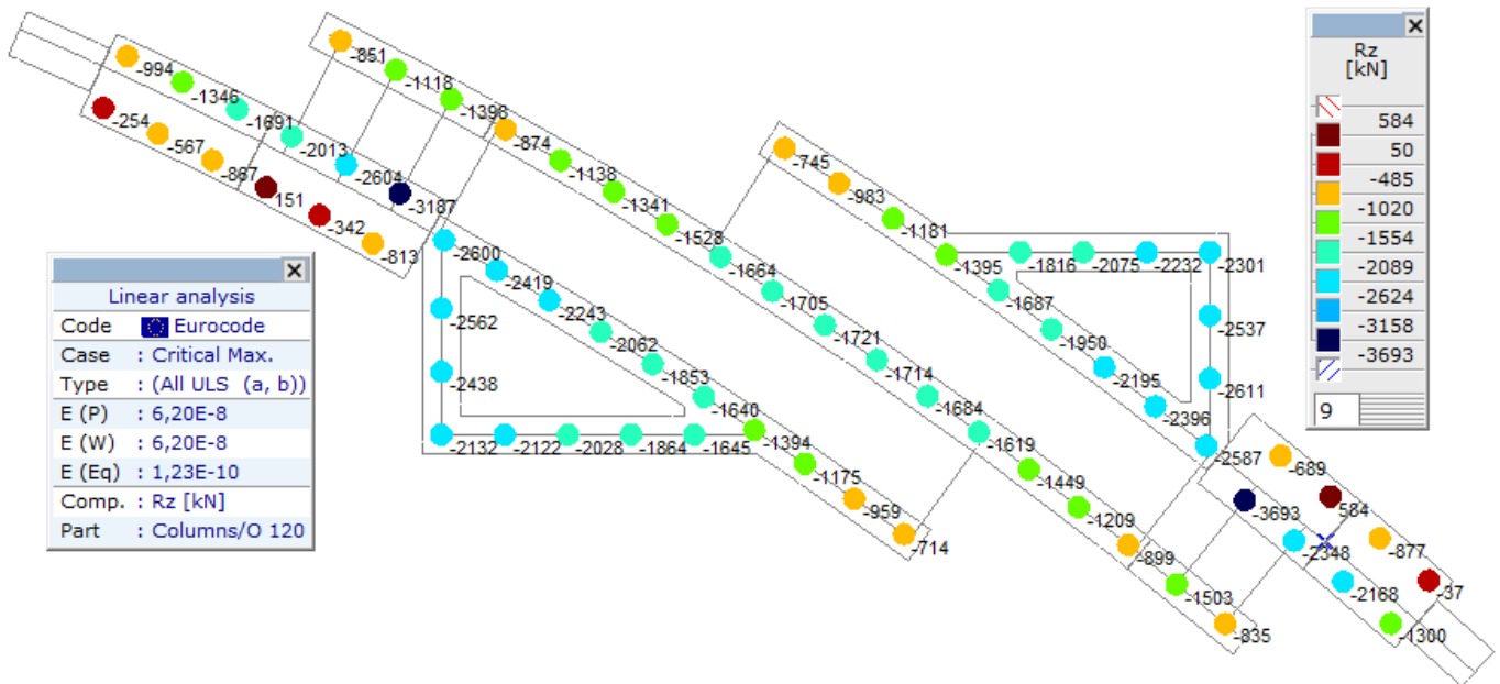
Линеарно,(Auto) Крит. Мах., Rz (зглобни осл.), Isosurfaces 2D, Горњи поглед
