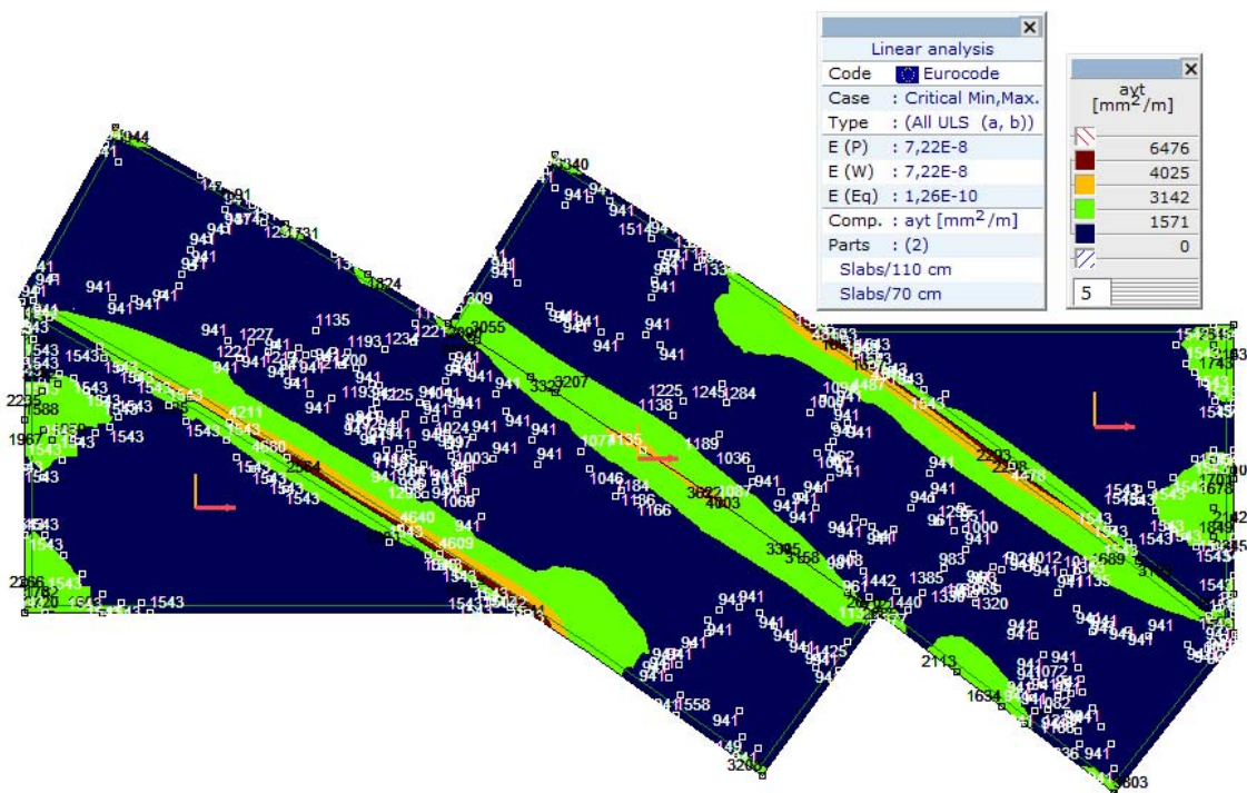
Линеарно,(Auto) Крит., ayt, Isosurfaces 2D, Горњи поглед
