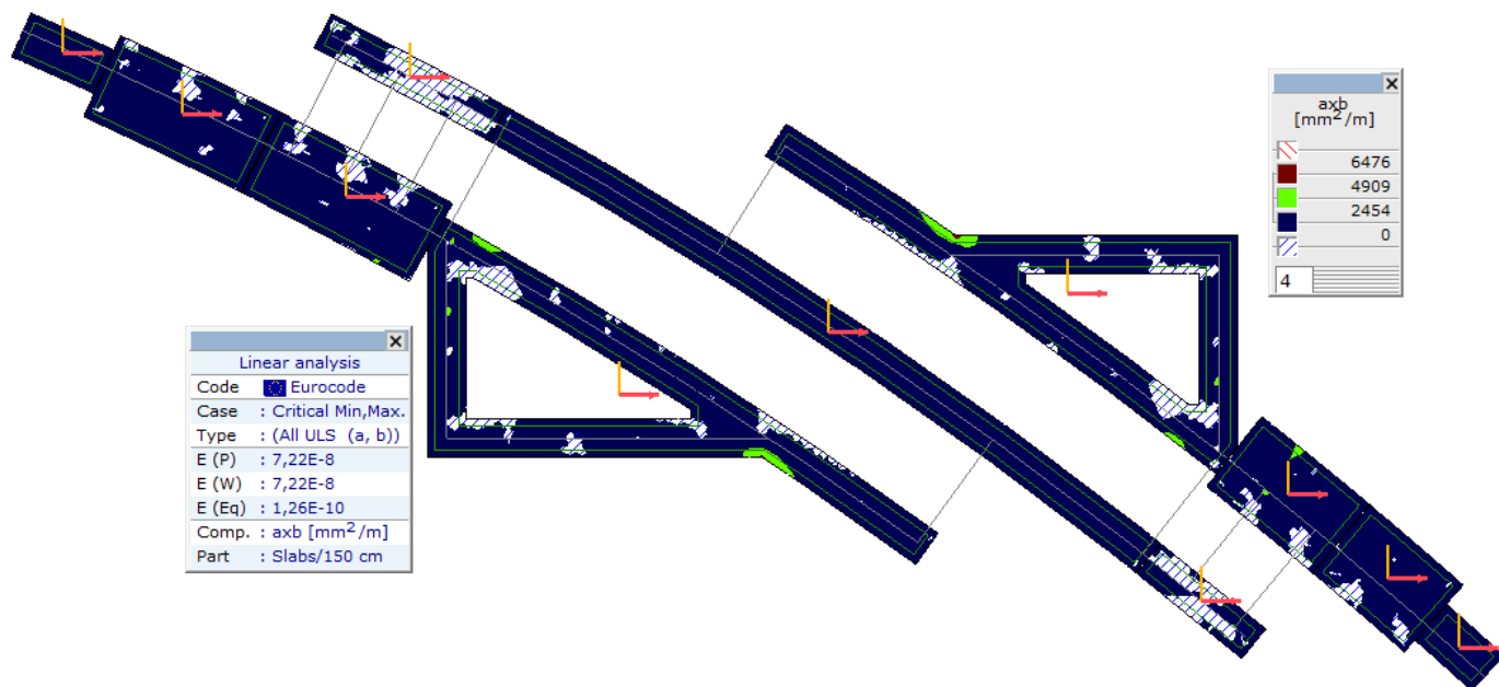
Линеарно, (Auto) Критично, axb, Isosurfaces 2D, Горњи поглед
