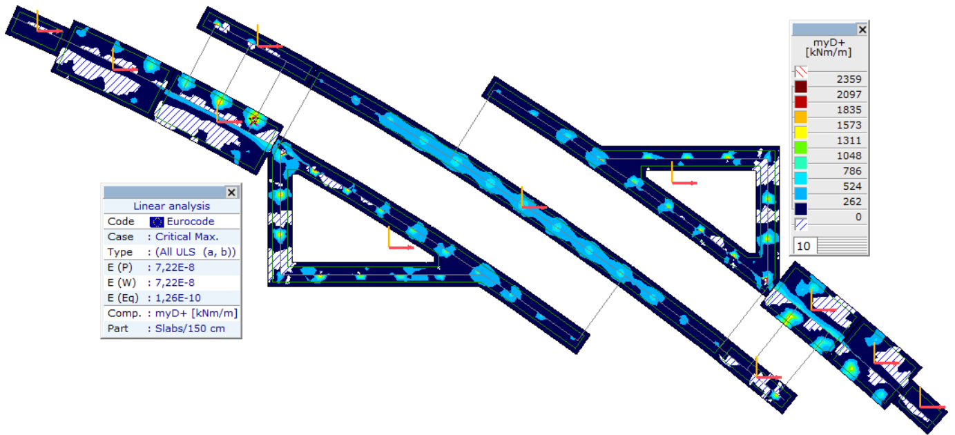
Линеарно,(Auto) Критично Мах., myD+, Isosurfaces 2D, Горњи поглед
