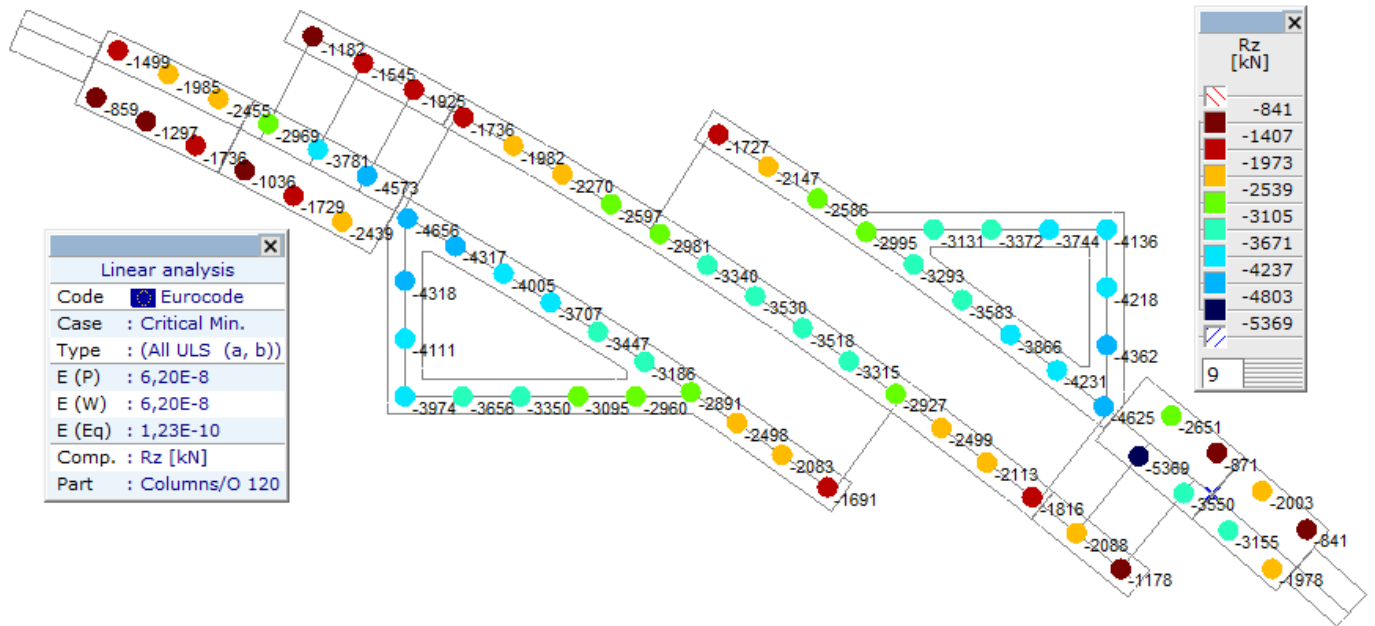
Линеарно,(Auto) Критично Мин., Rz (зглобни осл.), Isosurfaces 2D, Горњи поглед
