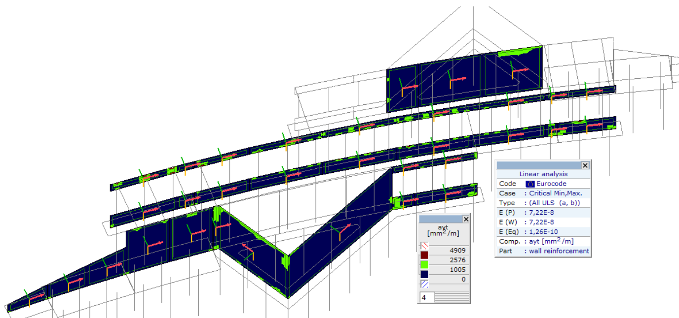
Линеарно,(Auto) Крив., ayt, Isosurfaces 2D
