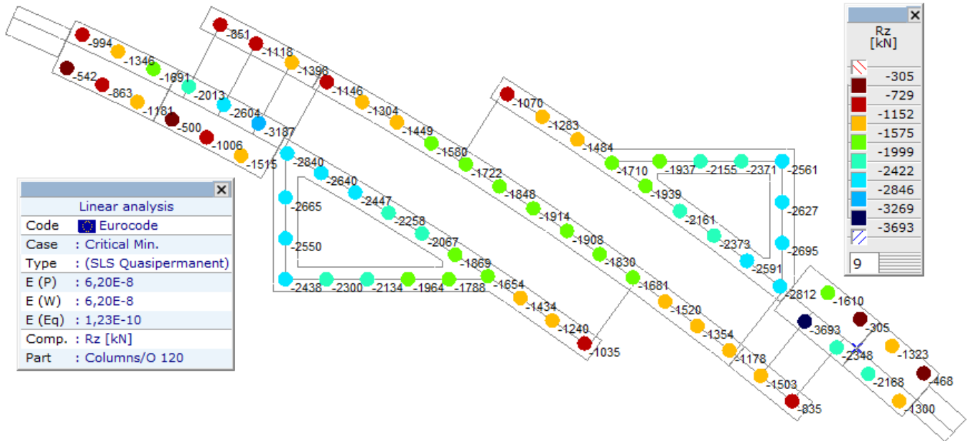
Линеарно,(ГСУ Квази-стално) Крит. мин., Rz (зглобни осл.), Isosurfaces 2D, Горњи поглед
