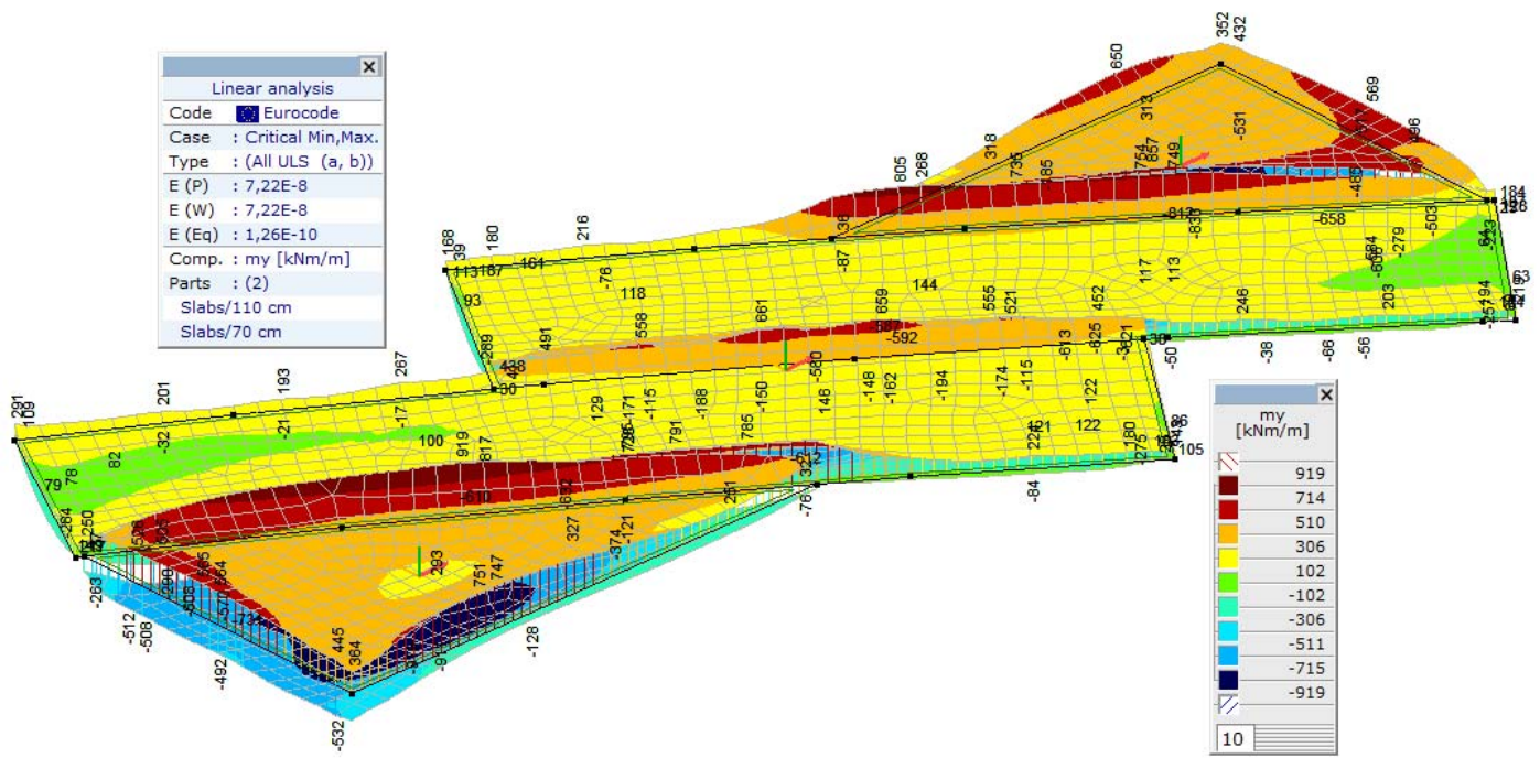
Линеарно,(Auto) Крум., my, Isosurfaces 3D
