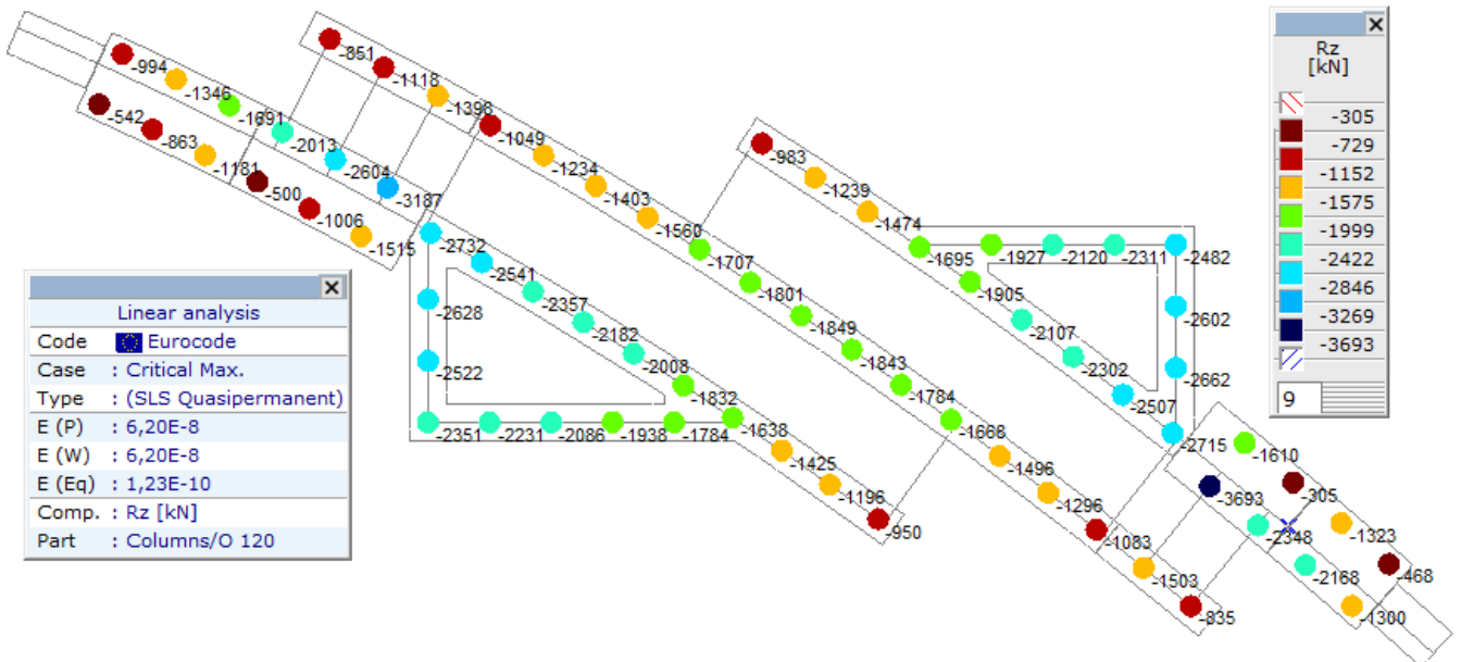
Линеарно,(ГСУ Квази-стално) Крит. Мах., Rz (зглобни осл.), Isosurfaces 2D, Горњи поглед
