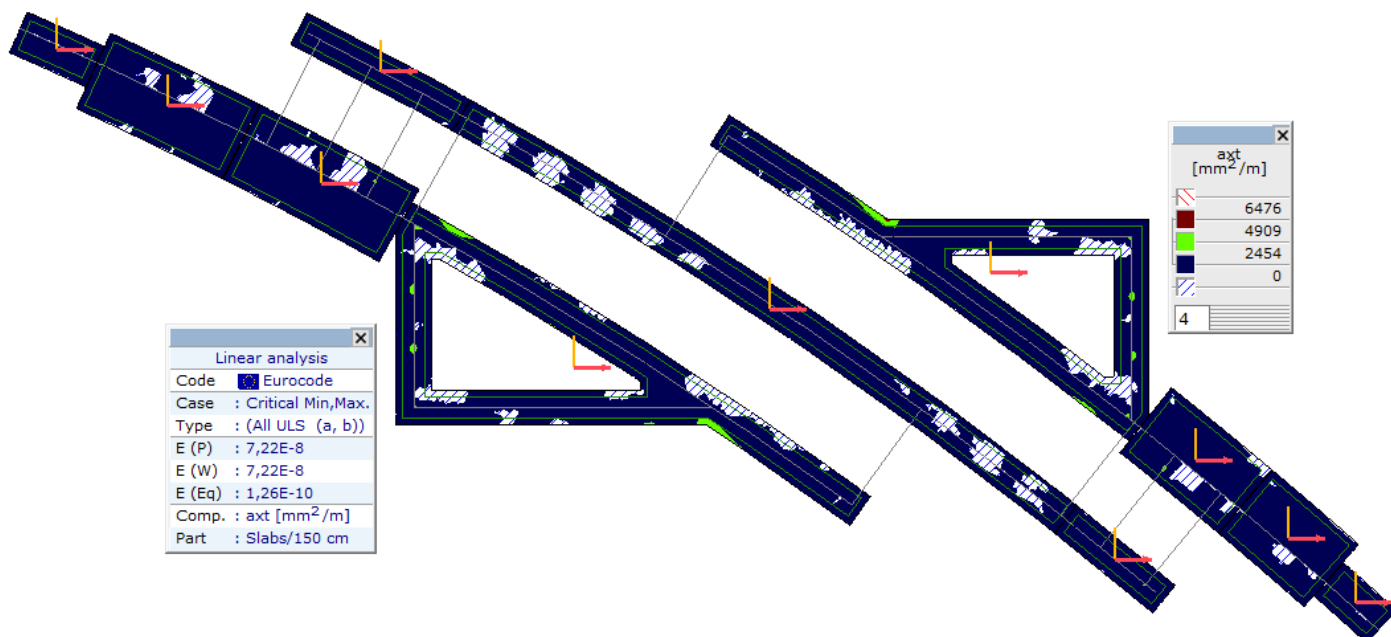
Линеарно, (Auto) Критично, axt, Isosurfaces 2D, Горњи поглед
