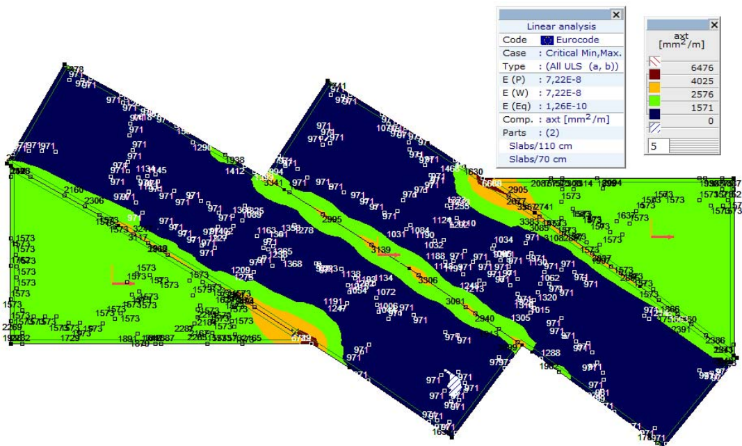
Линеарно,(Auto) Крит., axt, Isosurfaces 2D, Горњи поглед
