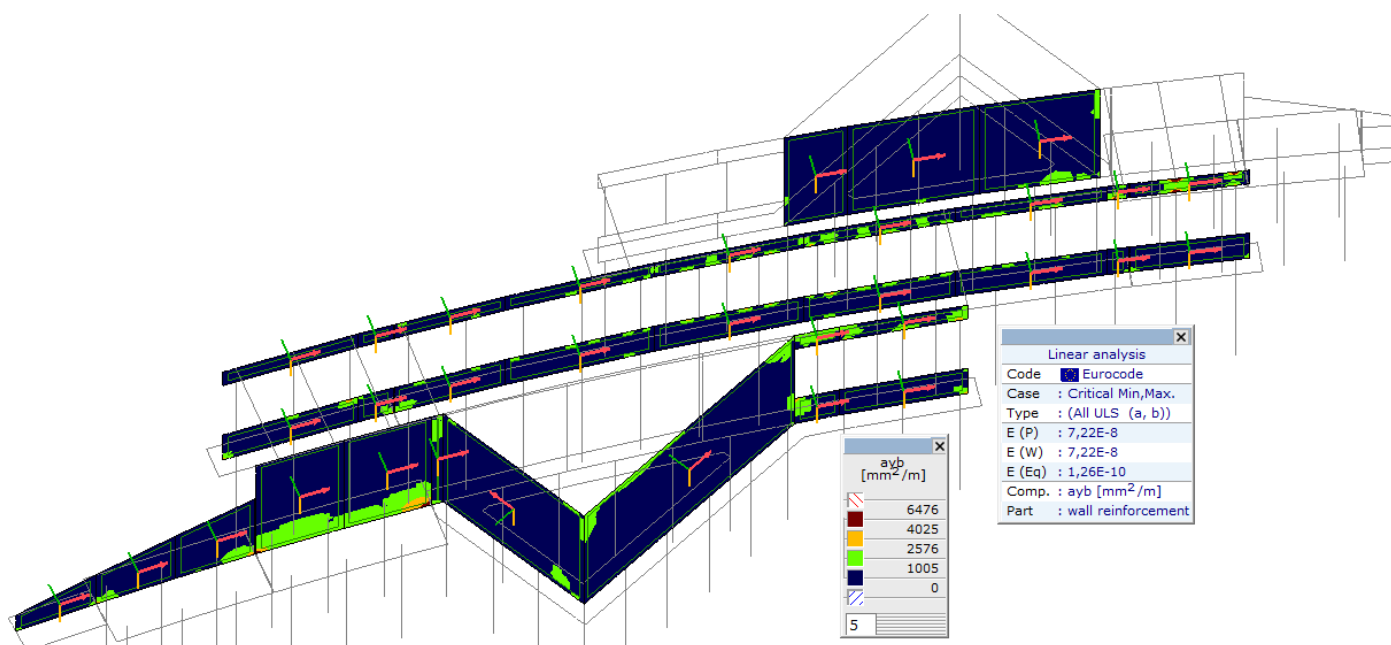
Линеарно,(Auto) Крив., ayb, Isosurfaces 2D
