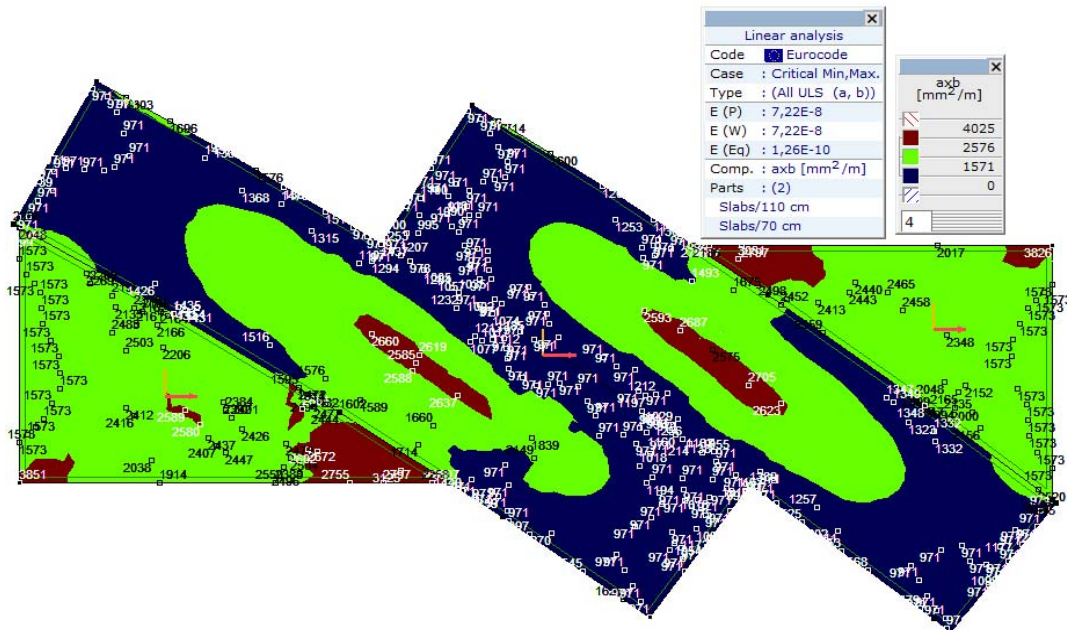
Линеарно,(Auto) Крит., axb, Isosurfaces 2D, Горњи поглед
