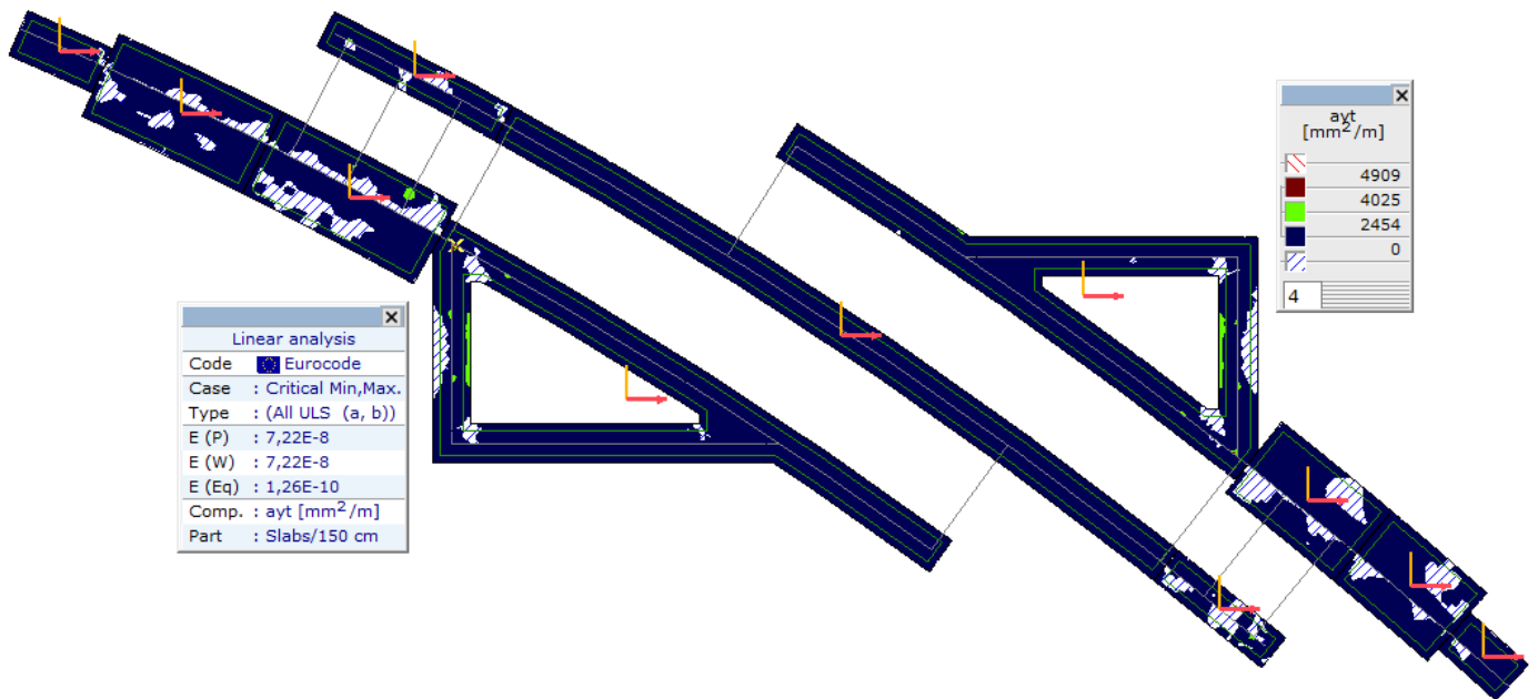
[R], > Плоча, Линеарно,(Auto) Критично, ayt, Isosurfaces 2D, Горњи поглед
