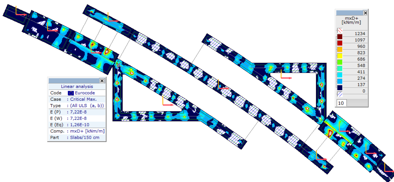
Линеарно,(Auto) Критично мах., mxD+, Isosurfaces 2D, Горњи поглед
