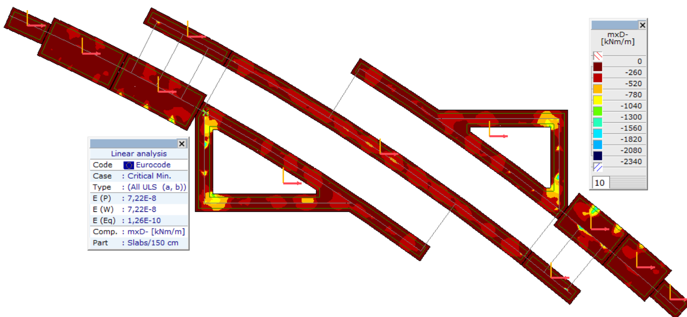
Линеарно,(Auto) Критично Мин., mxD-, Isosurfaces 2D, Горњи поглед
