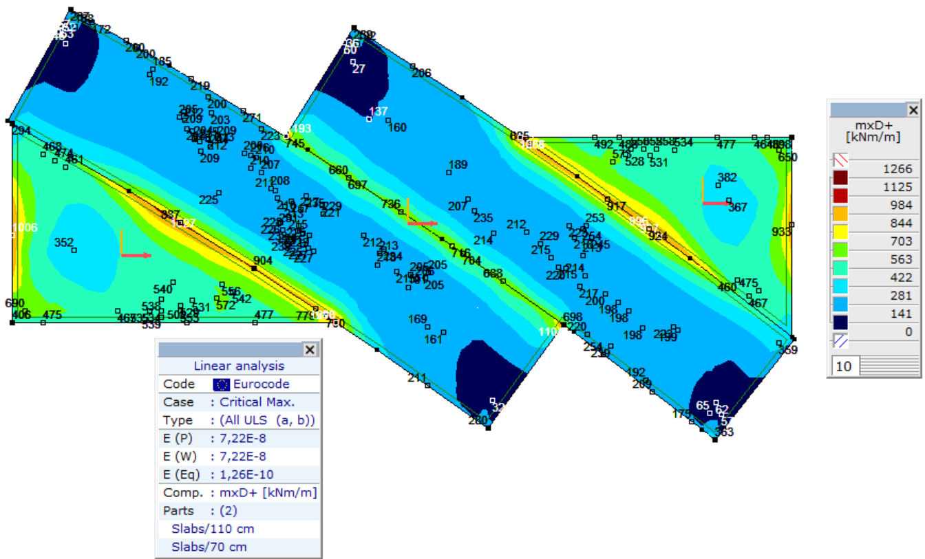
Линеарно,(Auto) Крит. Мах., mxD+, Isosurfaces 2D, Горњи поглед
