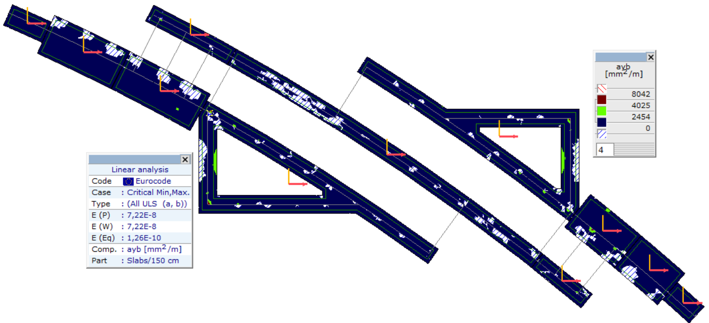
Линеарно,(Auto) Критично, ayb, Isosurfaces 2D, Горњи поглед
