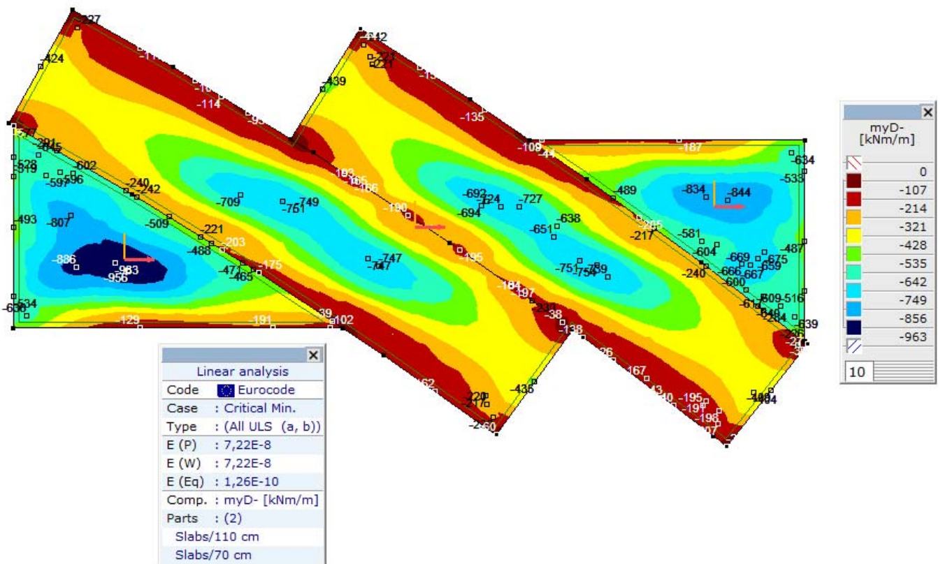
Линеарно,(Auto) Крит. Мин., myD-, Isosurfaces 2D, Горњи поглед
