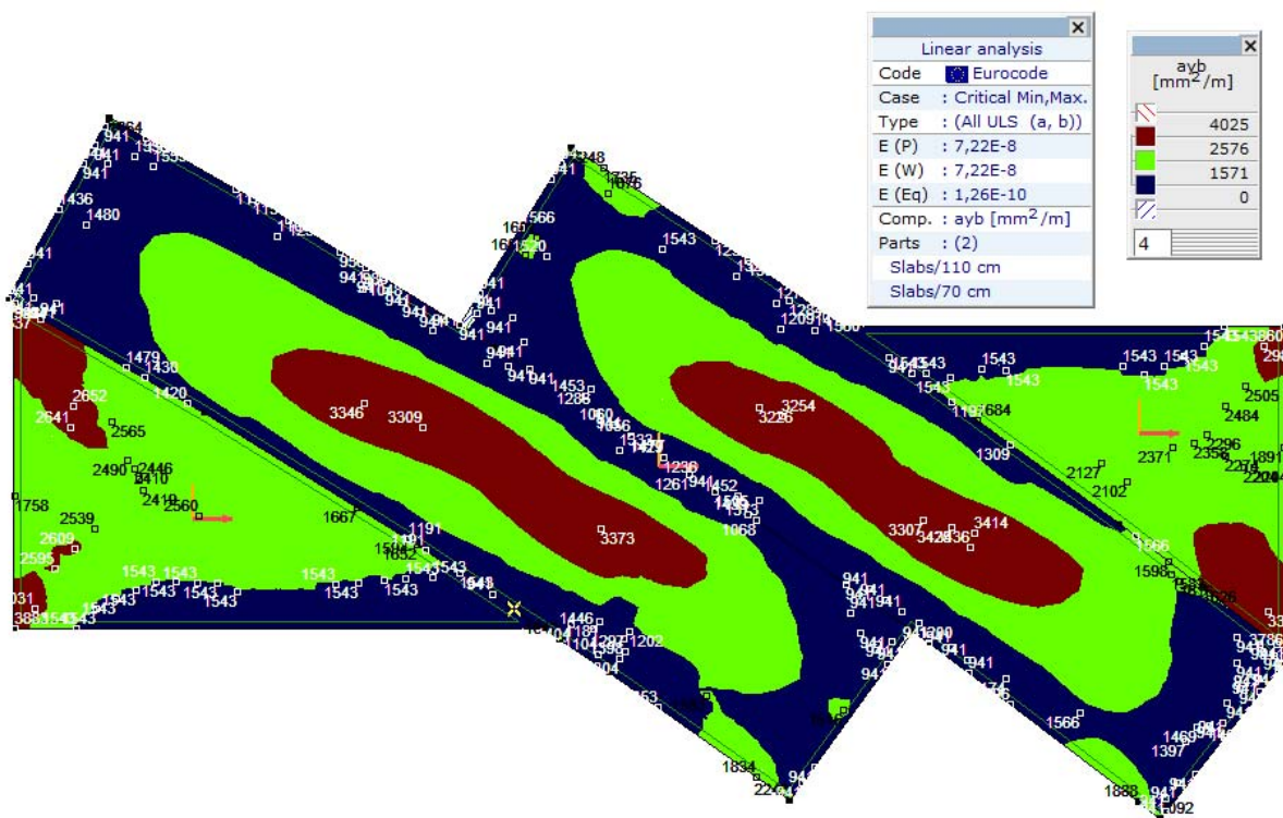
Линеарно,(Auto) Критично, ayb, Isosurfaces 2D, Горњи поглед
