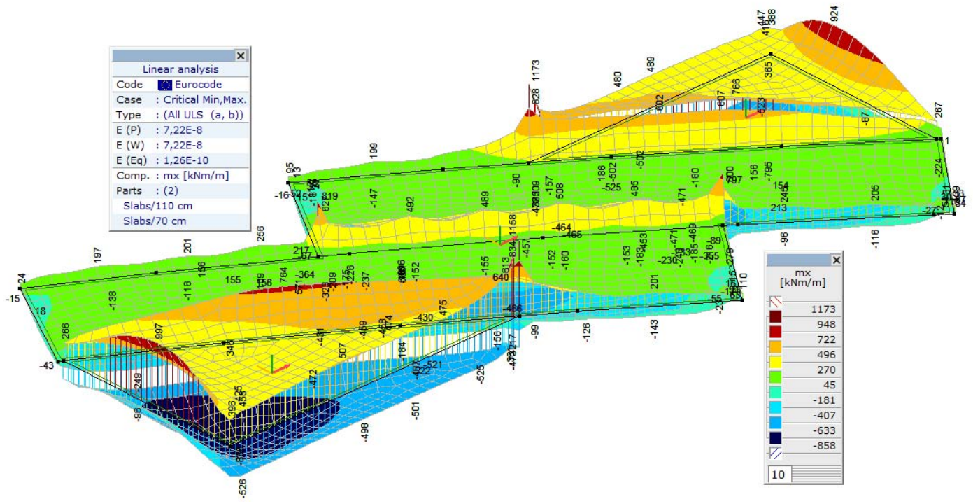
Линеарно,(Auto) Крум., mx, Isosurfaces 3D
