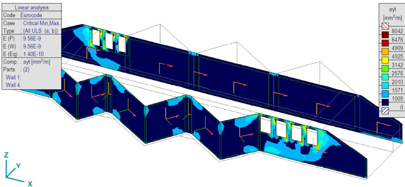
Кол. арм.- [Rl], > 2 parts, Линеарно,(Auto) Крив., ayt, Isosurfaces 2D
