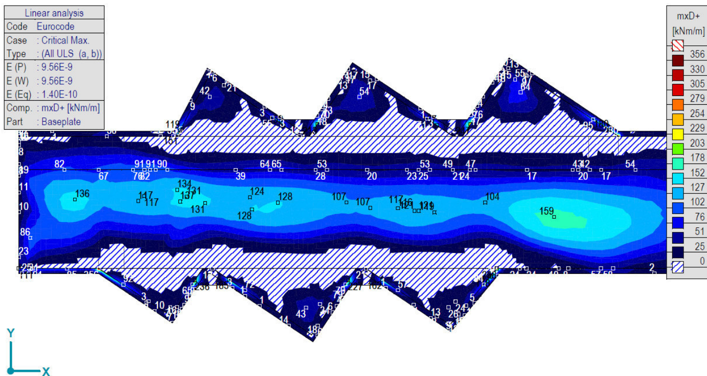
[[I], > Плоча, Линеарно,(Auto) Крит. Max., mxD+, Isosurfaces 2D, Горњи поглед
