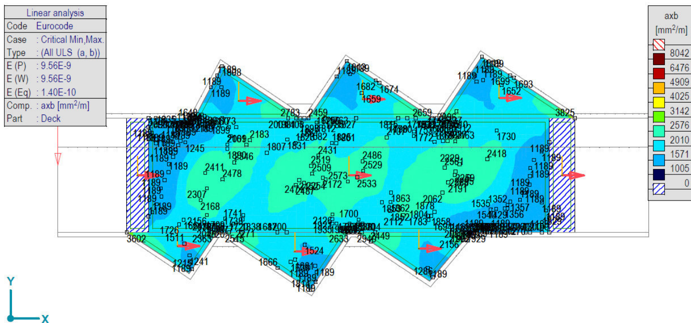
[R], > Палуба, Линеарно,(Auto) Крит., axb, Isosurfaces 2D, Горњи поглед
