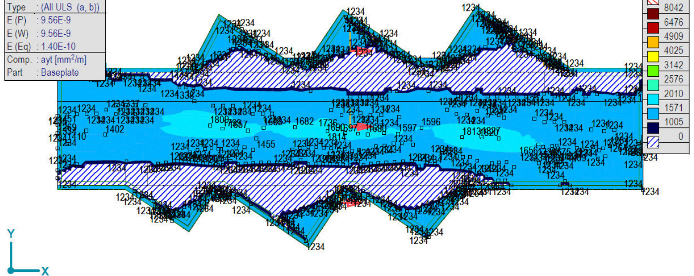
[RI], > Плоча, Линеарно,(Auto) Крит., ayt, Isosurfaces 2D, Горњи поглед
