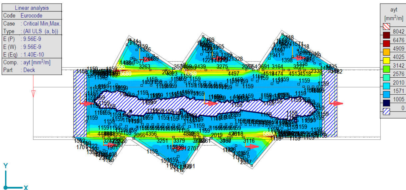
[R], > Палуба, Линеарно,(Auto) Крит., ayt, Isosurfaces 2D, Горњи поглед
