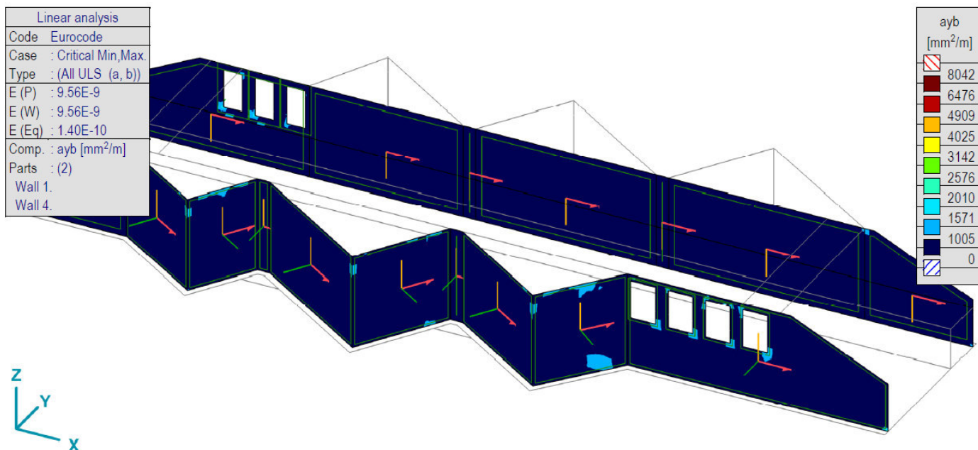
Кол. арм.- [Rl], > 2 parts, Линеарно,(Auto) Крив., ayb, Isosurfaces 2D
