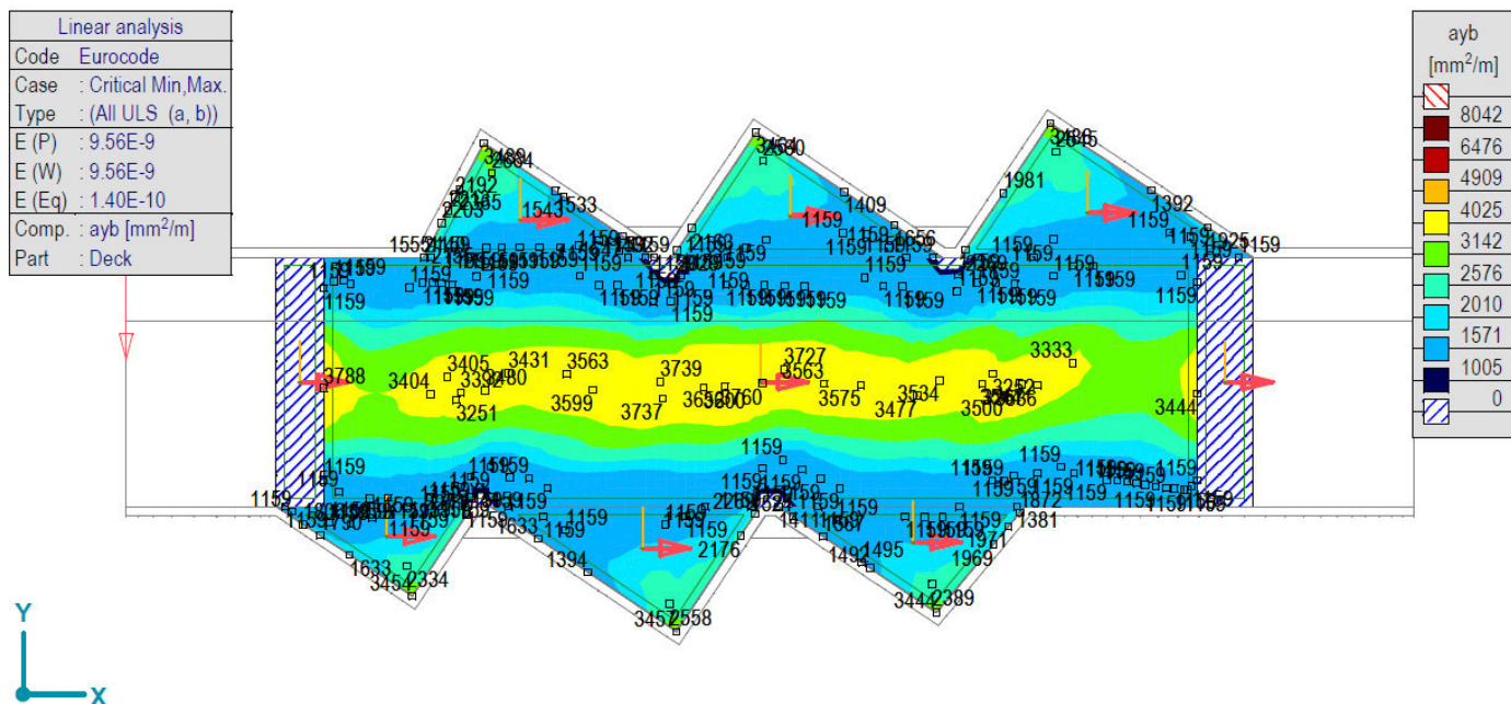
[R], > Палуба, Линеарно,(Auto) Крит., ayb, Isosurfaces 2D, Горњи поглед
