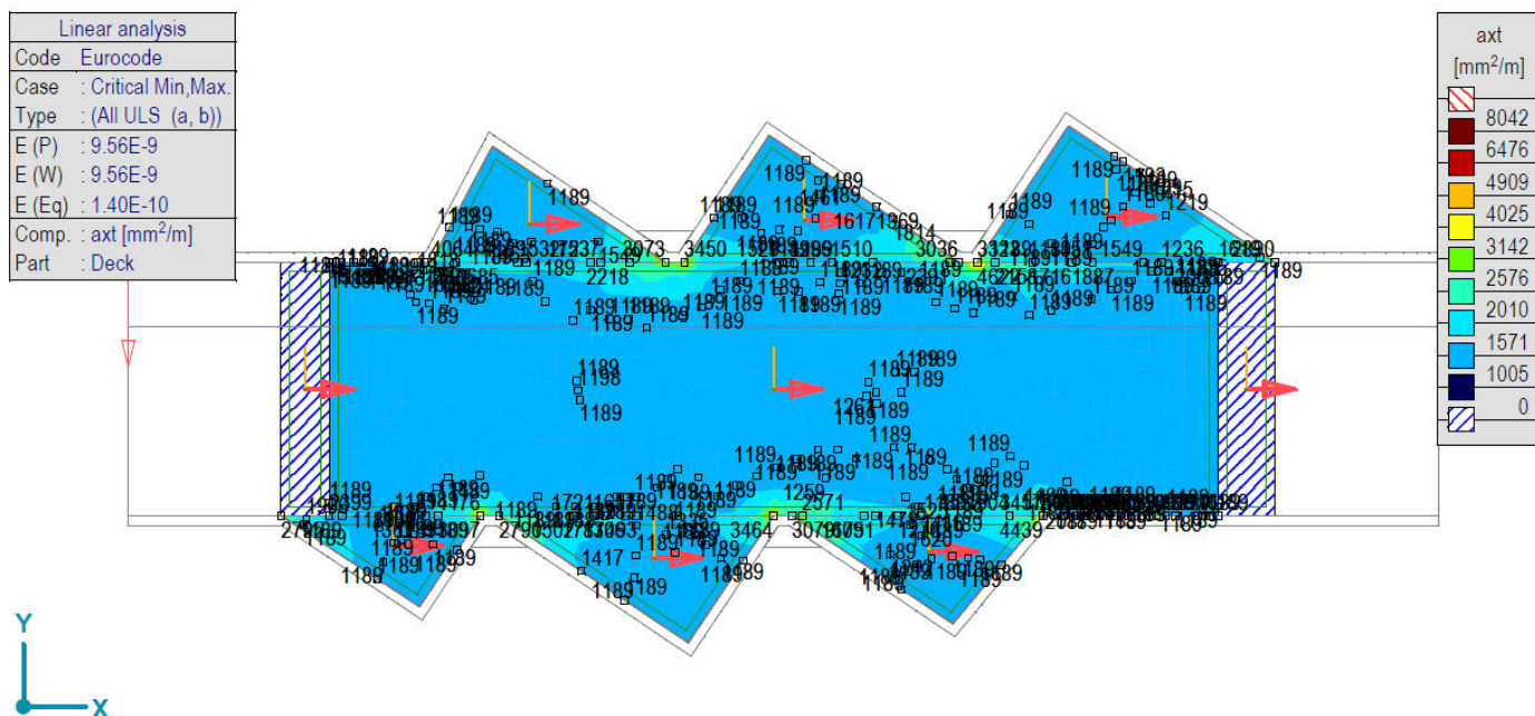
[R], > Палуба, Линеарно,(Auto) Крит., axt, Isosurfaces 2D, Горњи поглед
