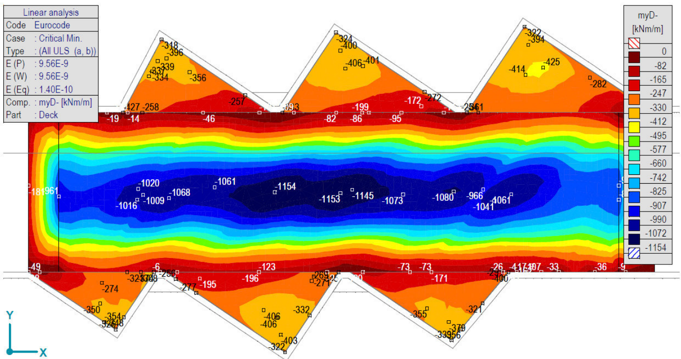
[I], > Палуба, Линеарно, (Auto) Крит. мин., myD-, Isosurfaces 2D, Горњи поглед
