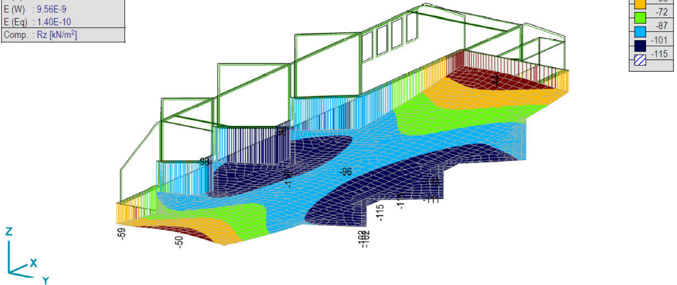
[I], Линеарно,(SLS Квази-стално) Крит. мин..., Rz (surf. supp.), Isosurfaces 3D
