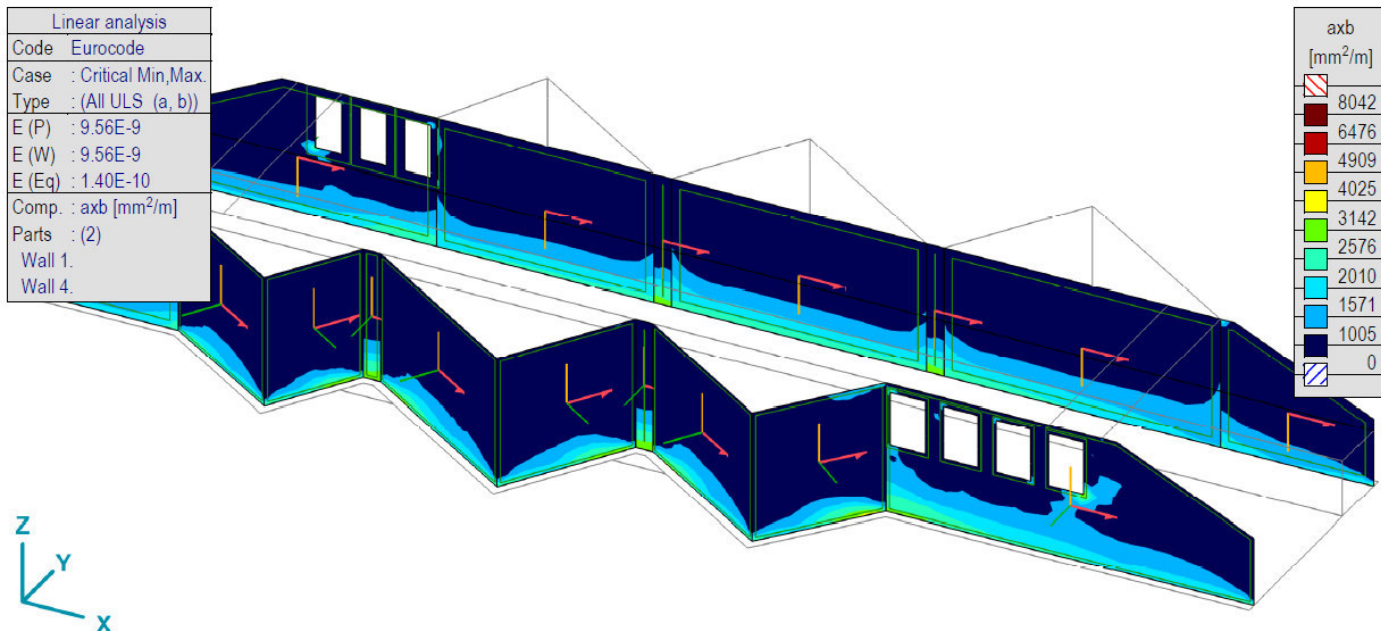
Кол. арм. - [RI], > 2 дела, Линеарно, (Auto) Крм., axb, Isosurfaces 2D
