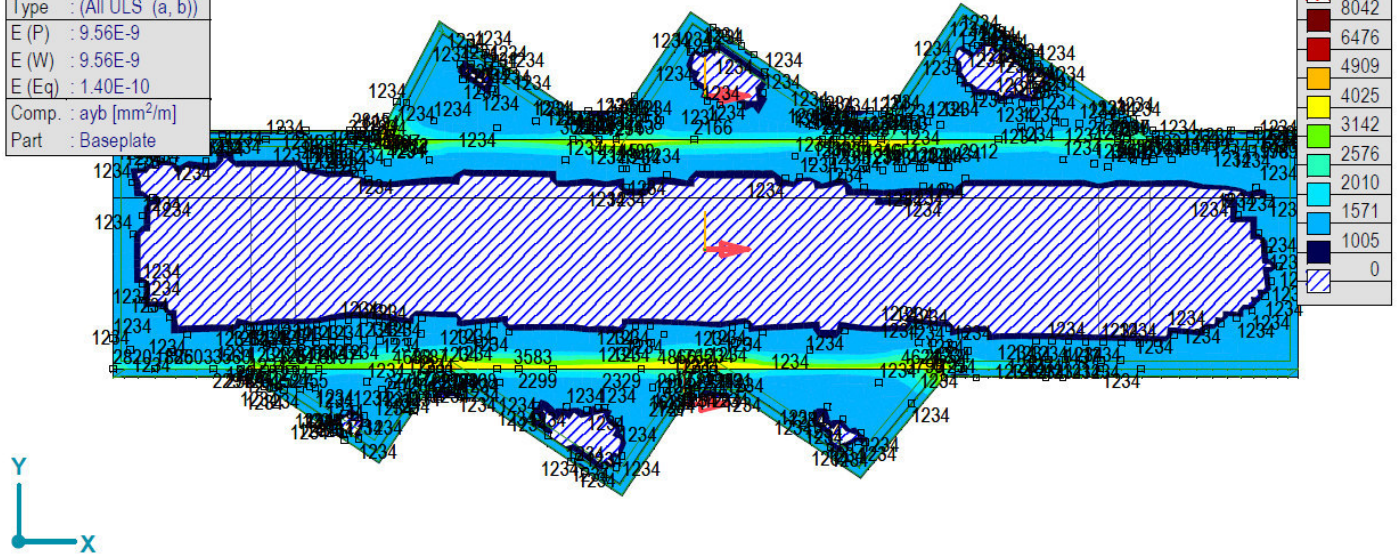
[RI], > Плоча, Линеарно,(Auto) Крит., ayb, Isosurfaces 2D, Горњи поглед
