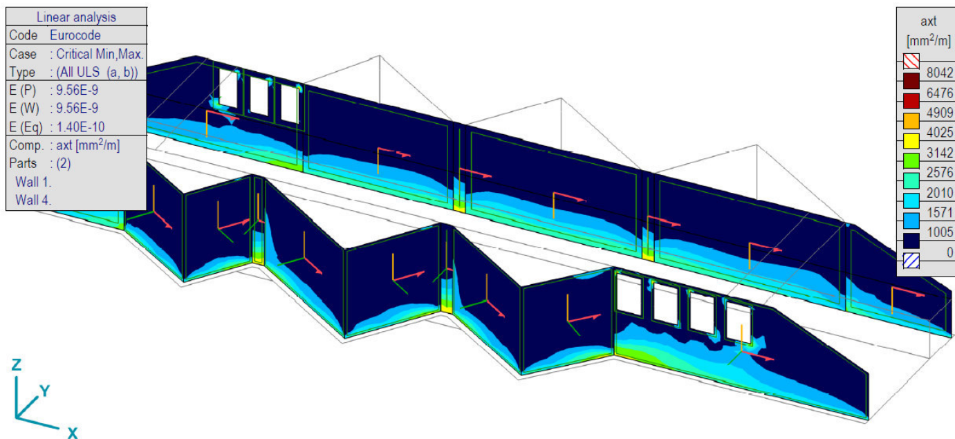
Кол. арм. - [RI], > 2 parts, Линеарно, (Auto) Крм., axt, Isosurfaces 2D
