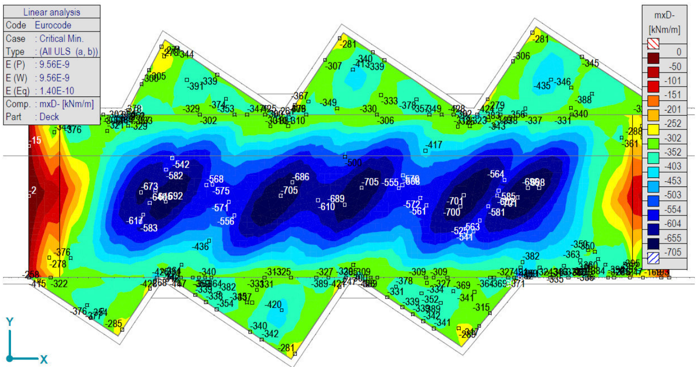
[I], > Палуба, Linear,(Auto) Крит. мин., mxD-, Isosurfaces 2D, Горњи поглед
