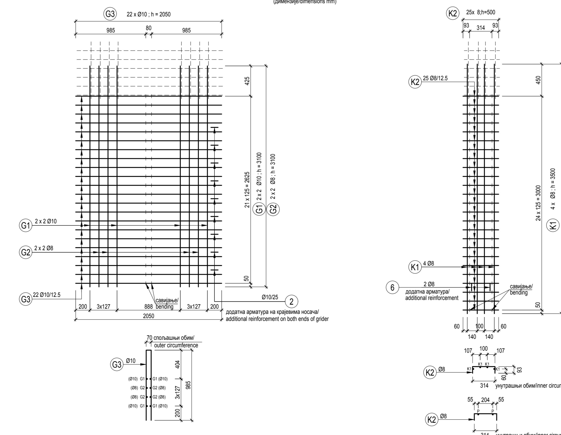
Заварене мреже/welded mesh 1:25 (квалитет/quality: ВНВ 55.50) (димензије/dimensions mm)
