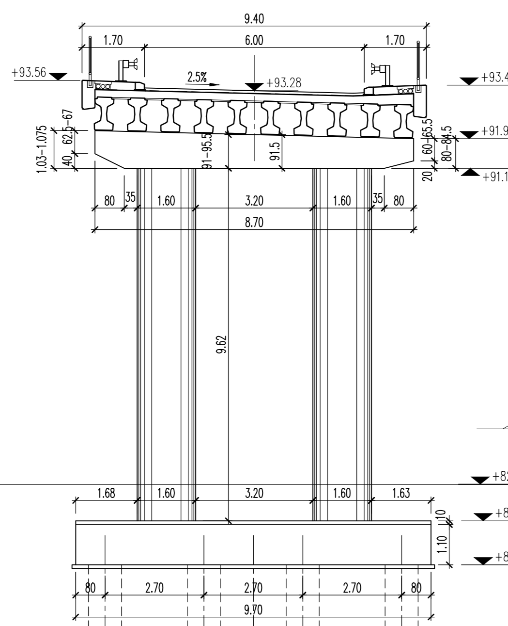
ПОПРЕЧНИ ПРЕСЕК СТУБА С3 CROSS SECTION С3 km 0+238.45 1:100
