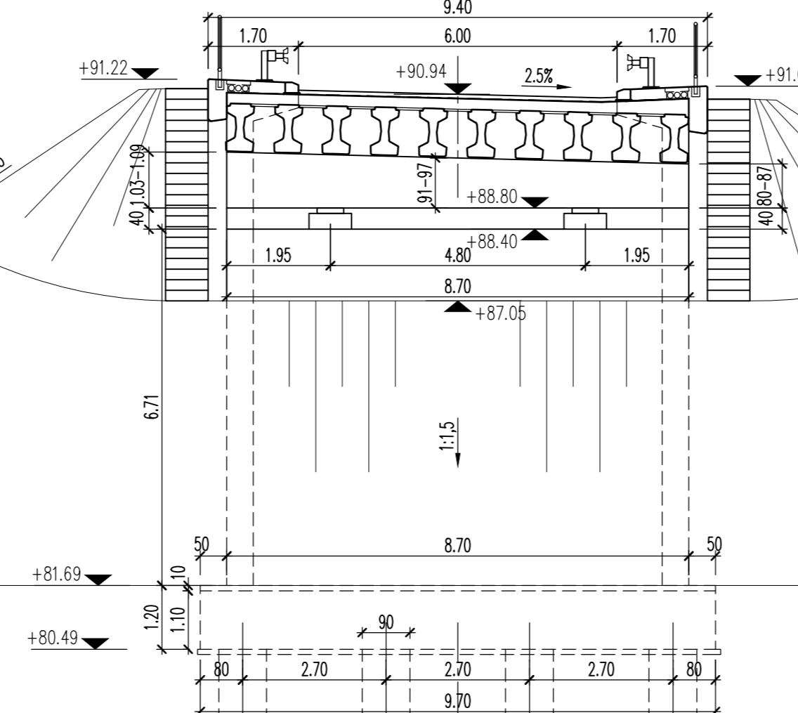
ПОПРЕЧНИ ПРЕСЕК СТУБА С6 CROSS SECTION С6 km 0+303.95 1:100
