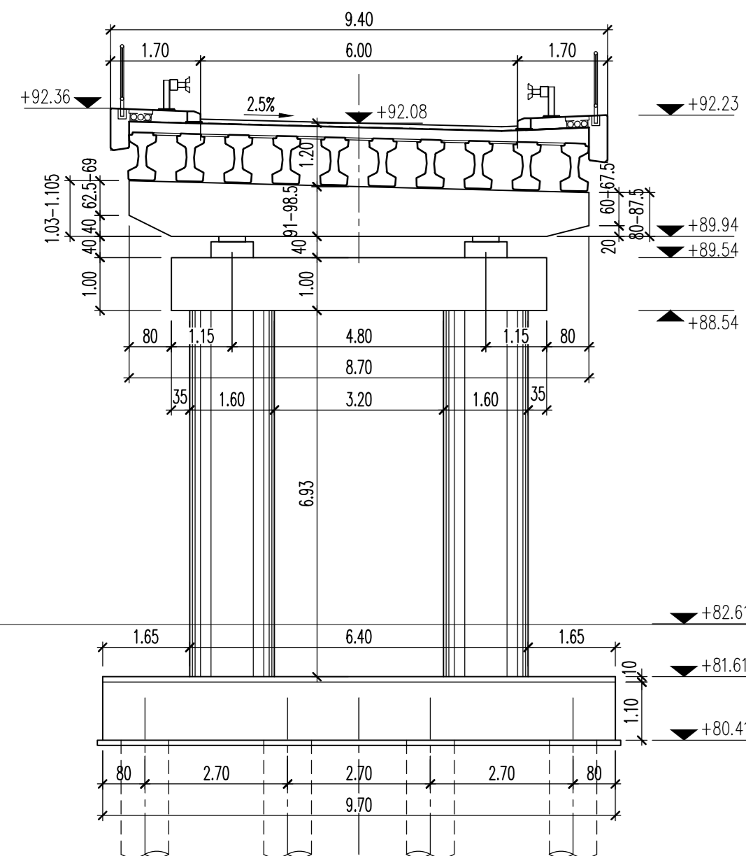
ПОПРЕЧНИ ПРЕСЕК СТУБА С2 CROSS SECTION km 0+215.25 1:100
