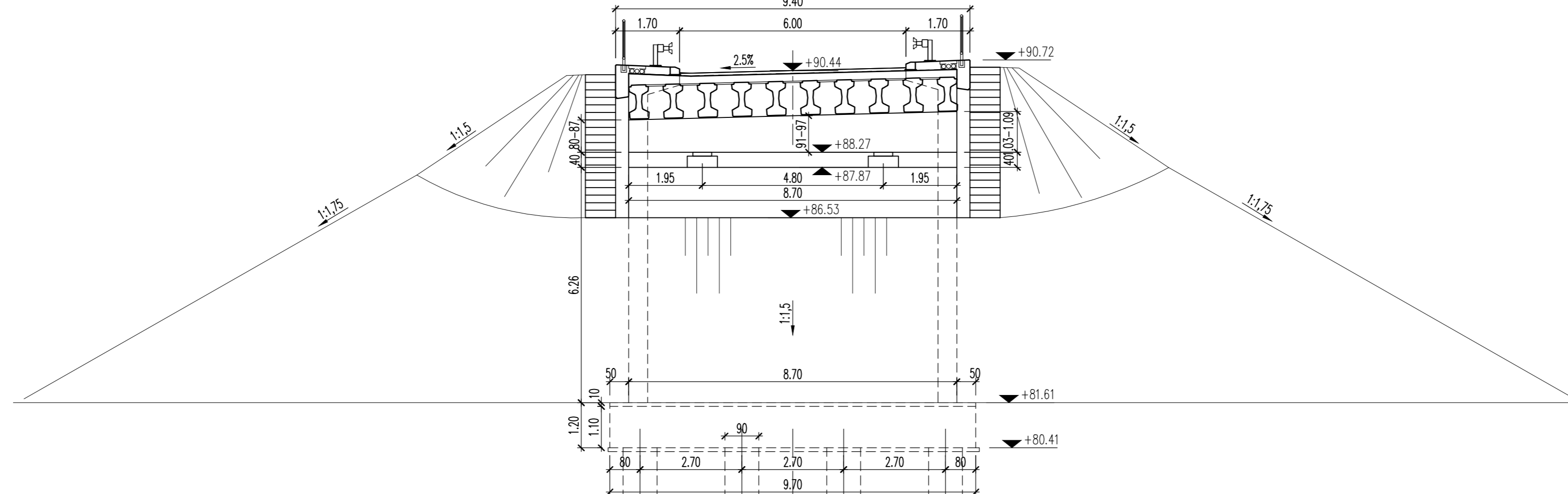
ПОПРЕЧНИ ПРЕСЕК СТУБА С6 CROSS SECTION KM 0+326.09 1:100
