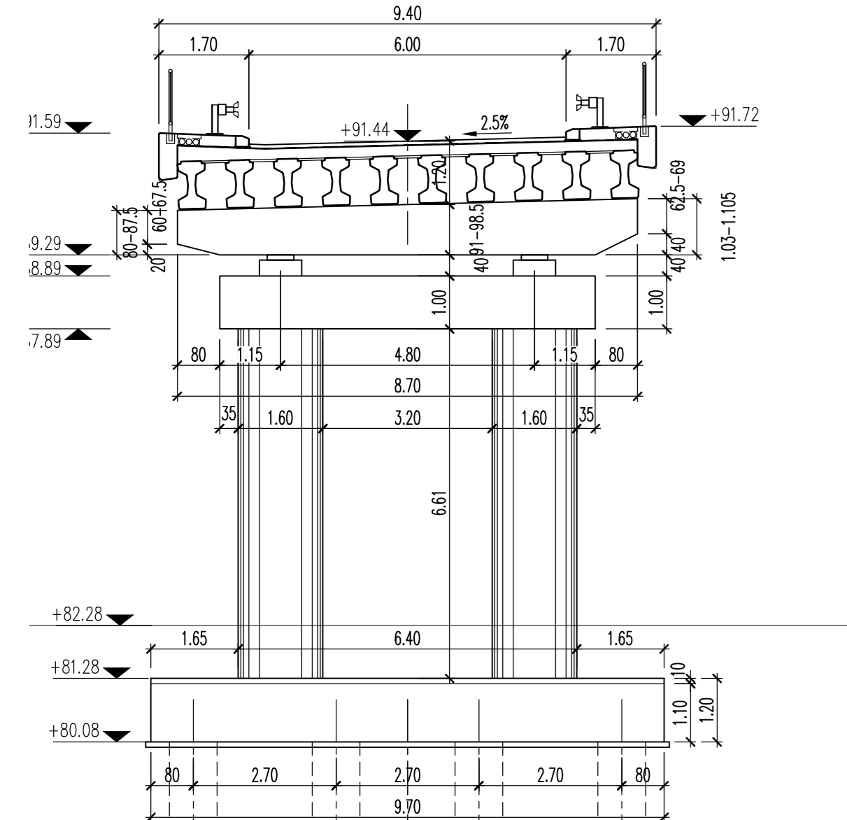
ПОПРЕЧНИ ПРЕСЕК СТУБА С2 CROSS SECTION KM 0+239.39 1:100
