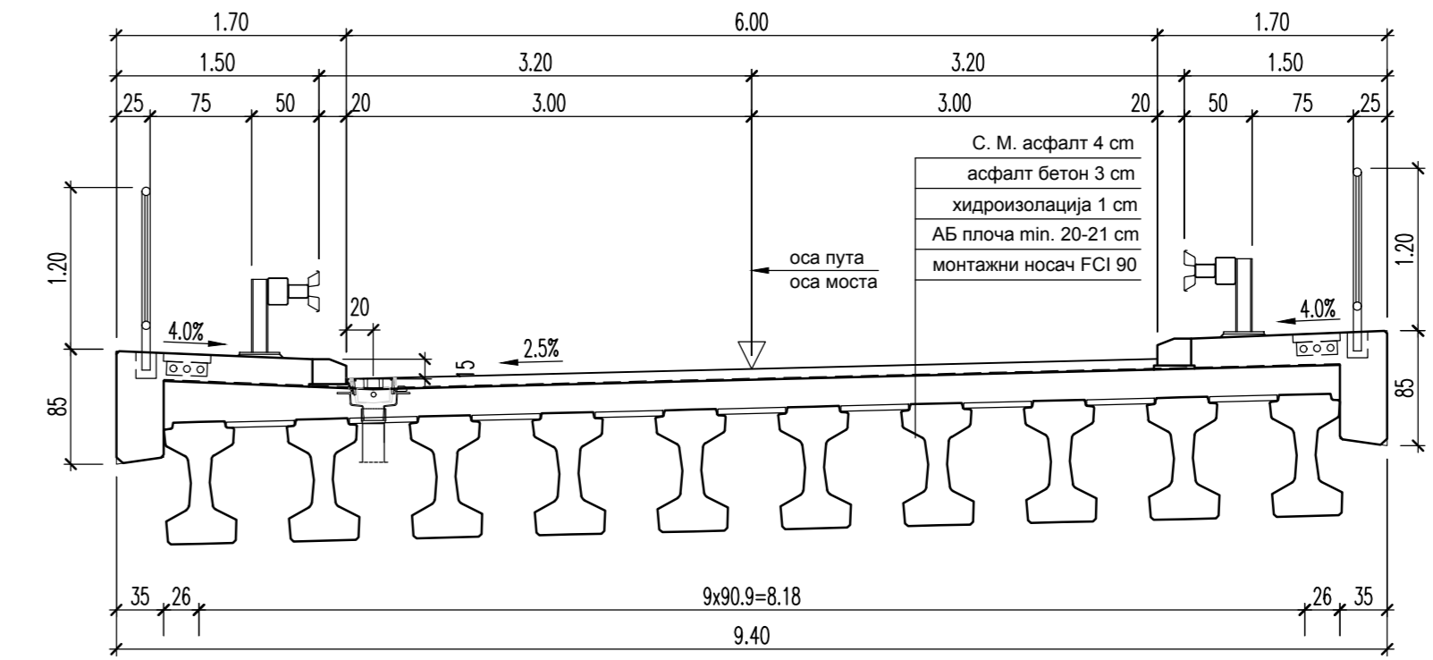
КАРАКТЕРИСТИКЕ МАТЕРИЈАЛА
