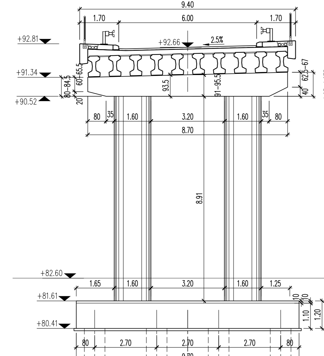
ПОПРЕЧНИ ПРЕСЕК СТУБА С3 CROSS SECTION KM 0+262.59 1:100
