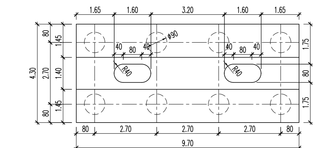
OSNOVNA ТЕЛО С3 BASE 1:100
