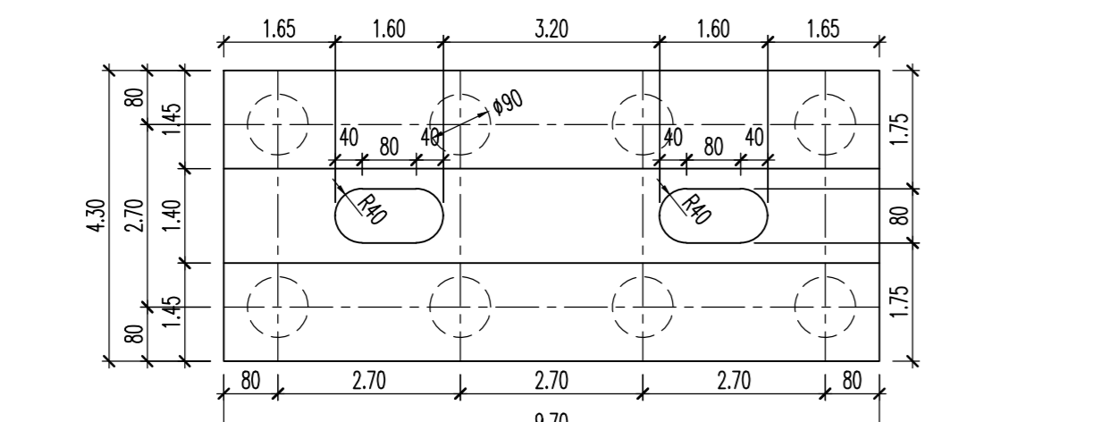
OSNOVNA ТЕЛО С3 BASE 1:100
