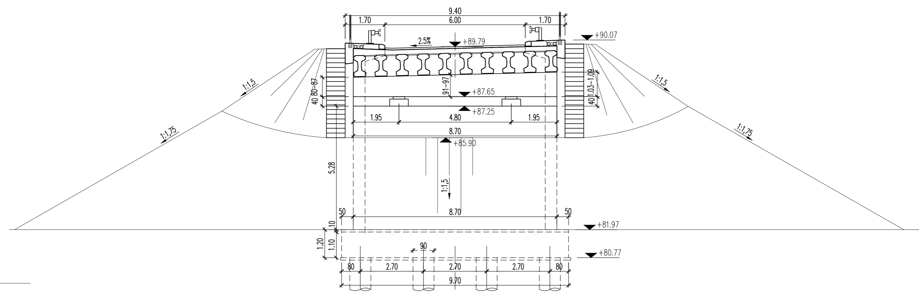
ОСНОВНО ТЕЛО С6 ABUTMENT 1:100
