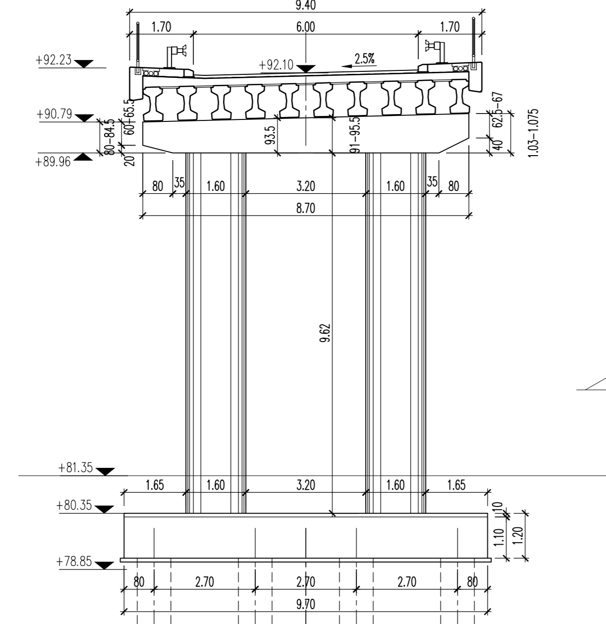
OSNOVNA ТЕЛО С3 BASE 1:100
