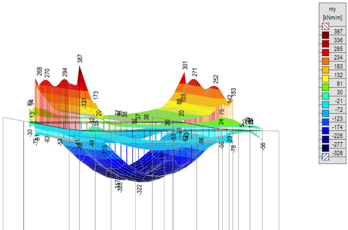
[[], > Палуба, Линеарно,(Auto) Крит., my, Isosurfaces 3D
