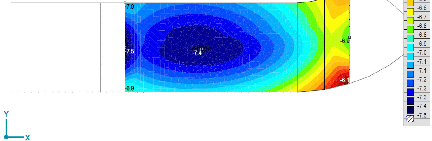
[I], > Палуба, Линеарно, (SLS Quasipermanent) Крит. мин., eZ, Isosurfaces 2D, Горњи поглед
