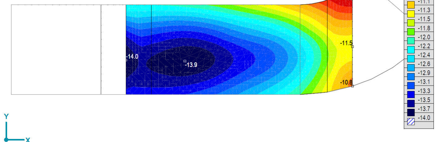
[I], > Палуба, Линеарно, (SLS Characteristic) Крит. мин., eZ, Isosurfaces 2D, Горњи поглед
