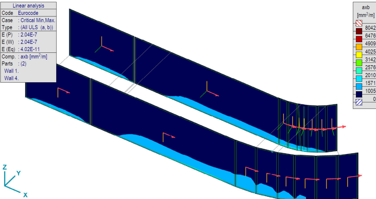
Кол. арм. - [R], > 2 дела, Линеарно, (Auto) Крм., axb, Isosurfaces 2D
