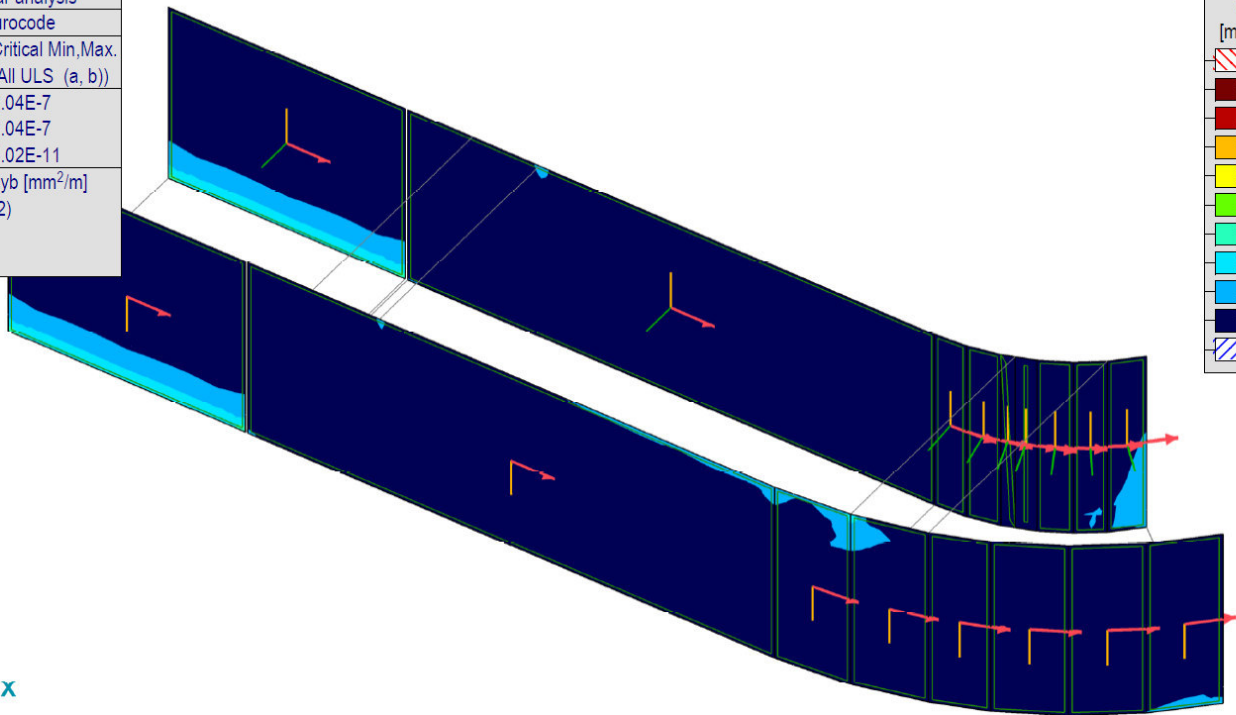
Кол. арм.- [R], > 2 parts, Линеарно,(Auto) Крив., ayb, Isosurfaces 2D
