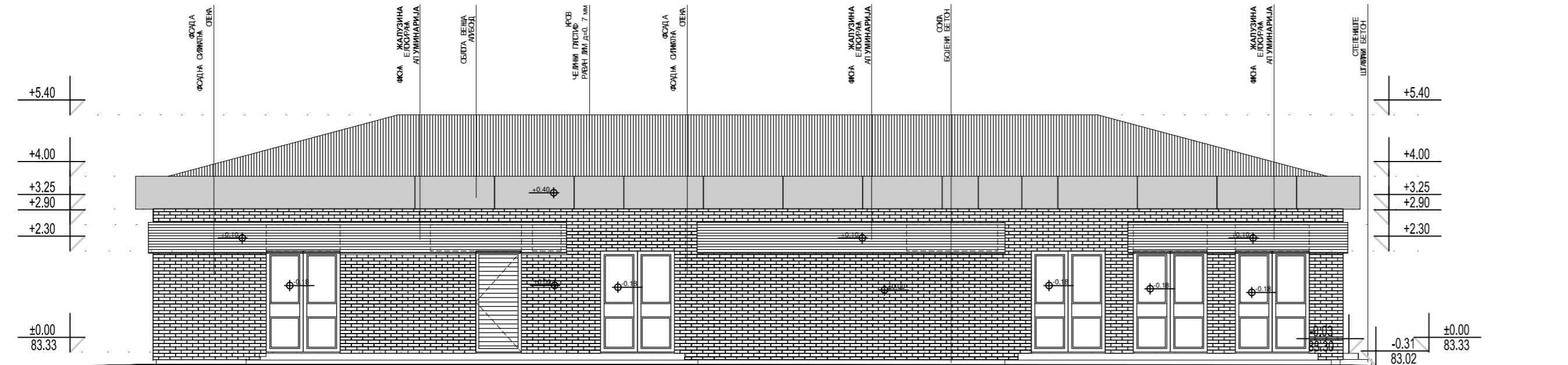
Ђ Д Г В Б А СЕВЕРОИСТОЧНИ ИЗГЛЕД
