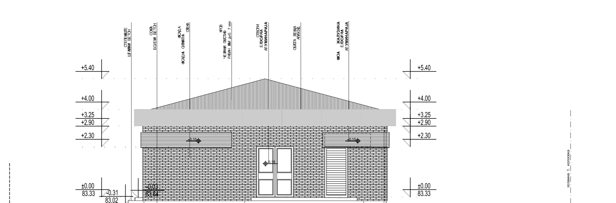
4 3 2 1 ЈУГОИСТОЧНИ ИЗГЛЕД
