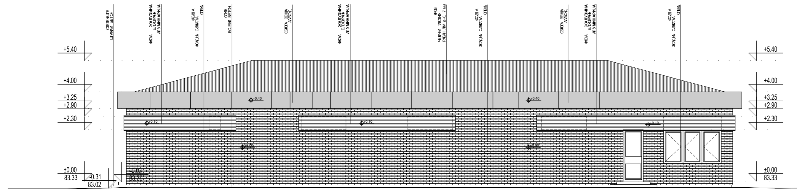
А Б В Г Д Ђ ЈУГОЗАПАДНИ ИЗГЛЕД
