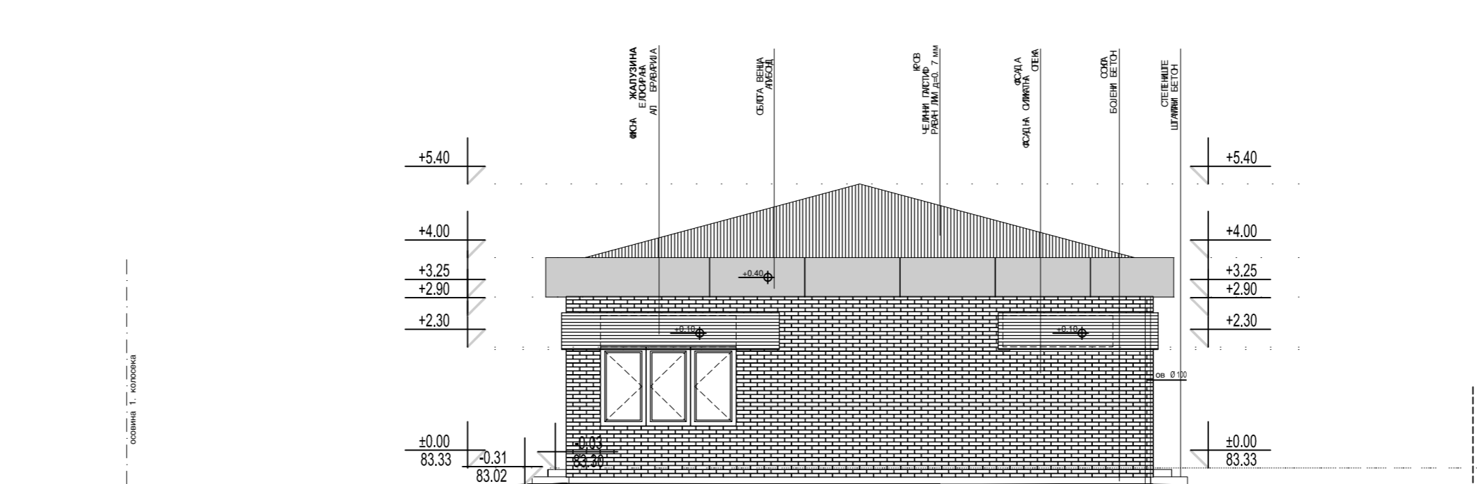
1 2 3 4 СЕВЕРОЗАПАДНИ ИЗГЛЕД
