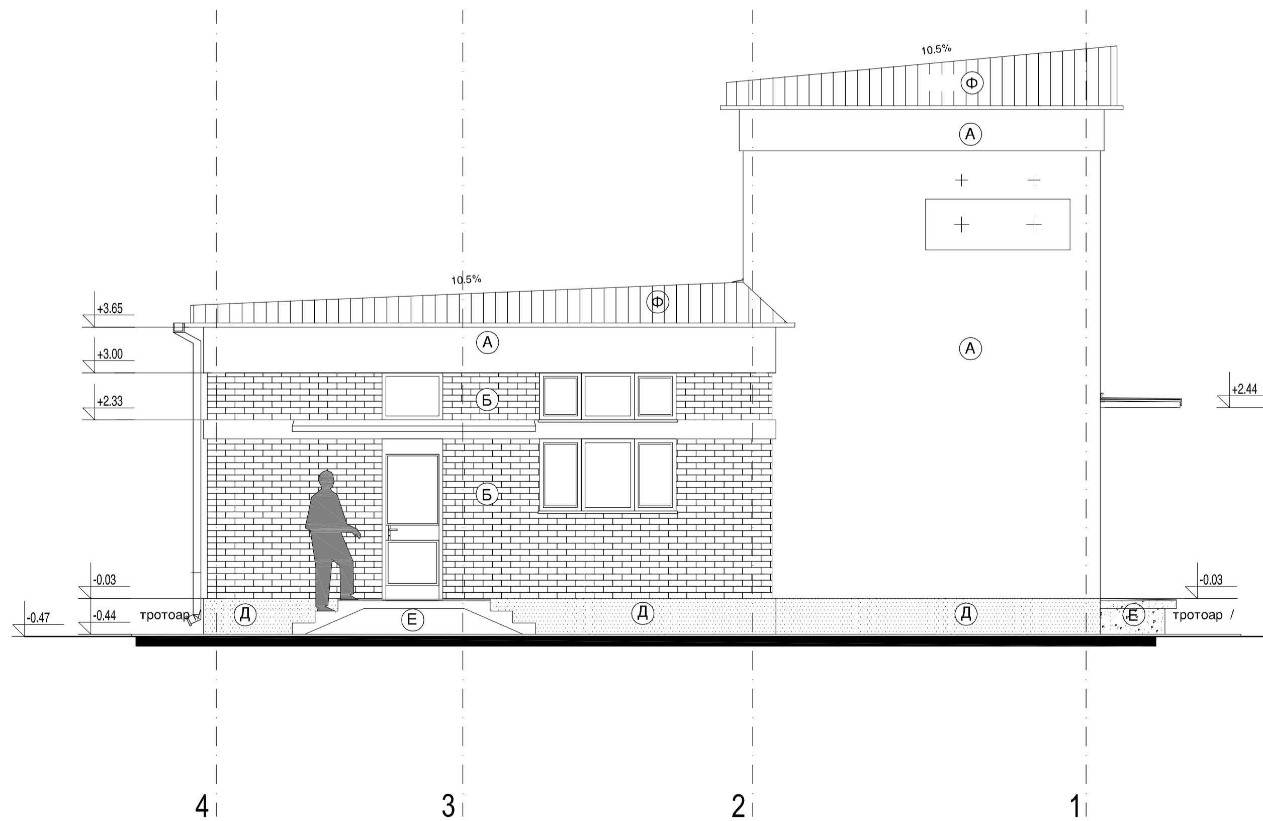
ИЗГЛЕД III
