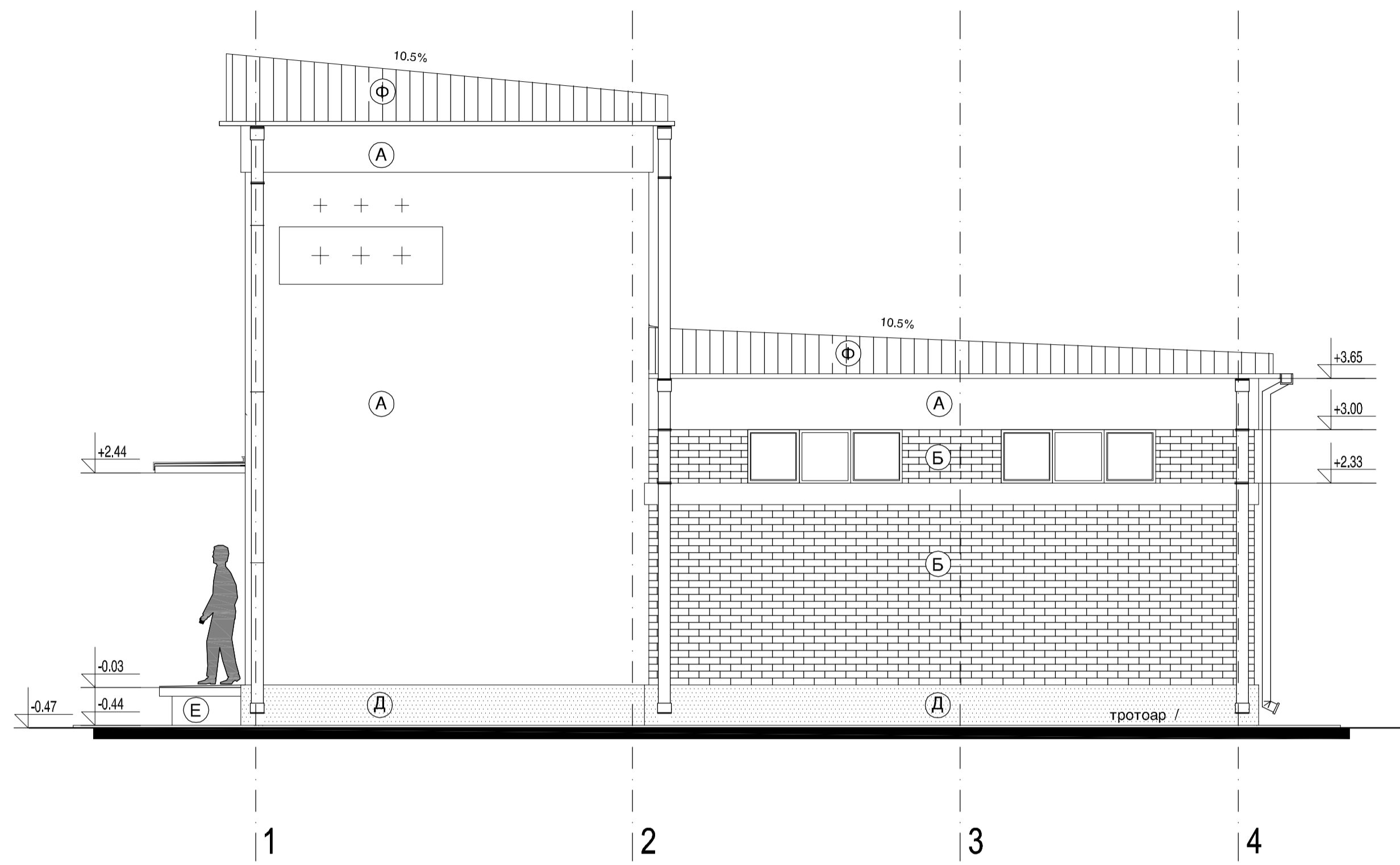
ИЗГЛЕД III
