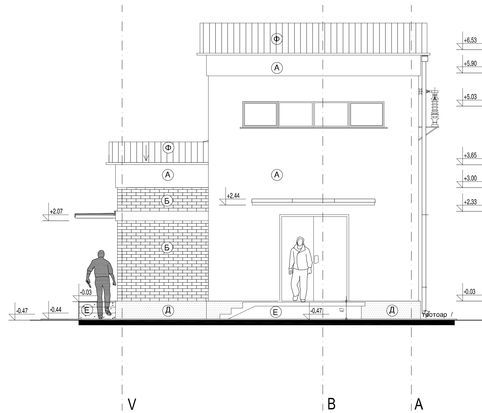
ИЗГЛЕД IV
