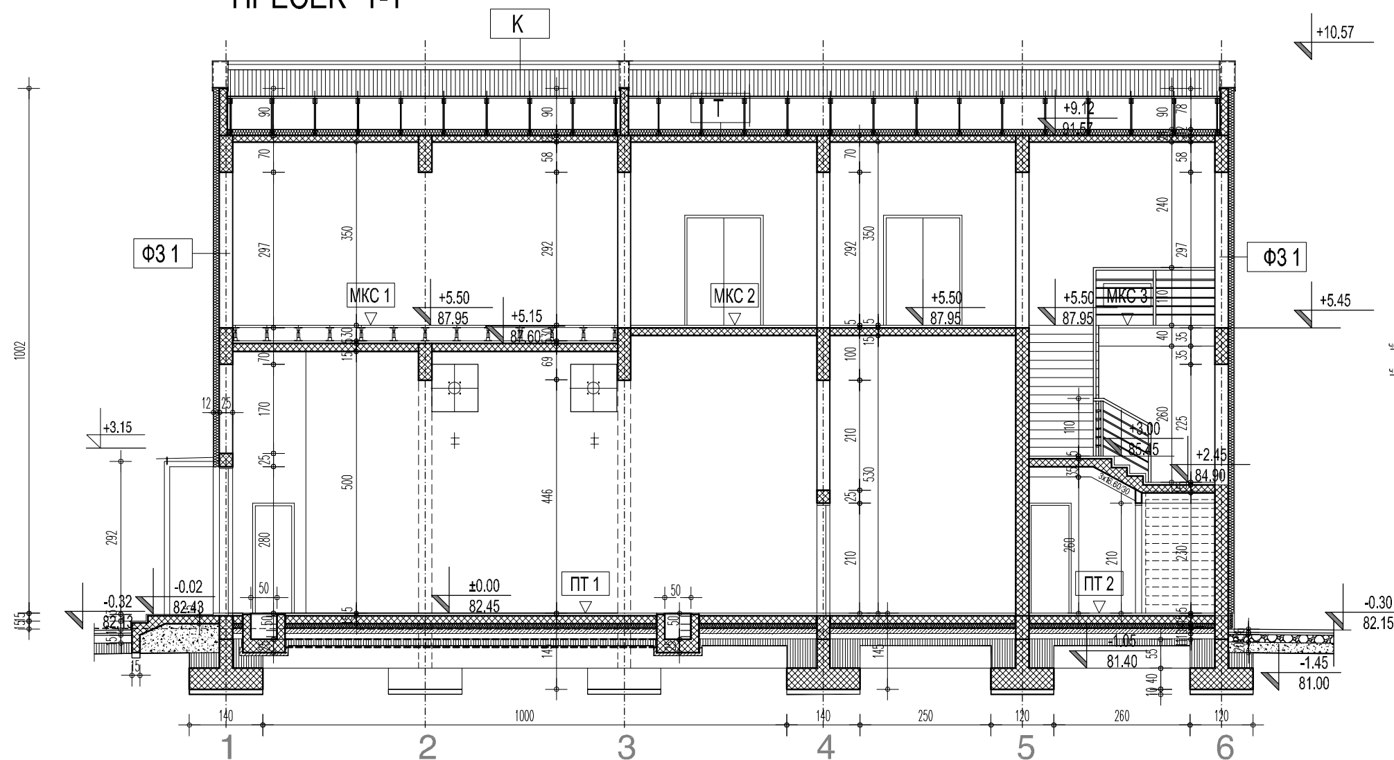
ПРЕСЕК 1-1
