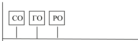
Слика 5. Циклуси редовних оправки парних локомотива узаног колосека
