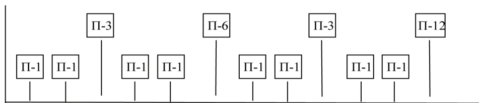
Слика 2. Циклуси периодичних прегледа дизел локомотива узаног колосека
