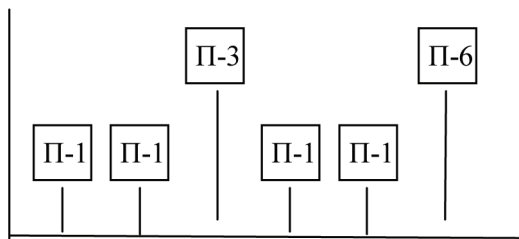
Слика 1. Циклуси периодичних прегледа парних локомотива узаног колосека
