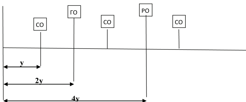
Слика 6. Циклуси редовних оправки дизел локомотива узаног колосека
