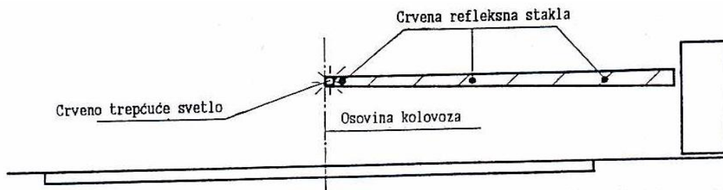
Слика 3. Распоред светлосних знакова на мотки браника ( полубраника) типа L=3,5m и L= 4.5m
