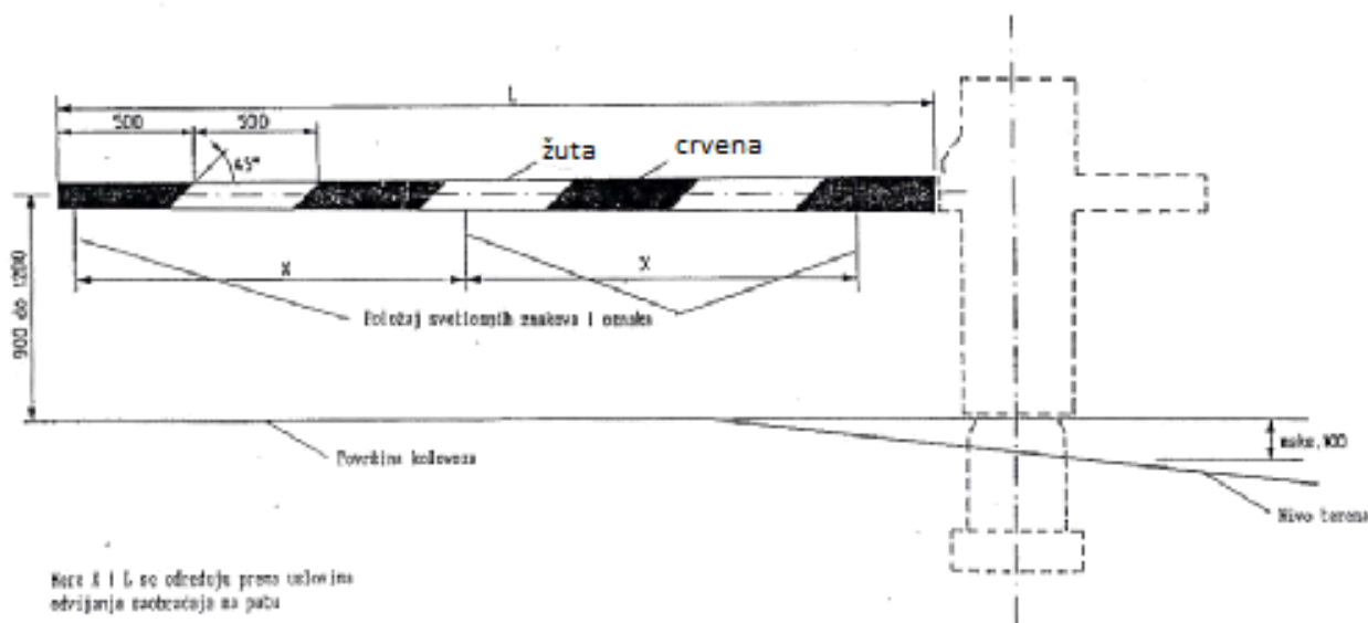
Слика 1 - Шематски приказ браника (полубраника)
