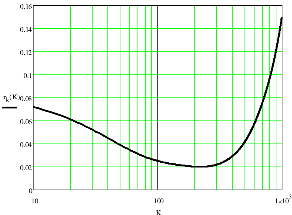
Слика 1 Дијаграм редукионог фактора кабла STKA и STA
