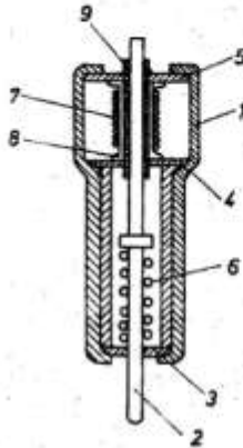
Sl. 3.27. Термички осигурач
