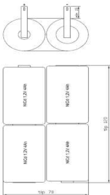
Слика 1: Изглед батеријског паковања 2,4V/ 8Ah
