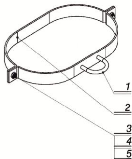
Слика 4 – Обујмица за вођење тегова УАЗ
