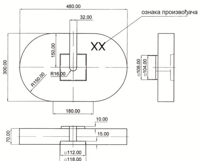
Слика 2 – Бетонски тег од 30 kg
