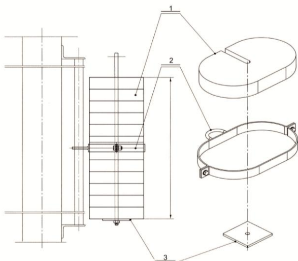
Слика 1 - Слот тегова од 25 kg
