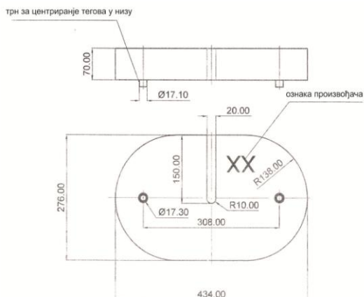
Слика 3 – Бетонски тег УАЗ 25 kg
