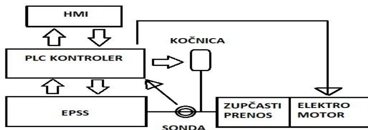
Слика 2. Блок шема дијагностичког уређаја ЕПСС
